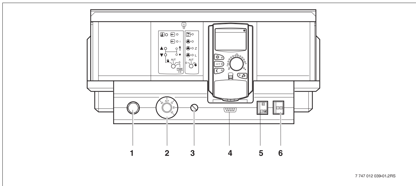
Obr. 4 Ovládací prvky regulačního přístroje Logamatic 4211 (stav při expedici)
