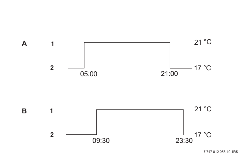
Obr. 20 Nový vytápěcí program
