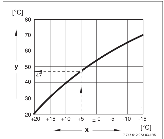
Obr. 3 Topná křivka otopného okruhu (příklad)
