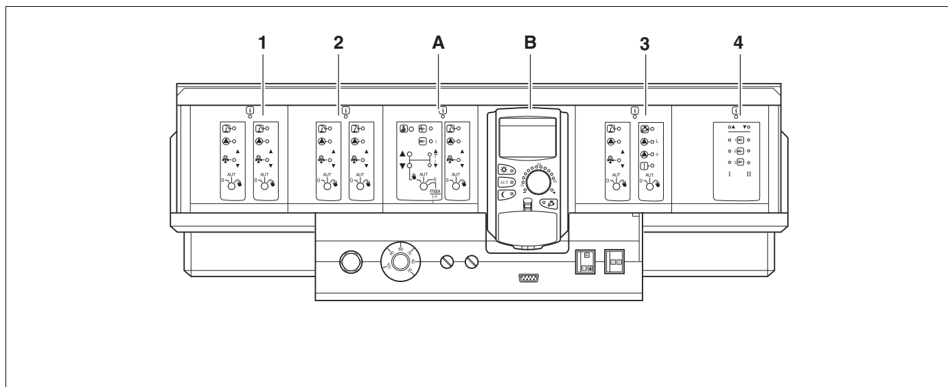
Obr. 5 Osazení moduly
