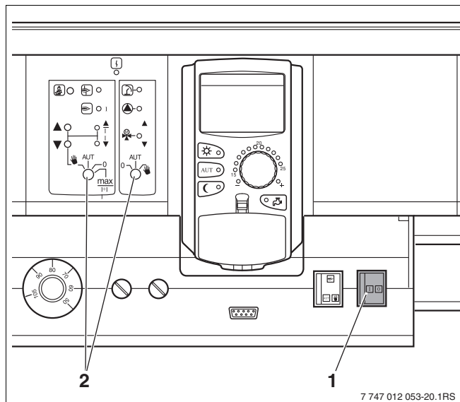
Obr. 8 Provozní spínač
