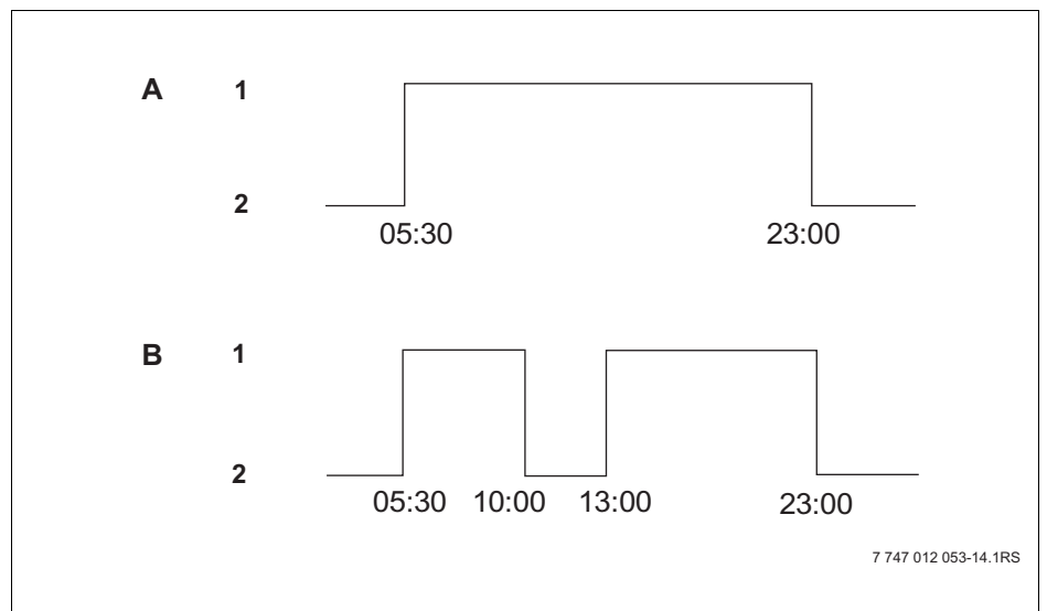
Obr. 16 Vložení spínacích bodů k přerušení fáze vytápění
