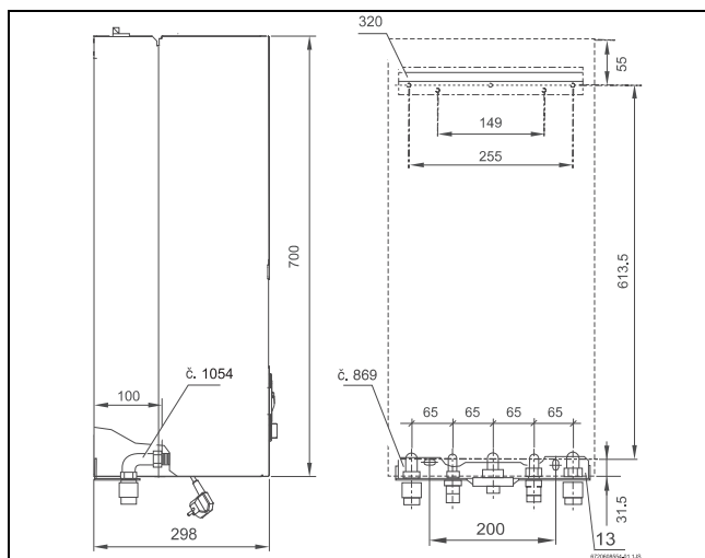
Obr. 8 Montáž s využitím klasické montážní přípojovací lišty (příslušenství č.869 a č.1054)
