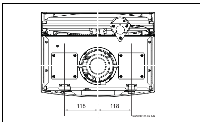
Obr. 2 Pohled shora
