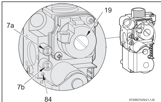
Obr. 31 Plynová armatura
