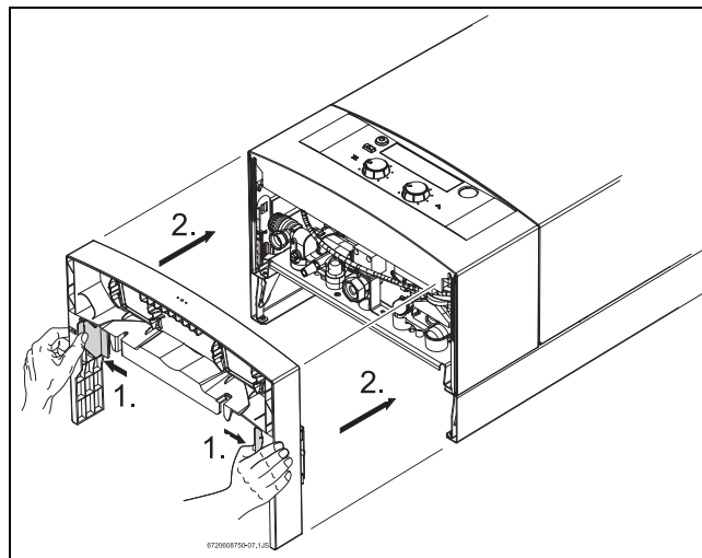
Obr. 17 Umístění podhledového krytu
