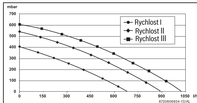
Obr. 5 Charakteristika čerpadla
