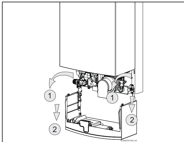
Obr. 12 Servisní poloha pro zpřístupnění rozvodů
