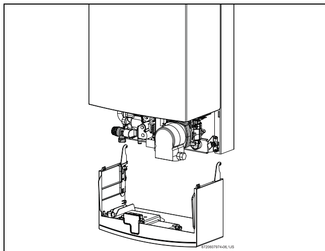
Obr. 13 Sejmutí ovládacího panelu
