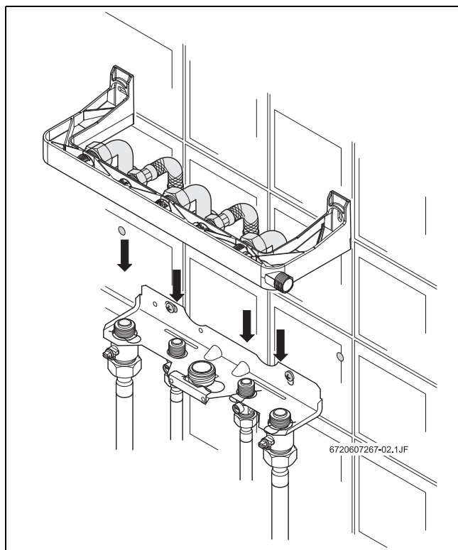
Obr. 9 Propojení kotle (předmontážního rámu č. 1008) s montážní lištou č. 869 pomocí příslušenství č. 1054
