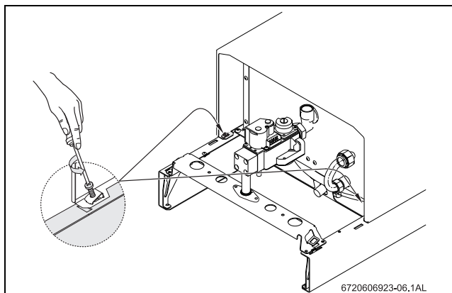
Obr. 14 Odšroubování jisticích šroubů předního krytu
