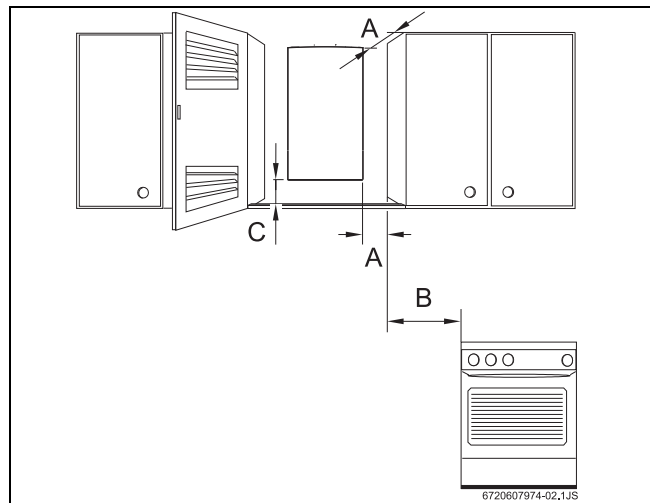
Obr. 6 Minimální odstupy
