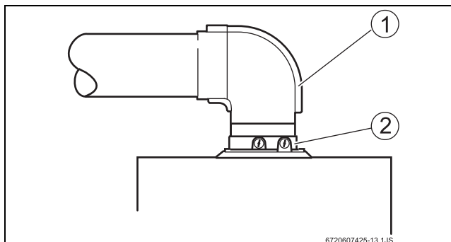
Obr. 15 Upevnění kolena pro odvod spalin pomocí svorek
