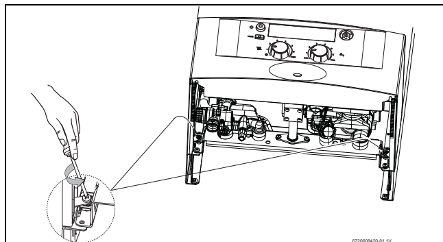
Obr. 11 Pojistné šrouby
