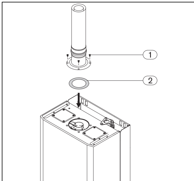
Obr. 16 Montáž omezovací clonky
