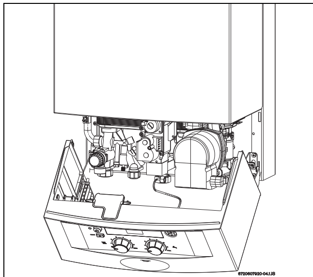
Obr. 30 Servisní poloha pro nastavení plynu
