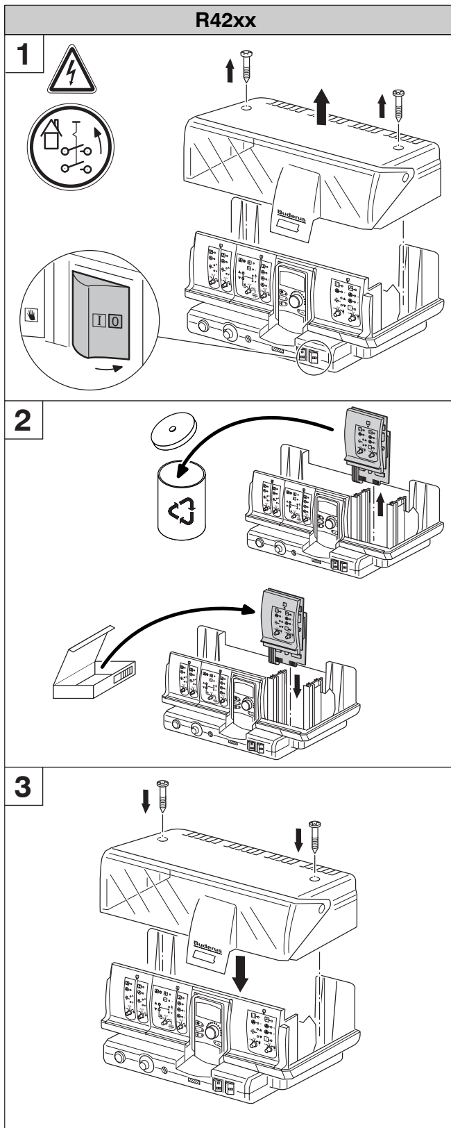
Bild1: Austausch vom Modulen (Logamatic 42xx/43xx)
