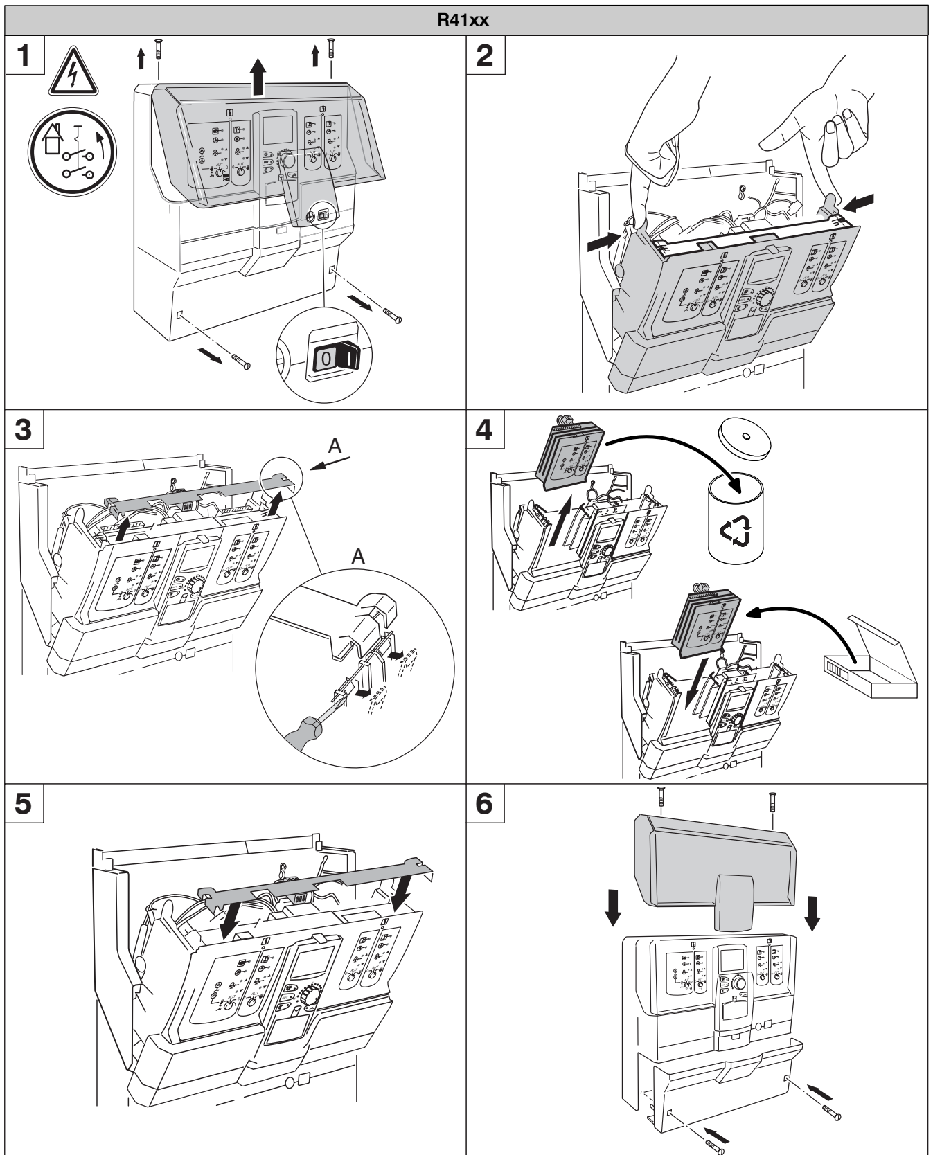
Bild 2: Austausch von Modulen (Logamatic 41xx)
