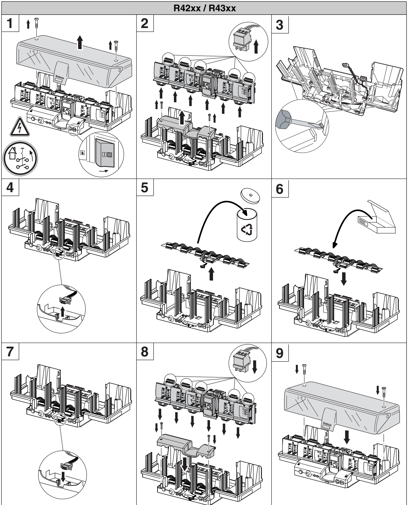
Bild 2: Austausch BM49x bei den Regelgeräten Logamatic 42xx und 43xx
