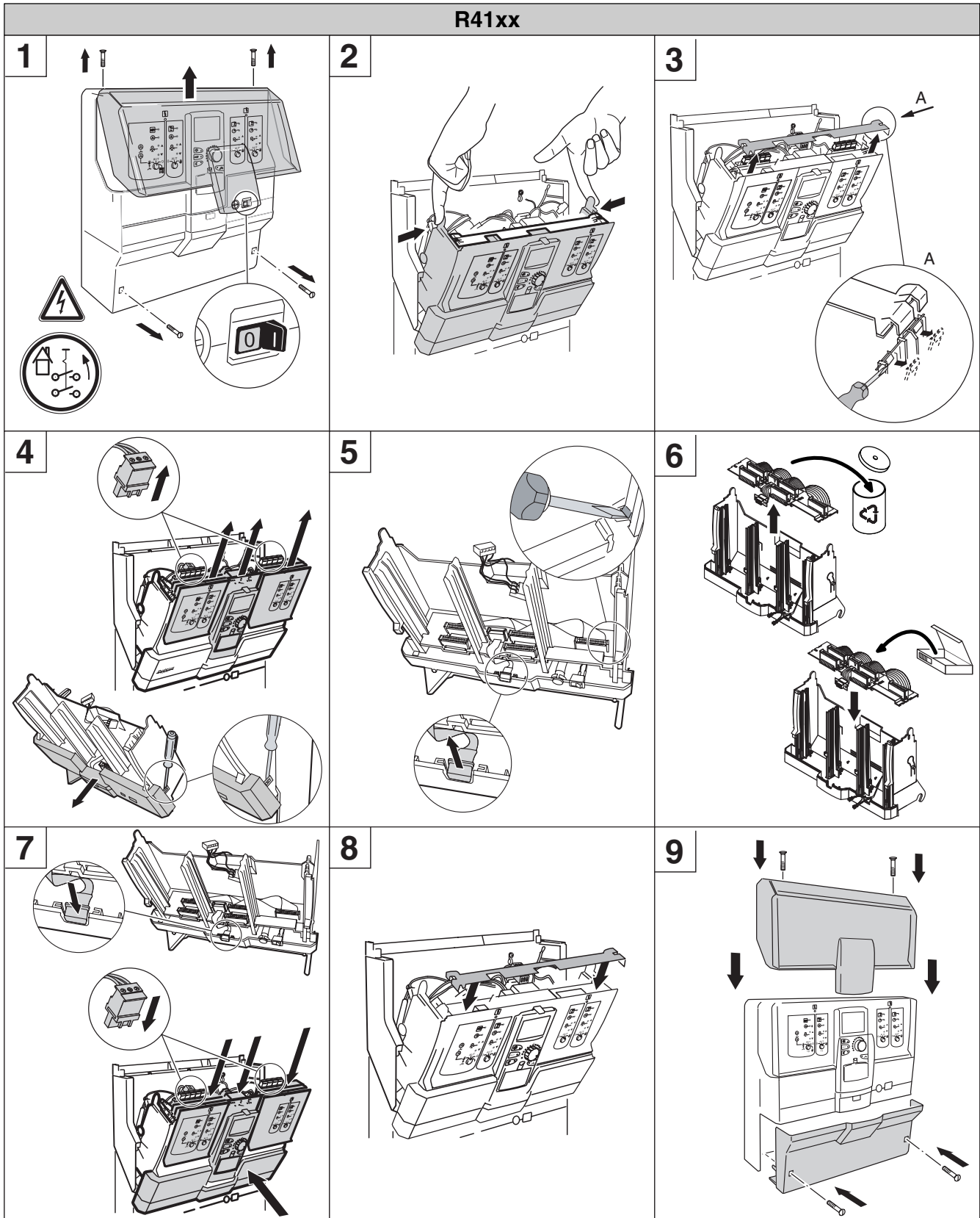
Bild1: Austausch Modul BM49x bei den Regelgeräten Logamatic 41xx
