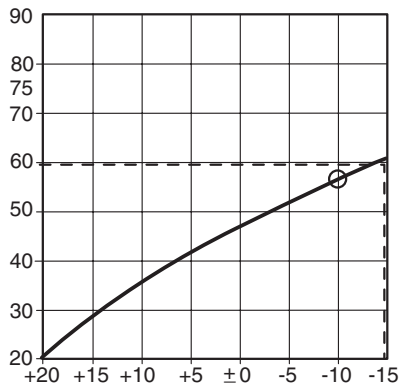
Abb. 7 Heizkennlinie ermitteln
