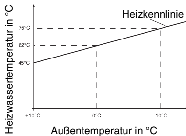
Abb. 9 Heizkennlinientest
