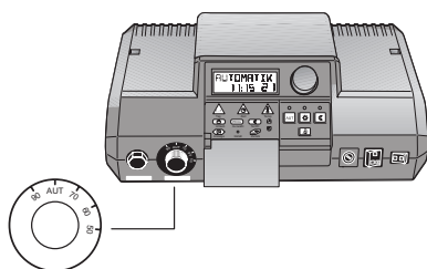
Abb. 2 Reglerknopf abziehen
