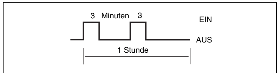
Abb. 8 Darstellung der Zirkulationspumpenlaufzeit mit der Werkseinstellung 2
