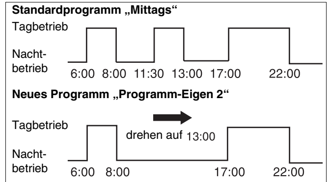
Abb. 8 Löschen einer Heizphase
