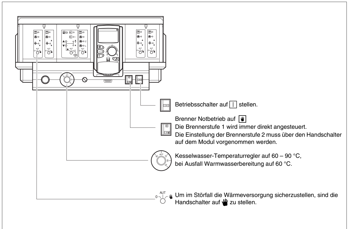
Abb. 13 Heizbetrieb über Handschalter
