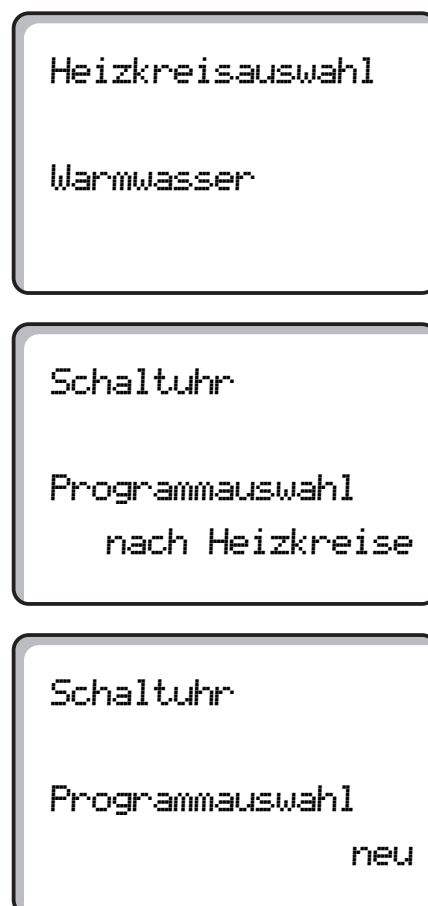
Abb. 10 Neues Warmwasser-Programm eingeben
