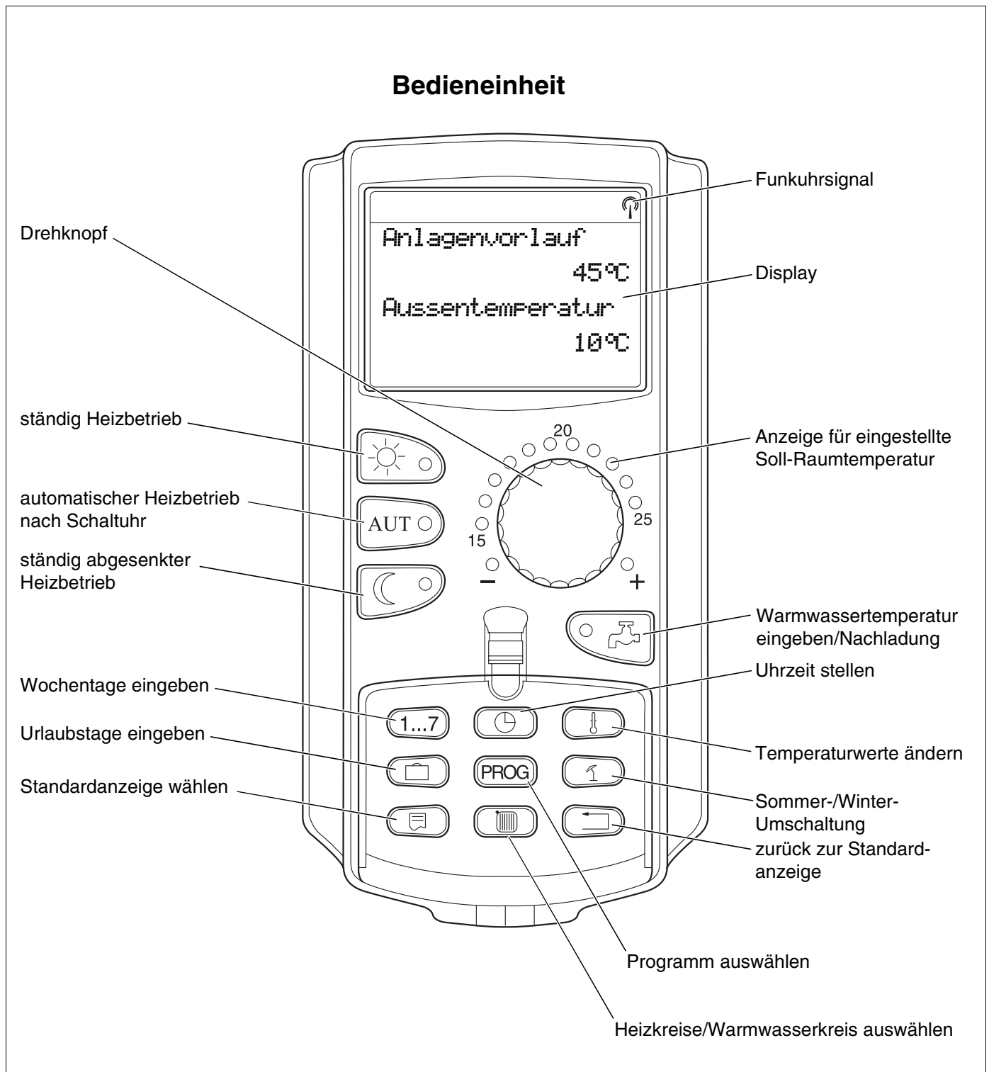
Abb. 5 Bedieneinheit MEC2
