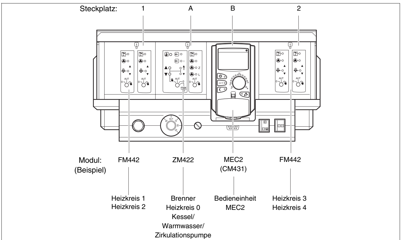
Abb. 2 Modulbestückung
