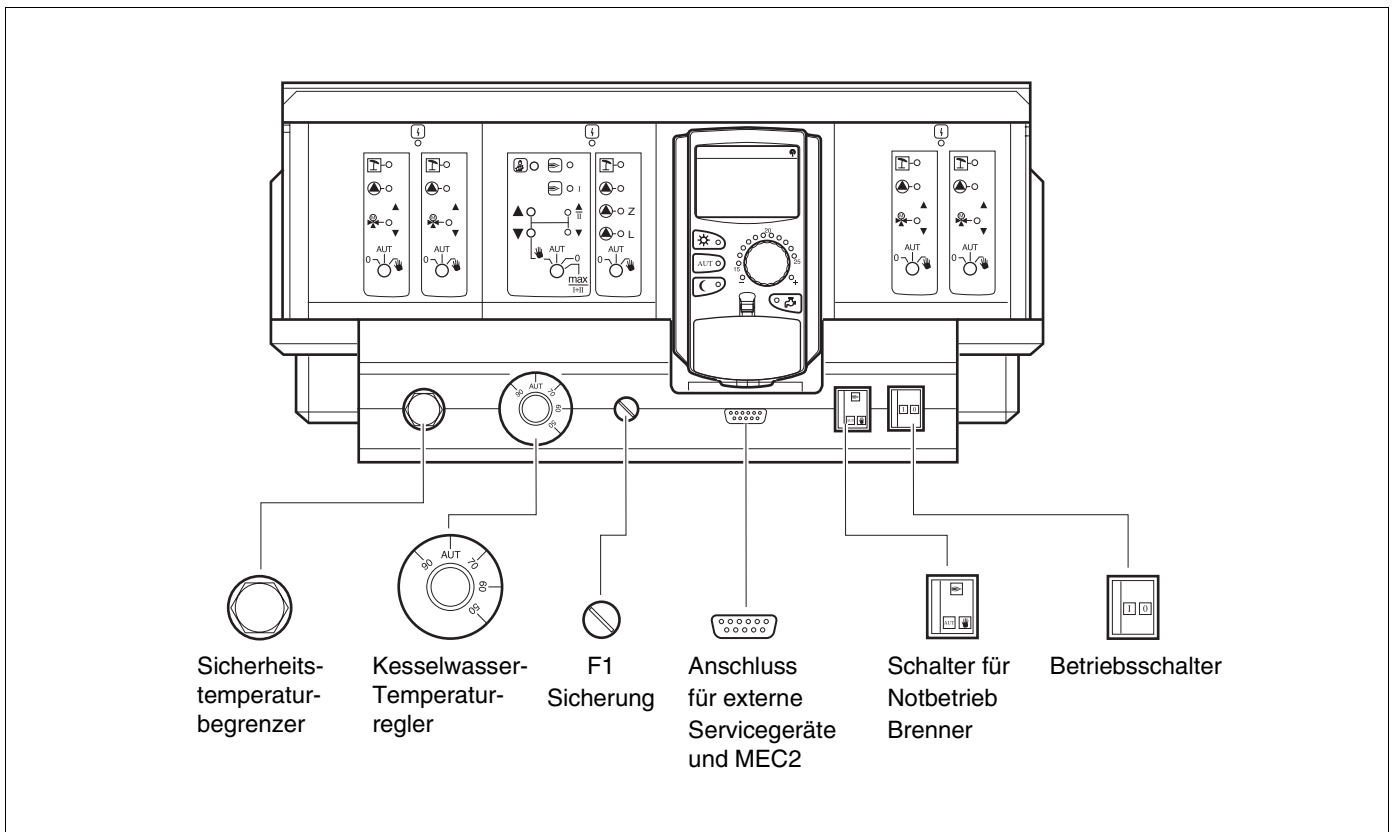
Abb. 1 Bedienelemente
