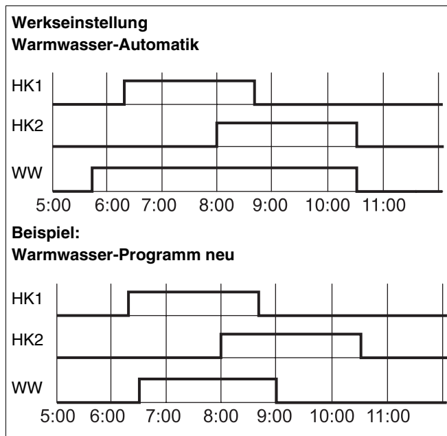
Abb. 10 Neues Warmwasser-Programm eingeben
