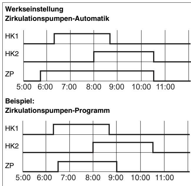
Abb. 11 Neues Zirkulationspumpen-Programm eingeben
