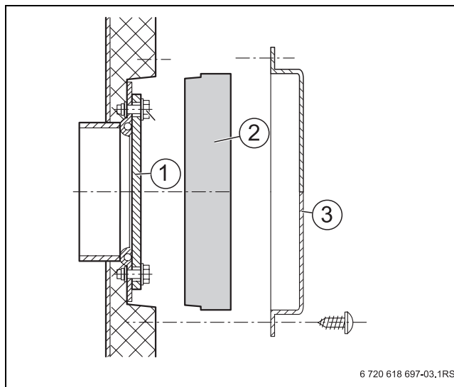
Obr. 10 Tepelná izolace revizního otvoru
