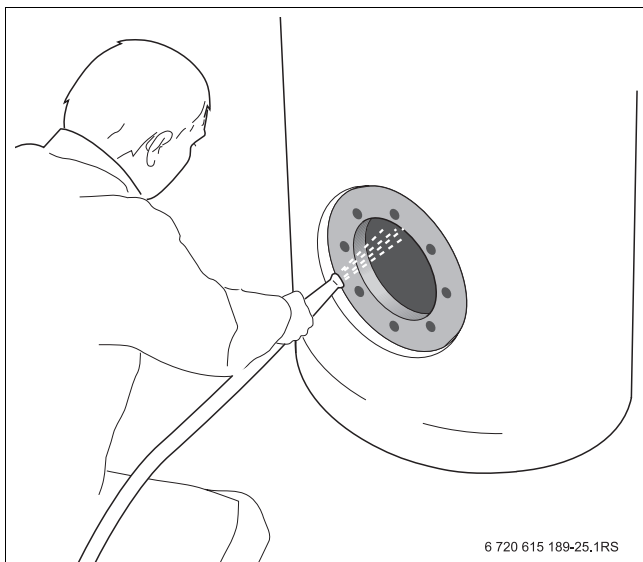
Obr. 12 Vystříkání zásobníku teplé vody
