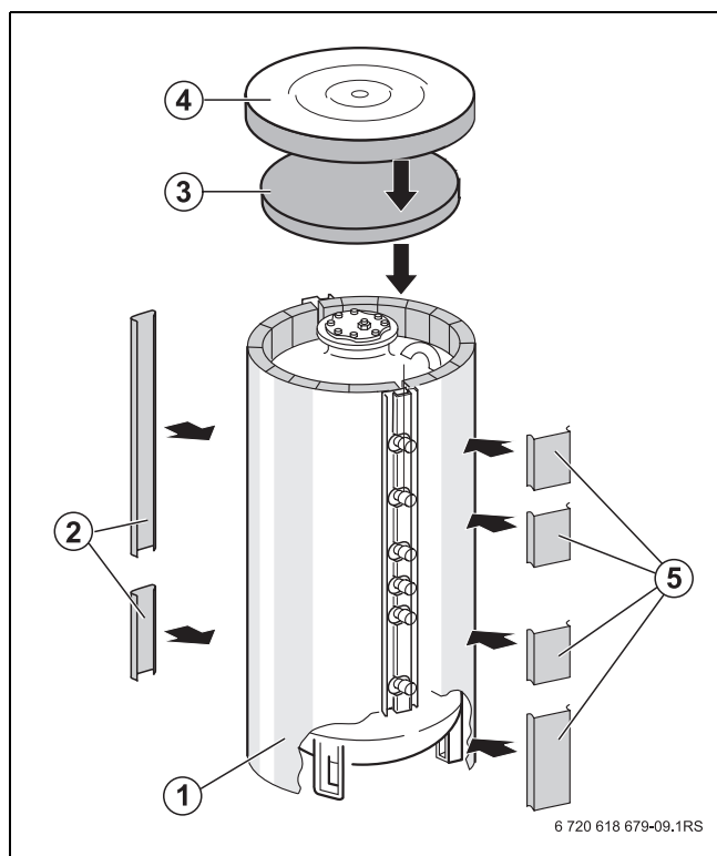
Obr. 9 Montáž krycích lišt a horní tepelné izolace (pohled zezadu)
