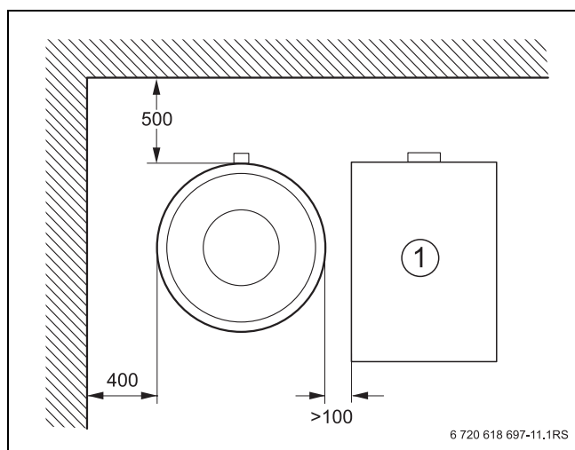
Obr. 4 Minimální míry odstupu od stěn (v mm)
