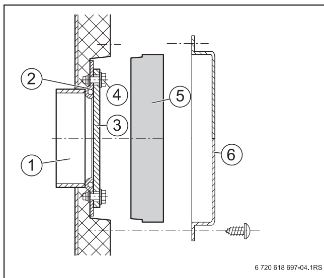
Obr. 14 Montáž víka revizního otvoru
