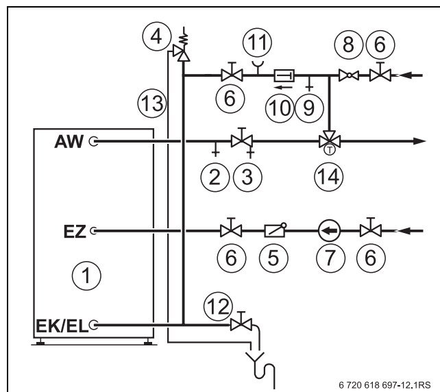
Obr. 5 Instalace (schématické znázornění)
