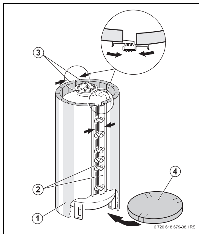
Obr. 8 Montáž tepelné izolace (pohled zezadu)
