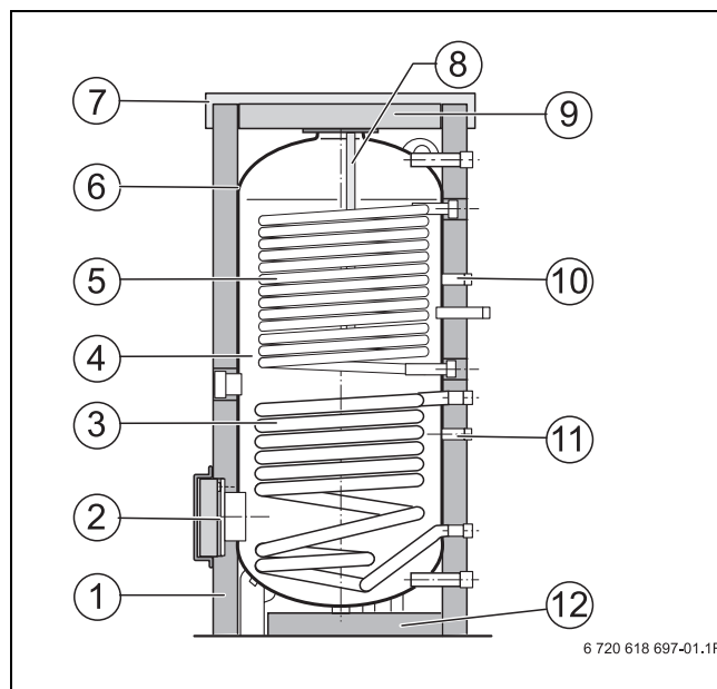
Obr. 1 Zásobník teplé vody Storacell SW400/500-1solar
