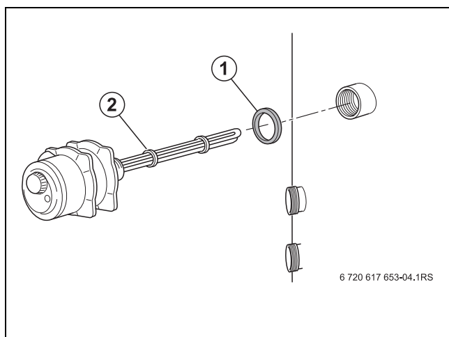
Obr. 7 Montáž elektrické topné vložky
