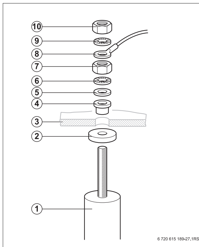
Obr. 13 Výměna hořčkové anody
