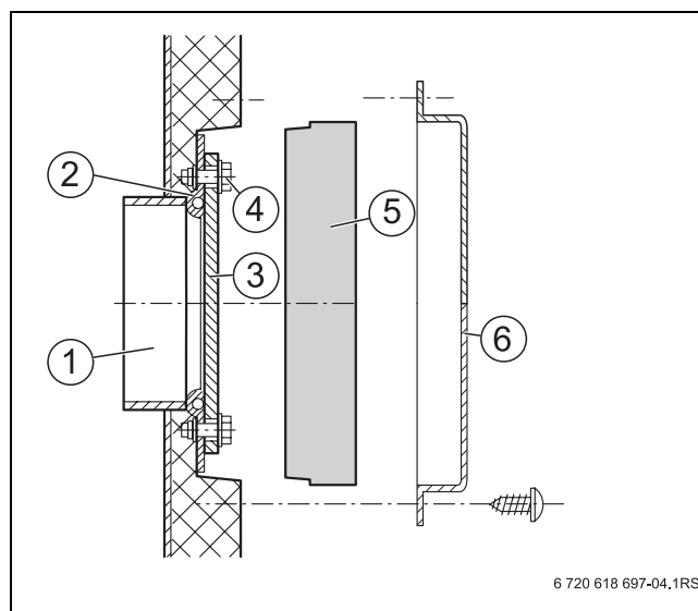
Obr. 11 Demontáž víka revizního otvoru
