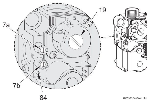
Obr. 4 Plynová armatura
