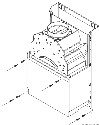
Obr. 1 Ochranný kryt
