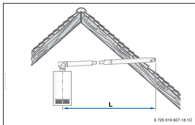
Obr. 17 Montážní varianty se stavební sadou WH/WS
