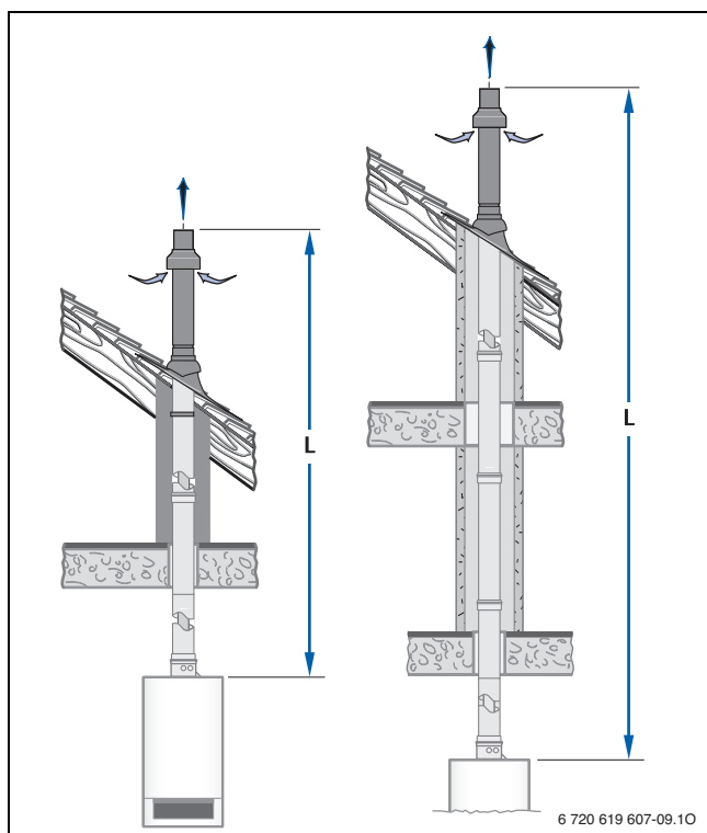
Obr. 16 Montážní varianty se stavební sadou DO
