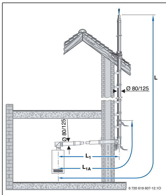
Obr. 20 Montážní varianty se stavební sadou GAF-K
