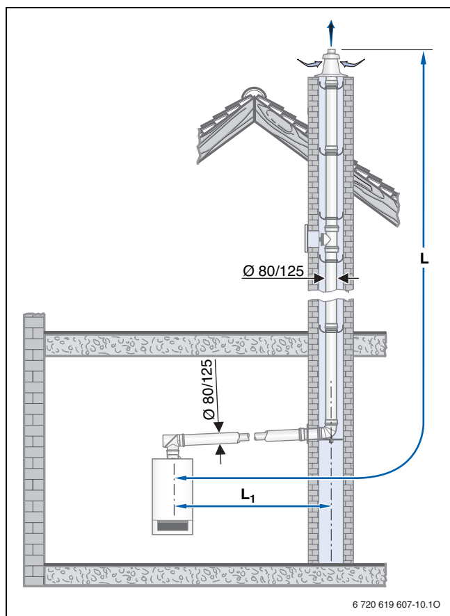
Obr. 18 Montážní varianty se stavební sadou DO-S
