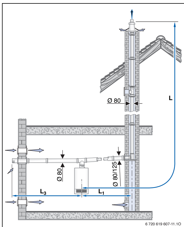
Obr. 19 Montážní varianty se stavební sadou GAL-K + GA-K
