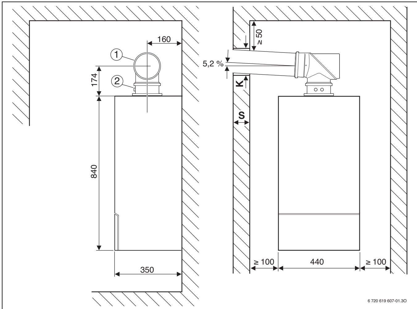
Obr. 8 Vedení spalin \varnothing 80/125 mm nebo \varnothing 80 mm
