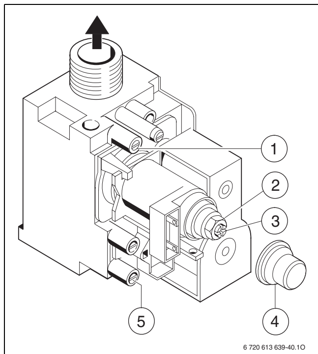
Obr. 43 Plynová armatura
