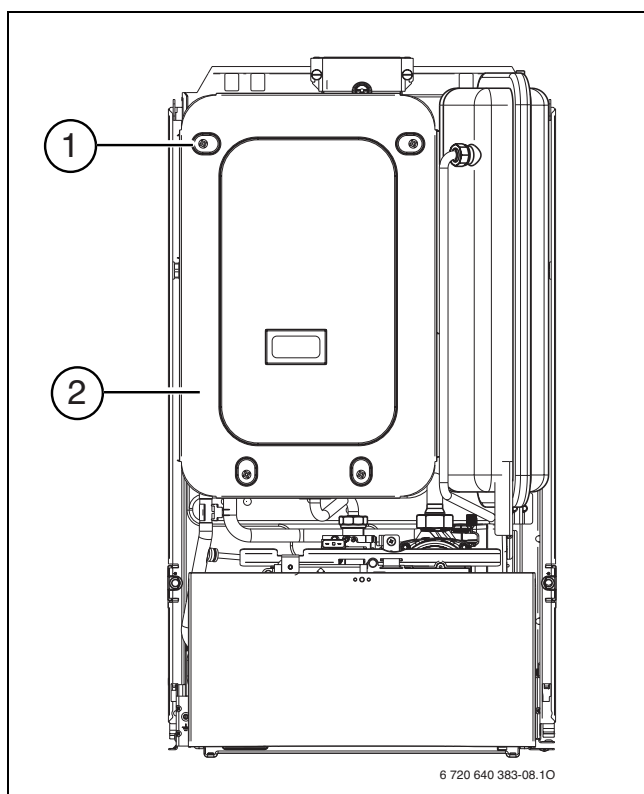
Obr. 53 Otevření vzduchové komory
