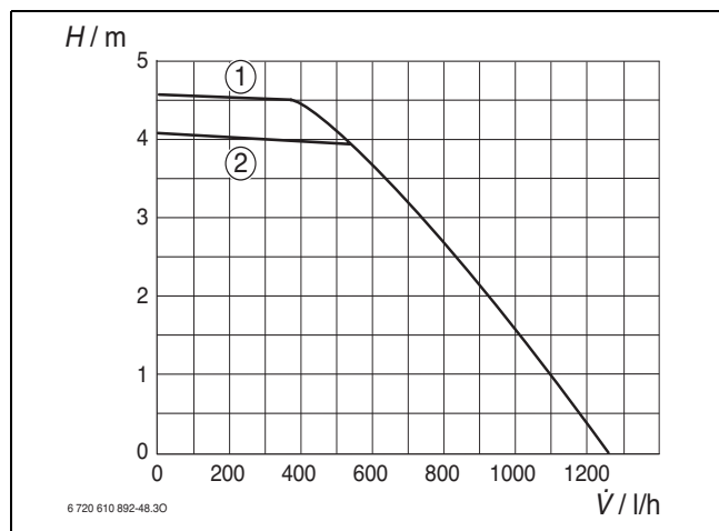
Obr. 39 Konstantní tlak
