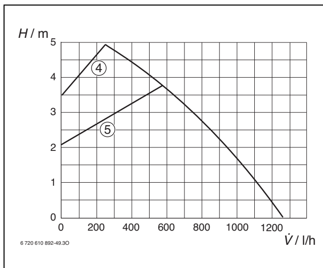
Obr. 40 Proporcionální tlak
