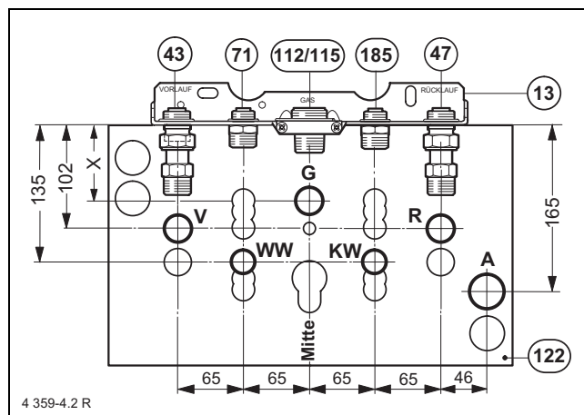
Obr. 8 Připojovací rozměry - instalace pod omítku
