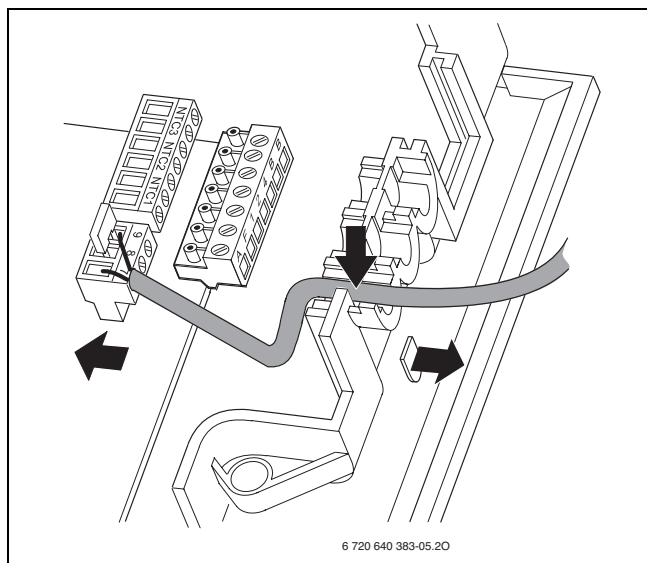
Obr. 22 Připojení termostatu zásobníku
