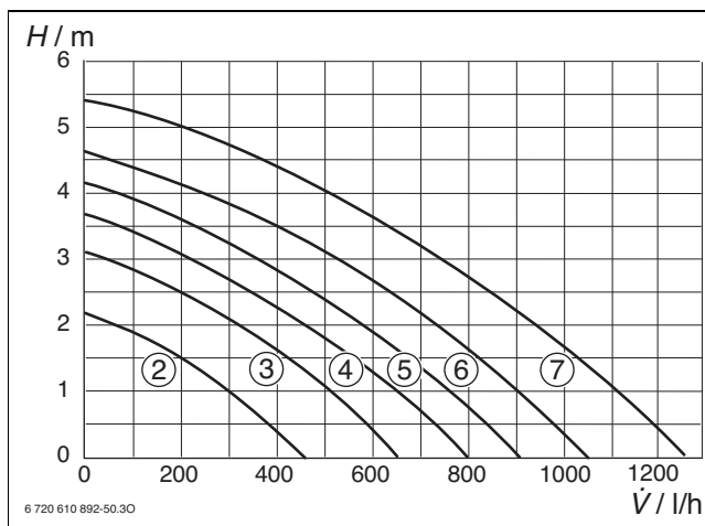
Obr. 41 Charakteristiky čerpadla
