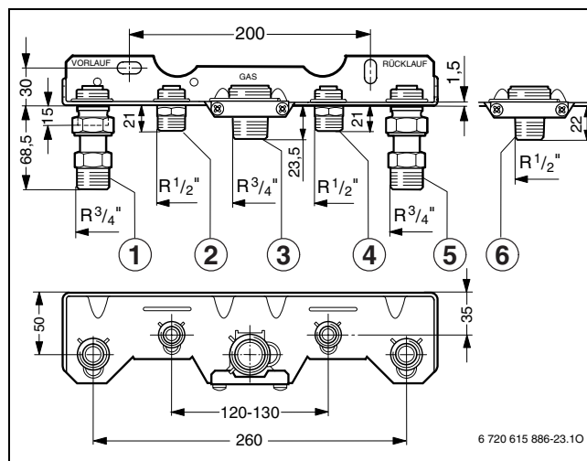
Obr. 7 Příklad: Montážní připojovací lišta č.258
