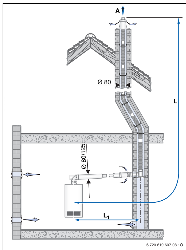
Obr. 15 Montážní varianta se stavební sadou GA-X + GA-K + ÜB-Flex
