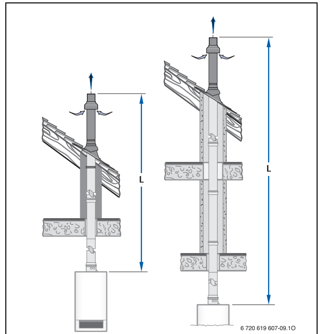
Obr. 17 Montážní varianty se stavební sadou DO (C 33x )
