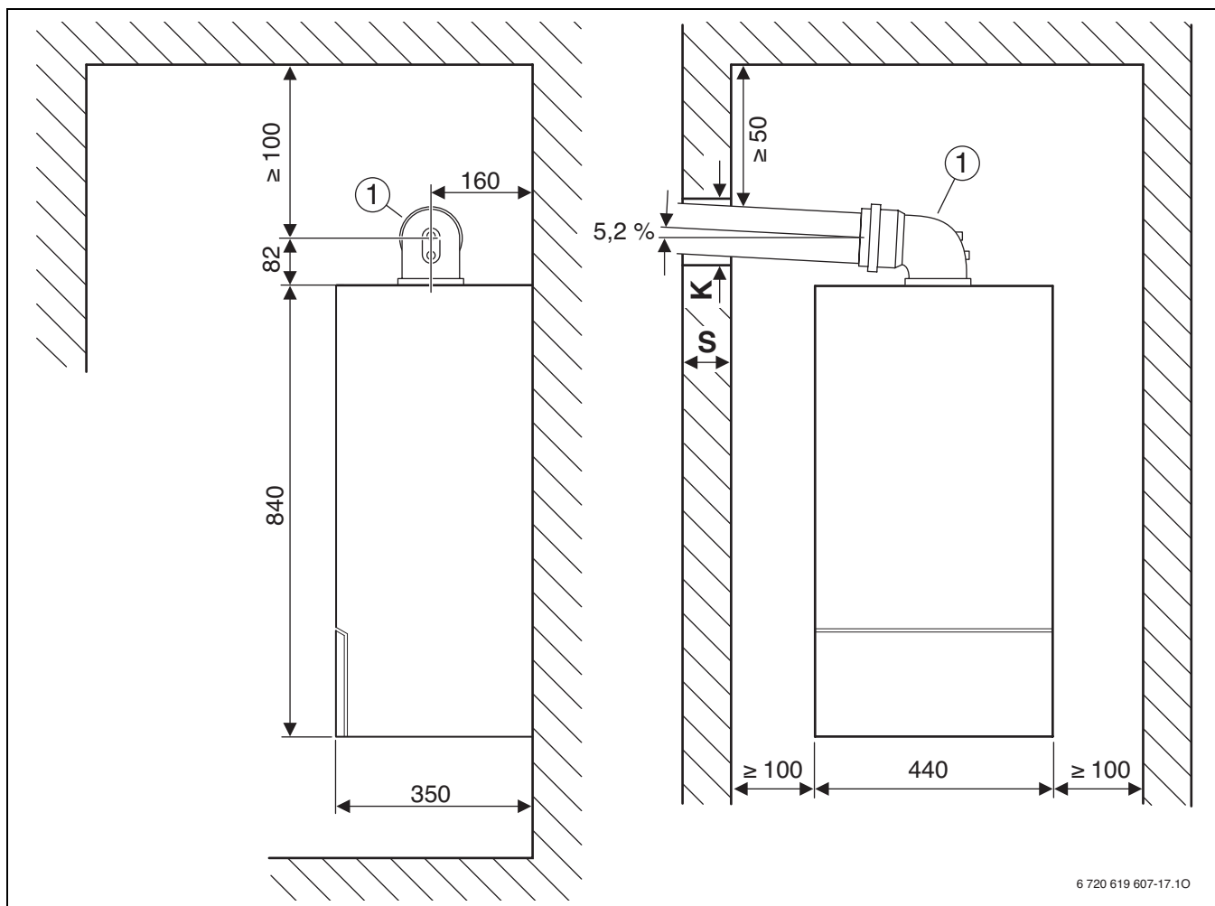
Obr. 9 Vedení spalin \varnothing 60/100 mm
