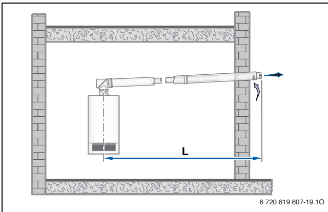
Obr. 16 Montážní varianty se stavební sadou WH/WS (C 13x )
