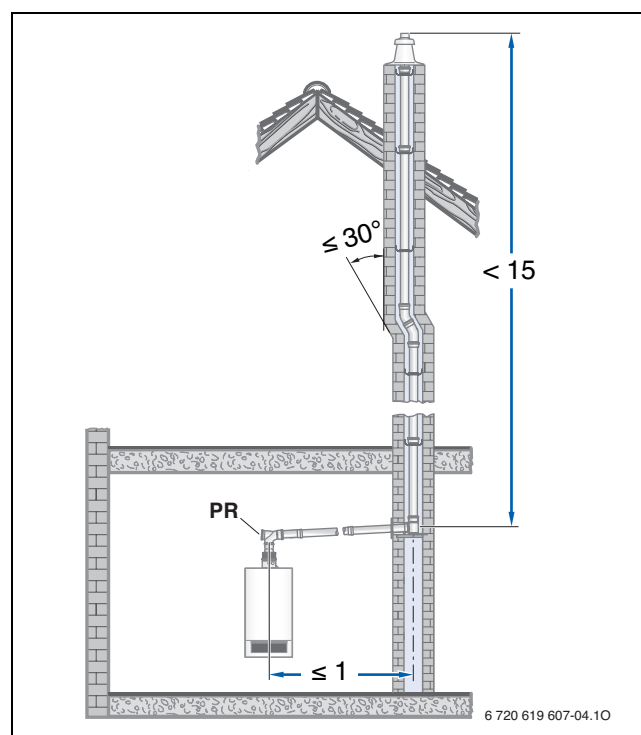
Obr. 4 Příklad umístění revizního otvoru u vodorovného spalinového potrubí bez ohybu v prostoru umístění (rozměry v m)
