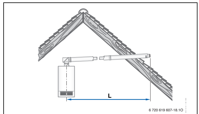
Obr. 18 Montážní varianty se stavební sadou WH/WS (C 33x )
