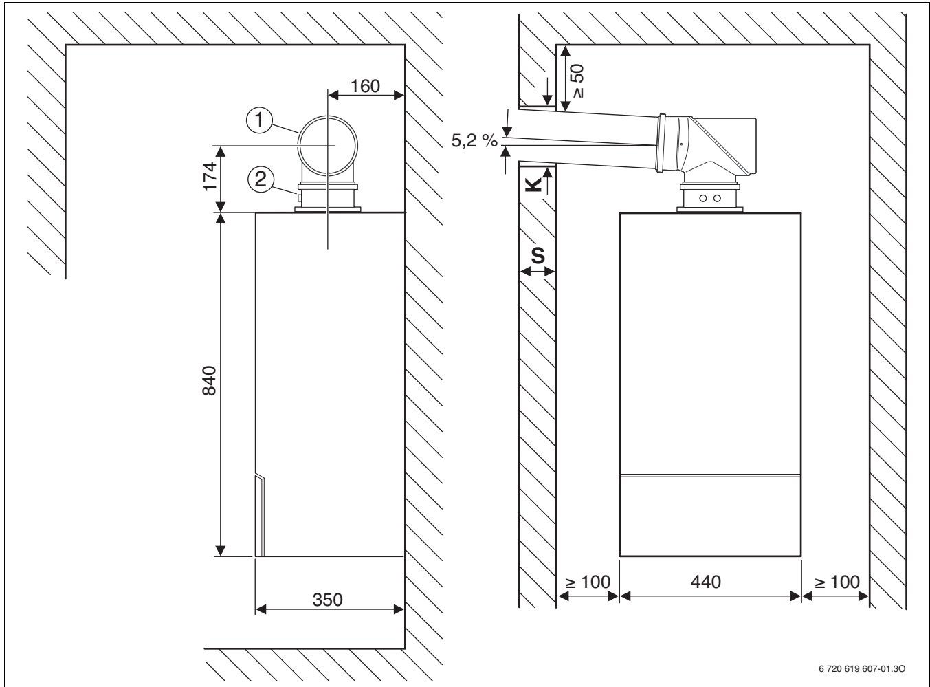
Obr. 8 Vedení spalin \varnothing 80/125 mm nebo \varnothing 80 mm
