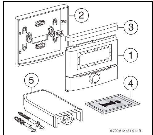
Obr. 4 Rozsah dodávky
