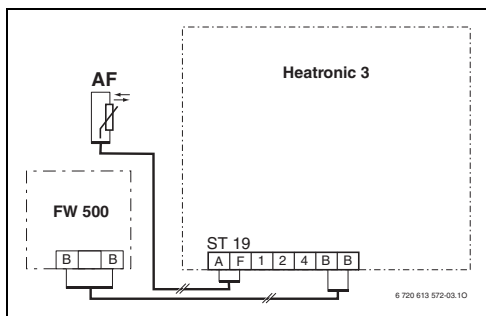
Obr. 17 Regulator připojený na jednotku Heatronic 3 vybavenou sběrníci BUS.
