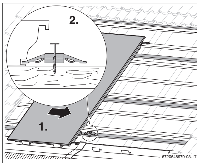
Obr. 48 Posunutí kolektoru doprava
