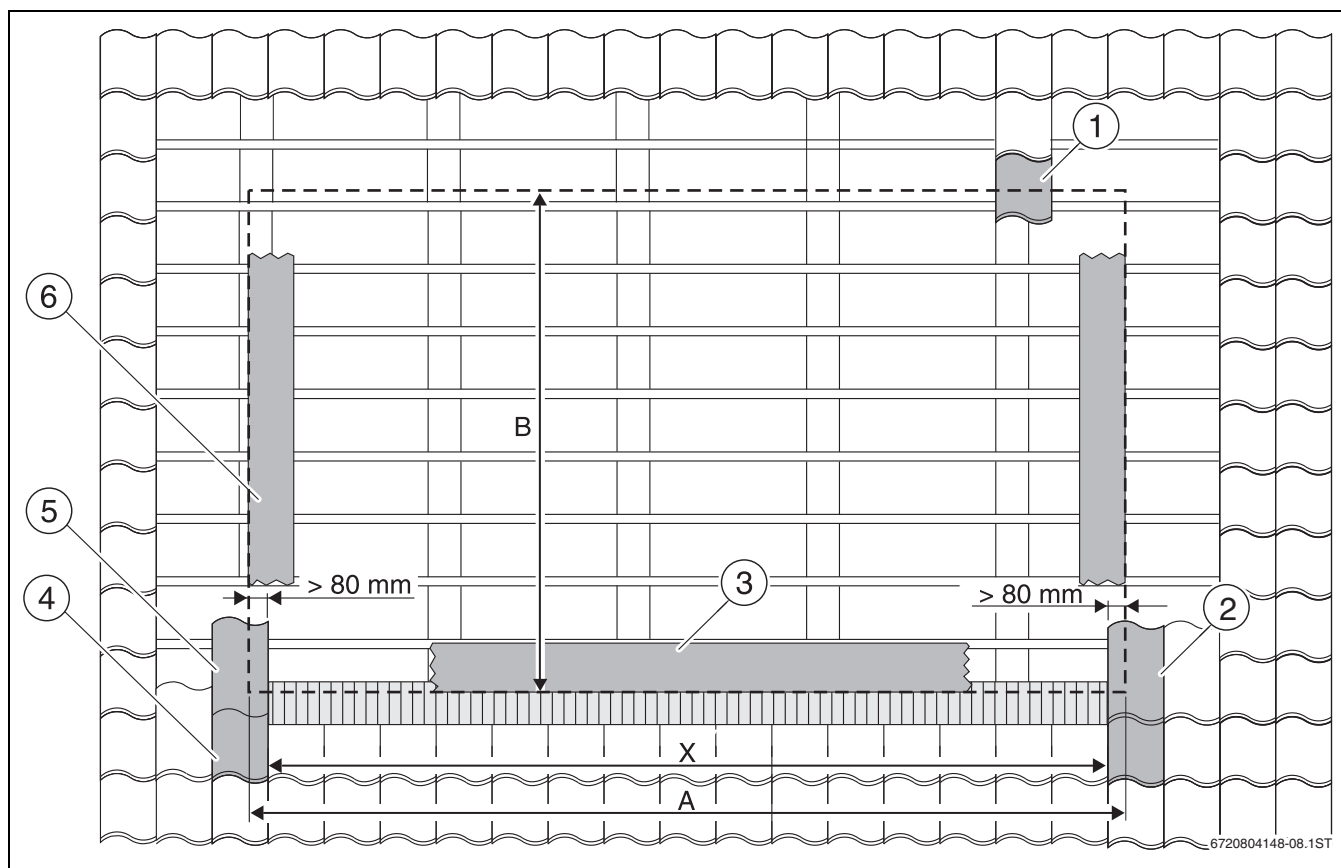
Obr. 25 Poloha kolektorového pole
