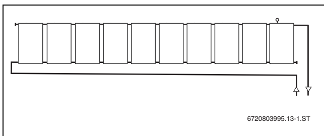
Obr. 23 Oboustranné připojení (1 řada)
