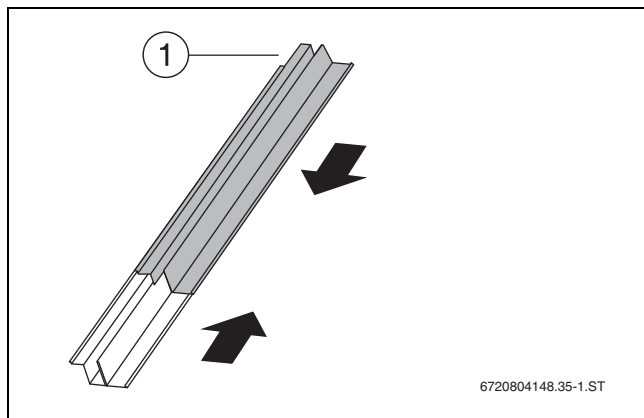
Obr. 68 Zasunutí bočních krycích plechů do sebe (svislé provedení)
