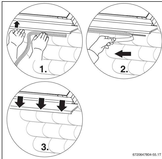
Obr. 86 Nalepení spodního krycího plechu na krytinu
