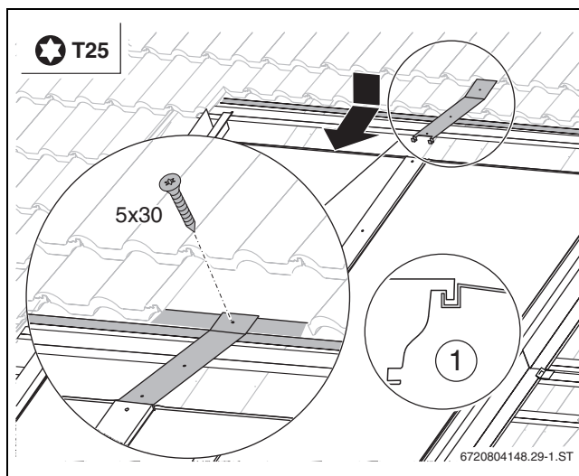
Obr. 75 Svislé uspořádání
