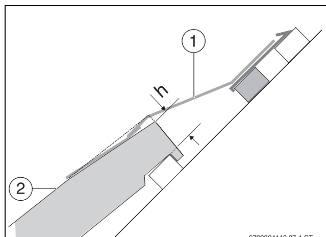
Obr. 27 Míra h
