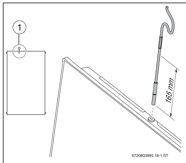
Obr. 61 Montáž čidla kolektoru
