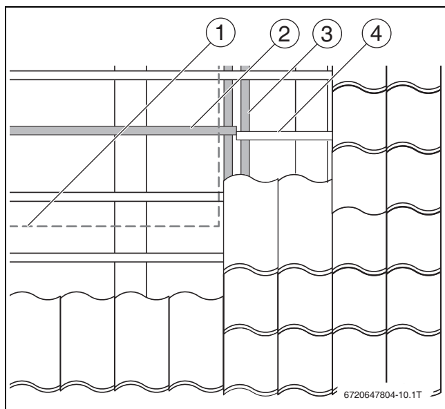
Obr. 31 Posunutí střešní latě
