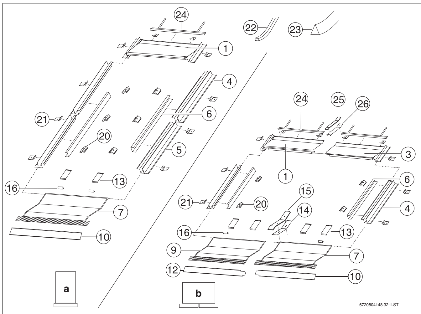
Obr. 11 Montážní sada pro 1 svislý resp. vodorovný kolektor: 1 montážní sada - základní provedení
