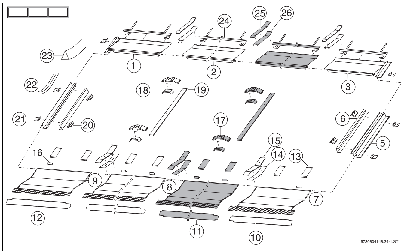
Obr. 8 Montážní sada pro 3 vodorovné kolektory: 1 montážní sada v základním provedení a 1 montážní sada jako rozšíření (šedá)
