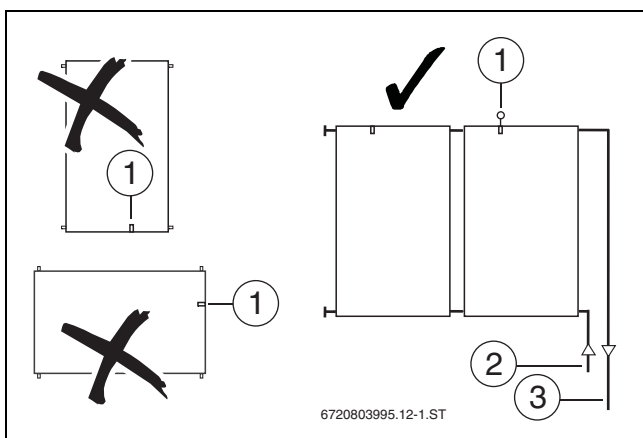
Obr. 21 Uspořádání kolektorů
