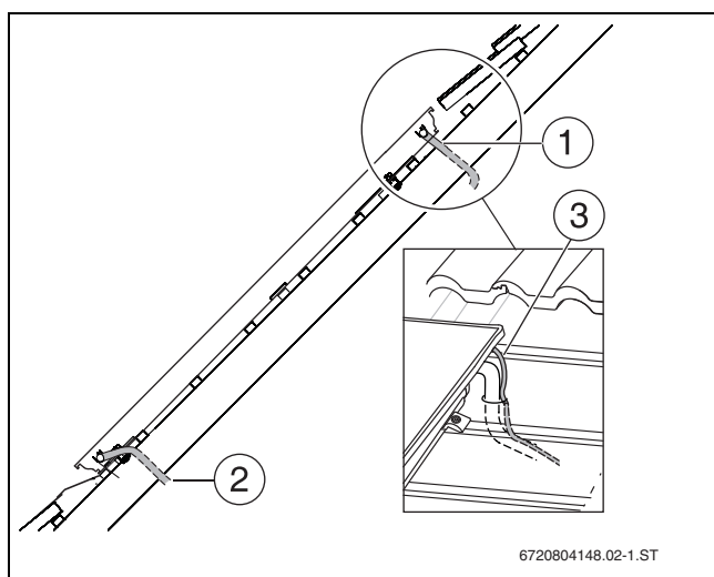
Obr. 62 Výstup a zpátečka
