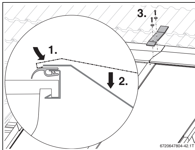
Obr. 81 Montáž horního dílu spojky
