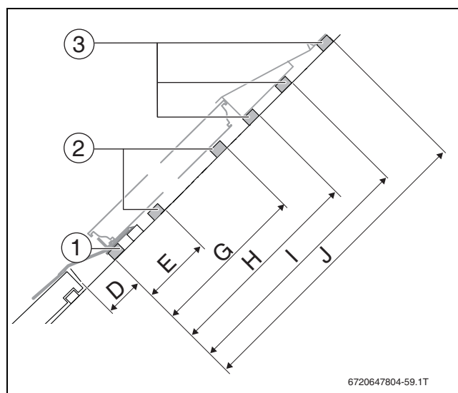
Obr. 30 Dodatečná montáž (vodorovný typ)
