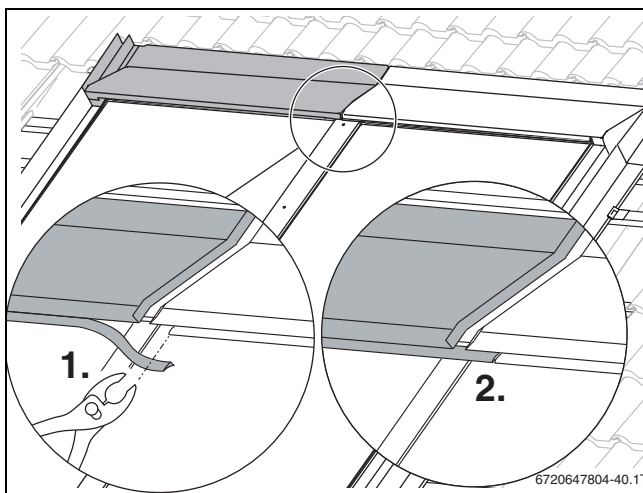
Obr. 79 Úprava těsnicího břitu
