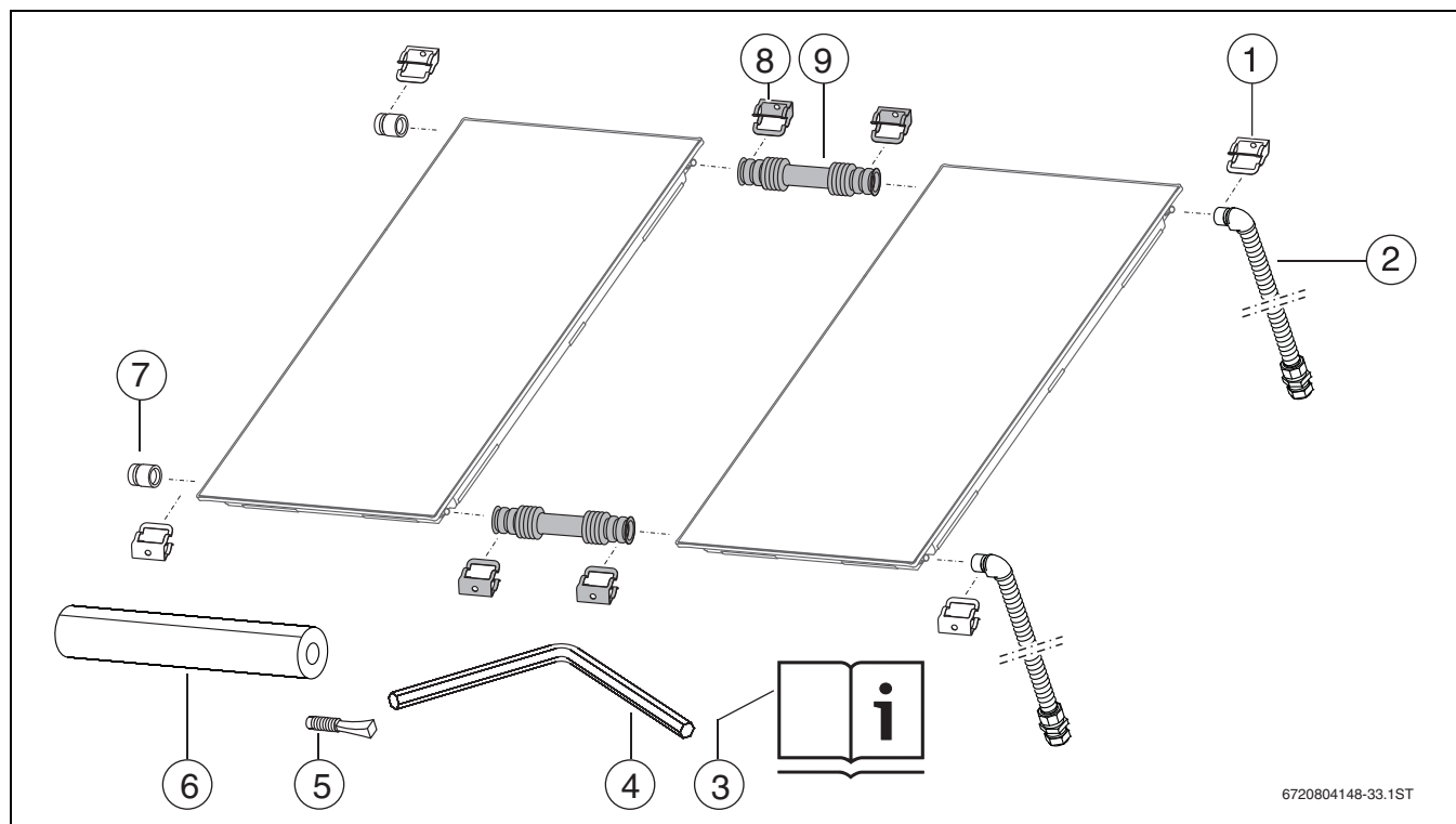
Obr. 14 1 připojovací sada do střechy a 2 propojovací sady (šedé)
