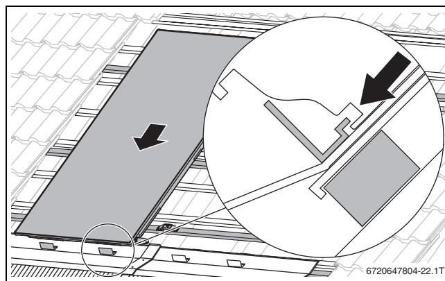
Obr. 47 Položení levého kolektoru
