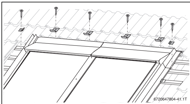
Obr. 80 Horní krycí plechy zajistěte příponkami
