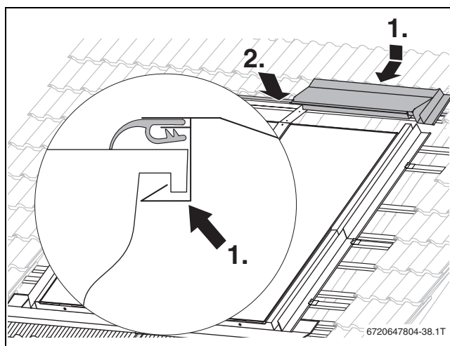
Obr. 77 Montáž pravého horního krycího plechu
