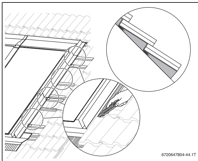
Obr. 83 Zaříznutí trojúhelníkového těsnicího pásu
