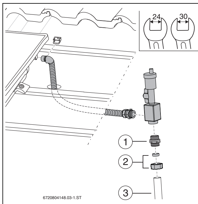
Obr. 66 Montáž automatického odvzdušňovače pod střechu
