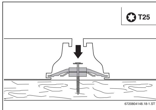
Obr. 57 Utažení šroubů
