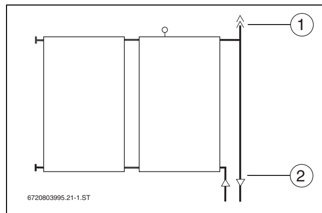
Obr. 64 Hydraulické zapojení s automatickým odvzdušňovačem
