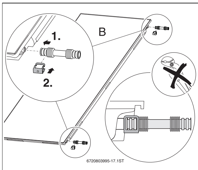
Obr. 46 Propojovací sada na druhém a všech dalších kolektorech
