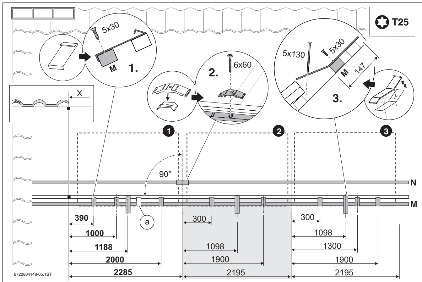
Obr. 38 Vodorovný typ kolektoru (3 kolektory), šedý úsek: při více než 2 kolektorech (tyto míry se opakují), rozměry v mm
