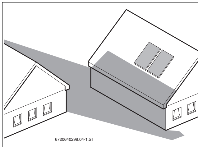
Obr. 19 Zábřana zastínění
