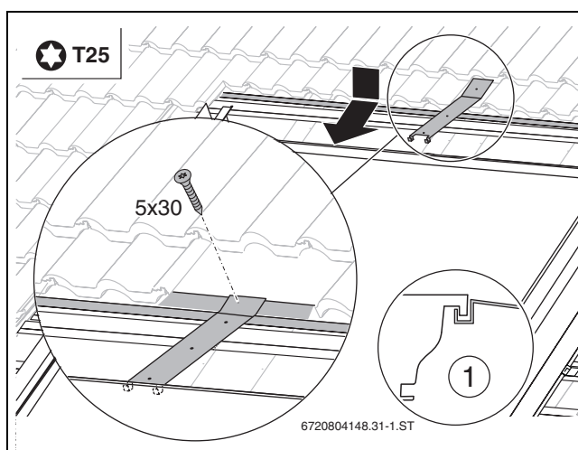
Obr. 76 Vodorovné uspořádání
