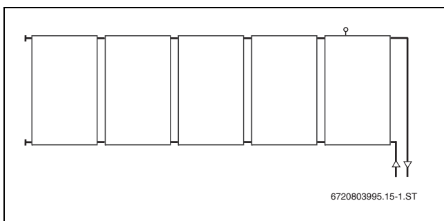
Obr. 22 Stejnostranné připojení vpravo nebo vlevo (1 řada)
