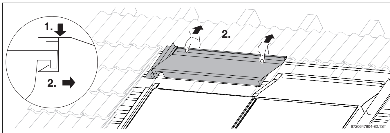
Obr. 90 Stažení horního krycího plechu
