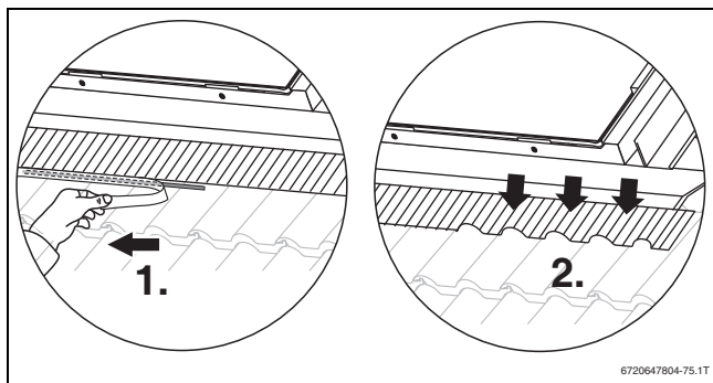
Obr. 85 Nalepení olověné zástěry na krytinu
