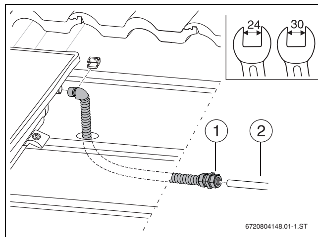
Obr. 63 Protažení potrubí (výstup) střechou
