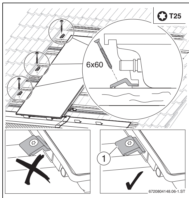
Obr. 50 Pevné přišroubování přídržovače
