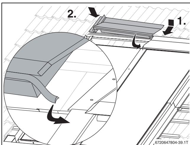
Obr. 78 Montáž levého horního krycího plechu
