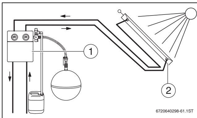
Obr. 20 Výstup u střešních kotelen
