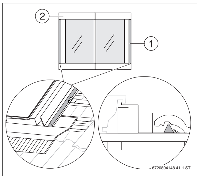
Obr. 82 Vložení trojúhelníkového těsnicího pásu
