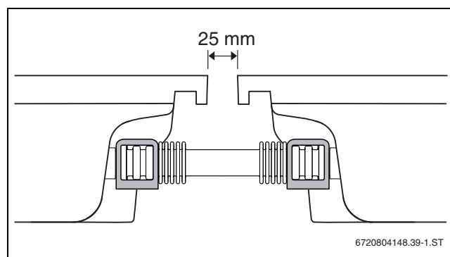
Obr. 56 Zajištěná vlnovcová spojka
