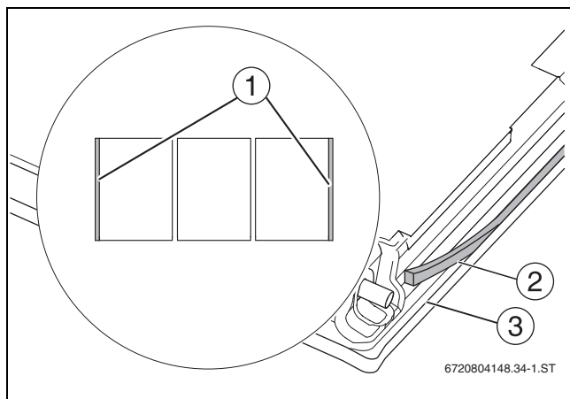
Obr. 45 Vložení těsnicí pásky (zadní strana kolektoru)
