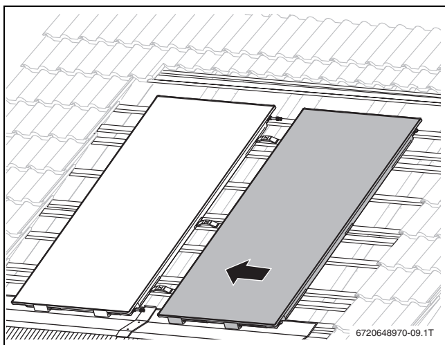
Obr. 54 Posunutí pravého kolektoru doleva
