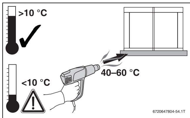
Obr. 84 Zahřátí olověné zástěry, je-li to nutné
