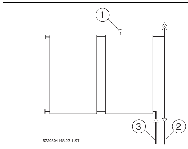
Obr. 60 Poloha čidla kolektoru
