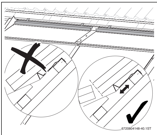
Obr. 87 Úprava polohy podložky tašek
