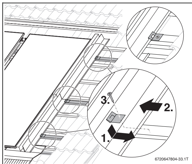
Obr. 71 Montáž příponek
