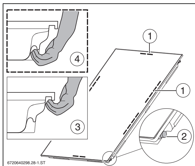
Obr. 17 Přenášení kolektoru
