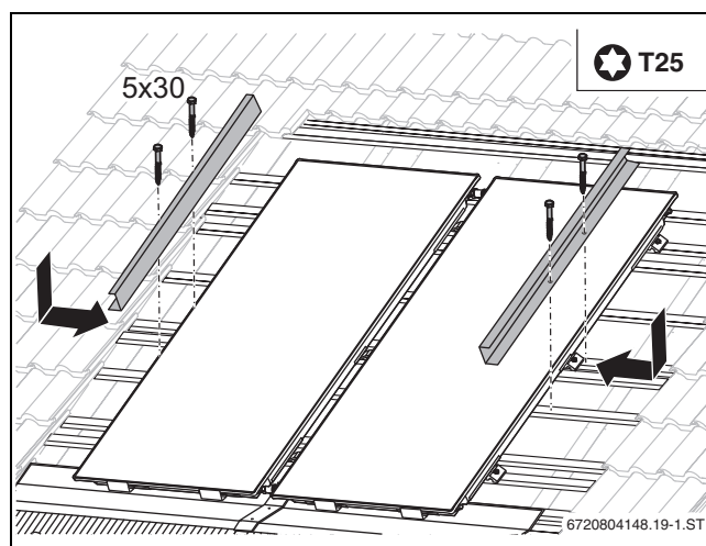
Obr. 67 Montáž bočních opěrných plechů
