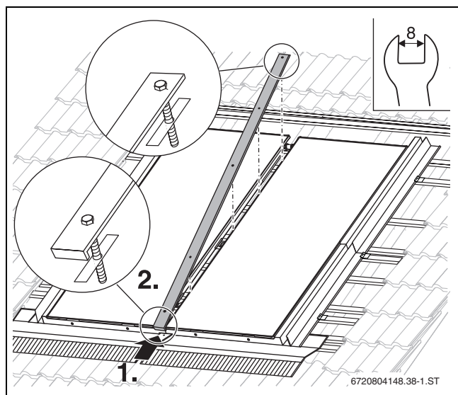
Obr. 74 Montáž krycí lišty
