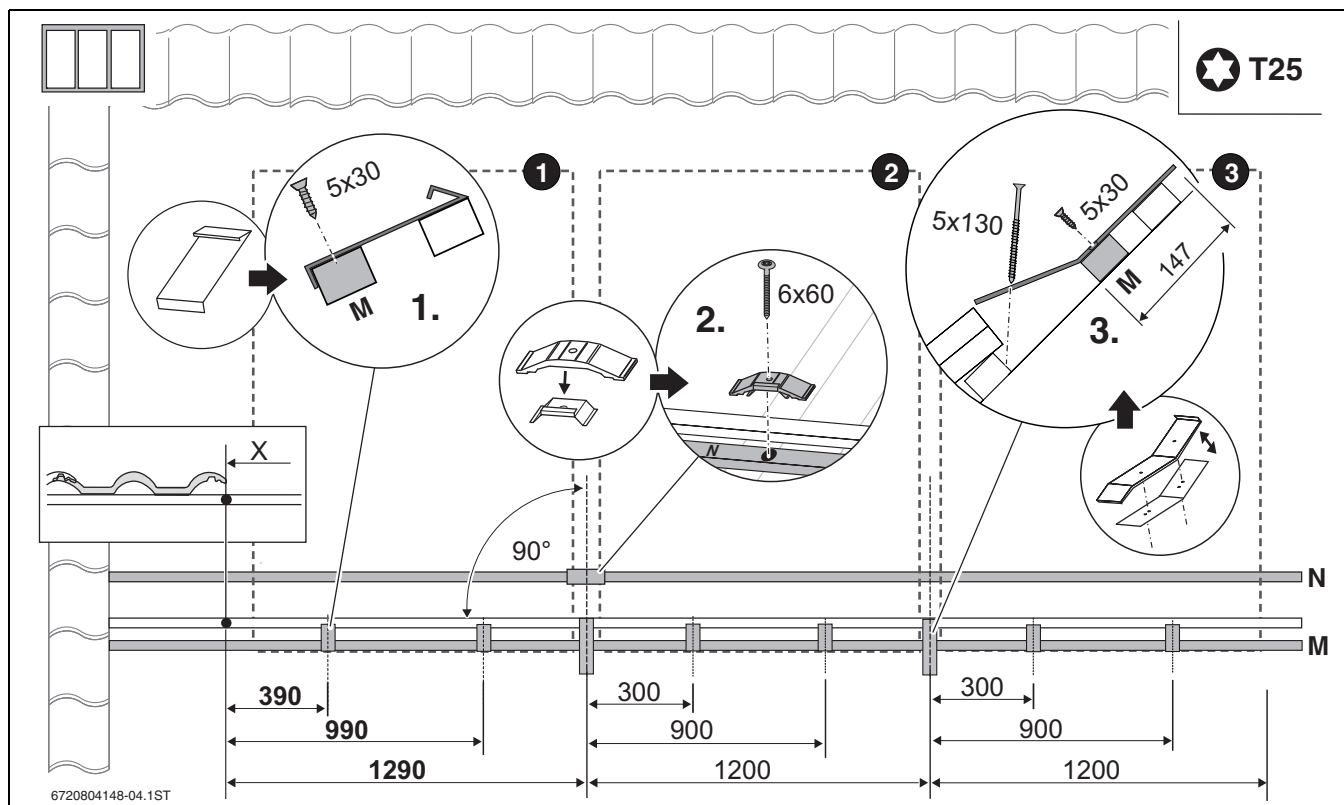
Obr. 37 Svislý typ kolektoru (3 kolektory), rozměry v mm
