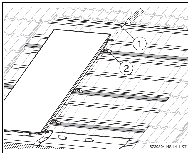
Obr. 51 Montážní poloha horní spojky
