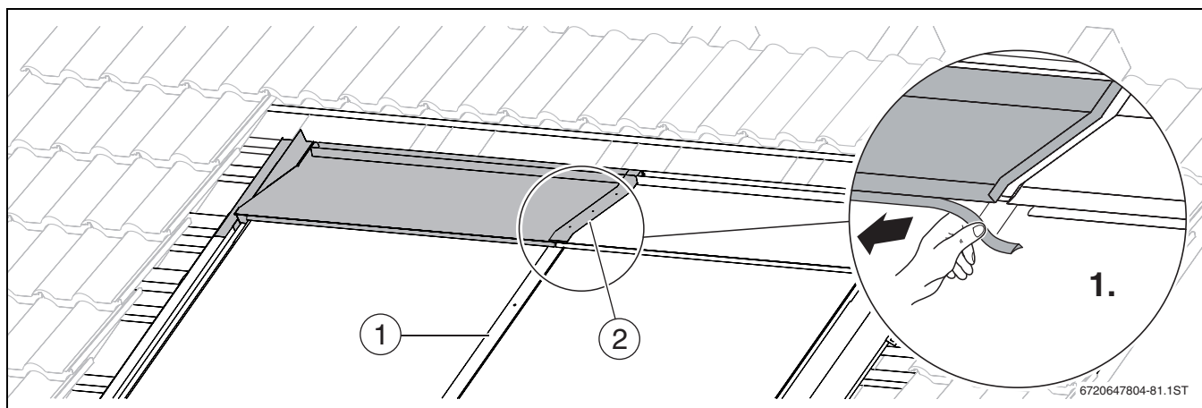
Obr. 89 Stažení těsnícího břítu
