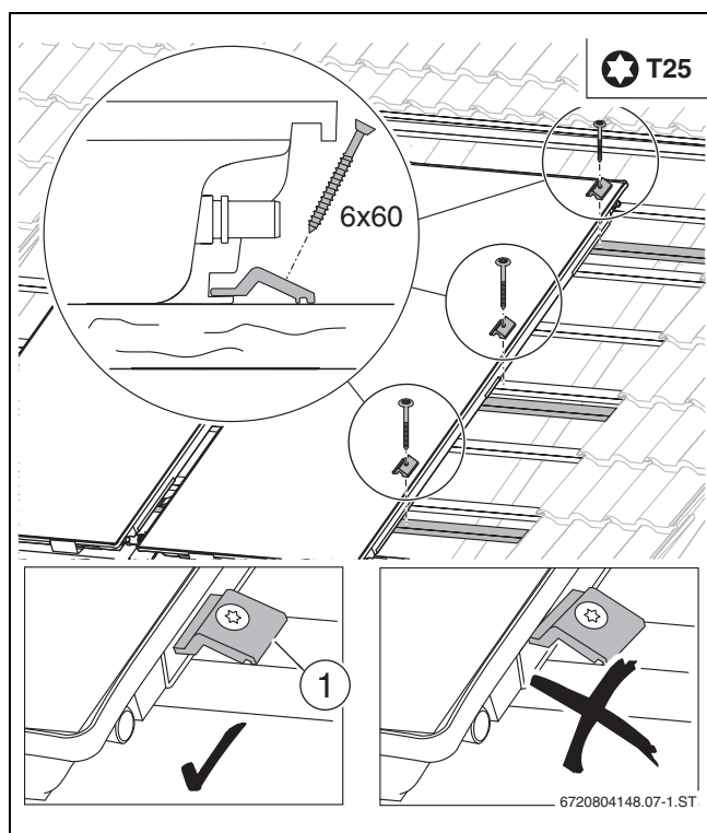
Obr. 59 Pevné přišroubování přídržovače
