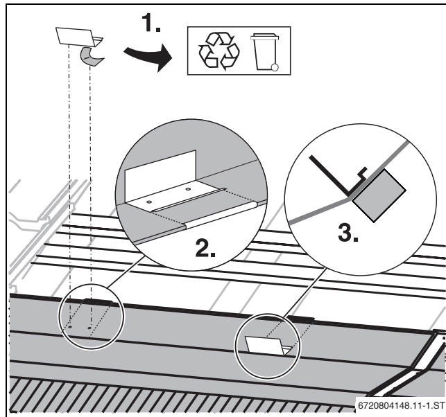
Obr. 41 Umístění pojistek proti sklouznutí do správné polohy a nalepení
