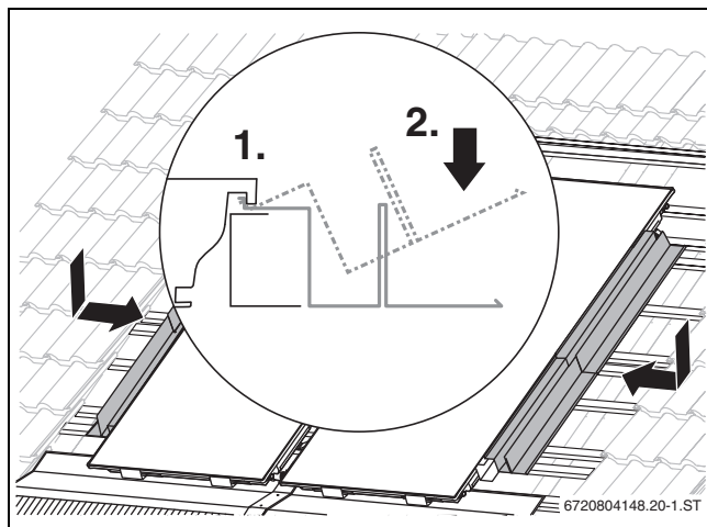
Obr. 69 Montáž bočních krycích plechů
