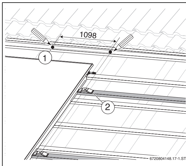
Obr. 52 Montážní poloha horní spojky u vodorovných kolektorů
