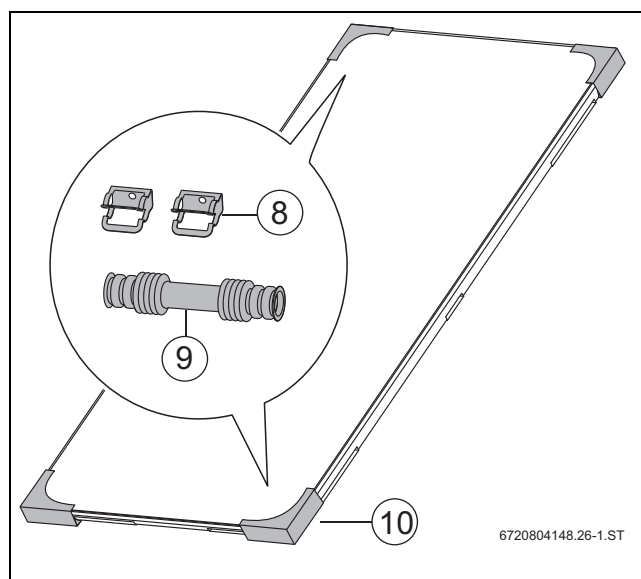
Obr. 15 2 přepravní ochranné rohy obsahují po 1 propojovací sadě (1 propojovací sada obsahuje 2 svorky a 1 vlnovcovou spojku)
