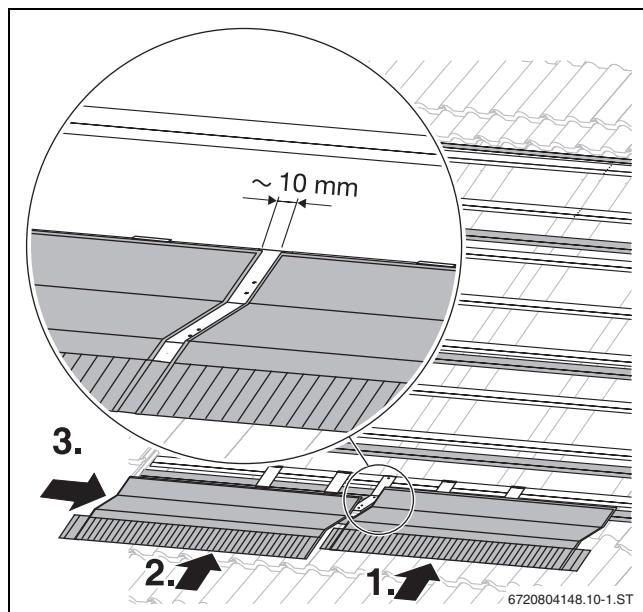
Obr. 40 Krycí plechy pro 2 kolektory
