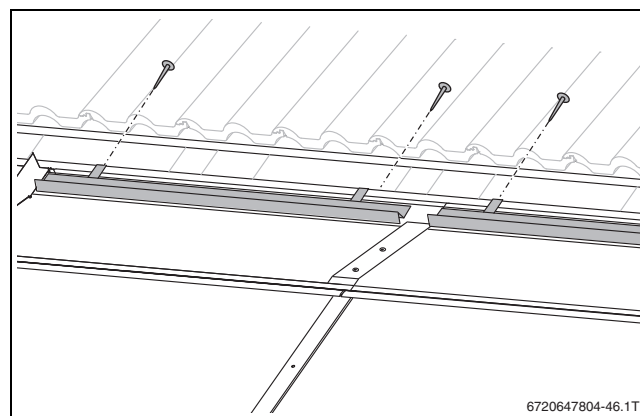
Obr. 88 Připevnění podložky tašek
