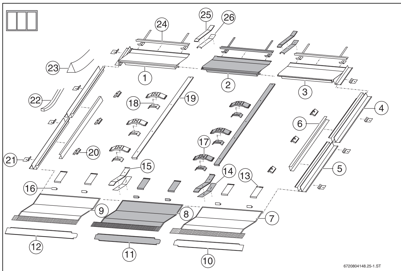
Obr. 5 Montážní sada pro 3 svislé kolektory: 1 montážní sada v základním provedení a 1 montážní sada jako rozšíření (šedá)
