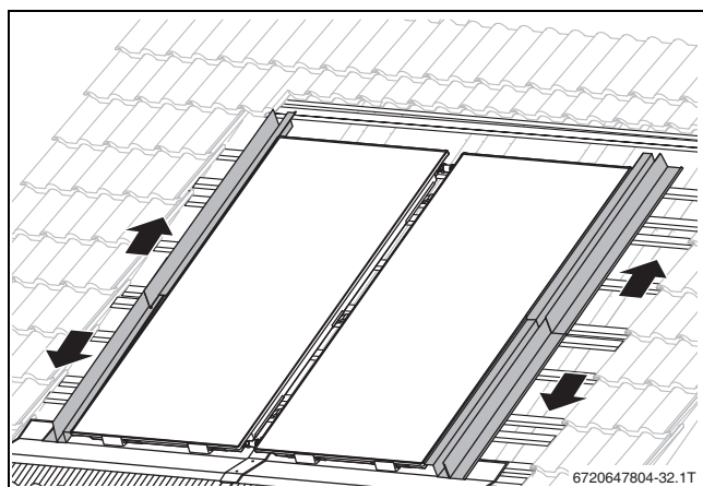
Obr. 70 Roztažení bočních krycích plechů (svislé provedení)
