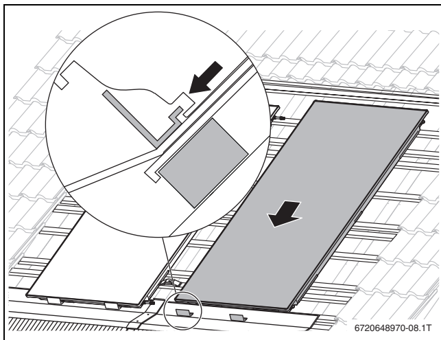
Obr. 53 Položení pravého kolektoru
