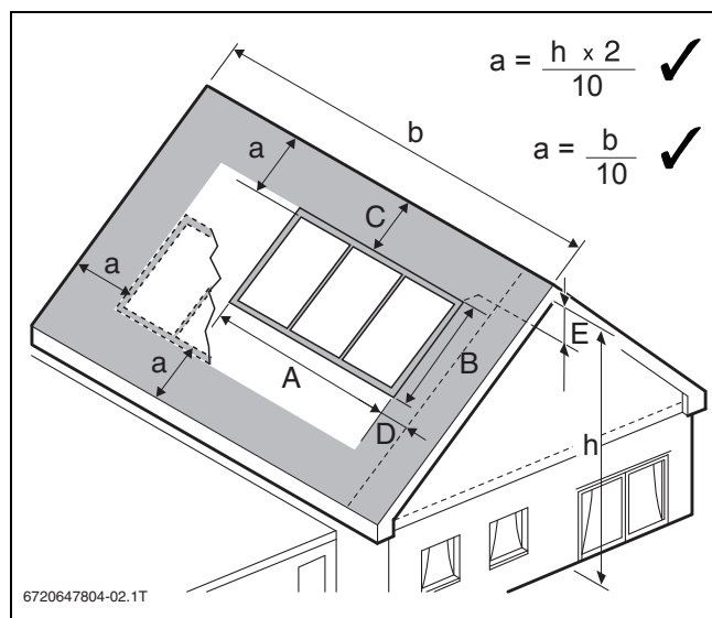
Obr. 24 Míry odstupů na střeše
