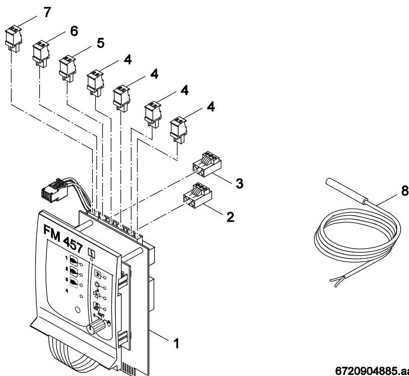
6720904885.aa.RS-Modul FM457
