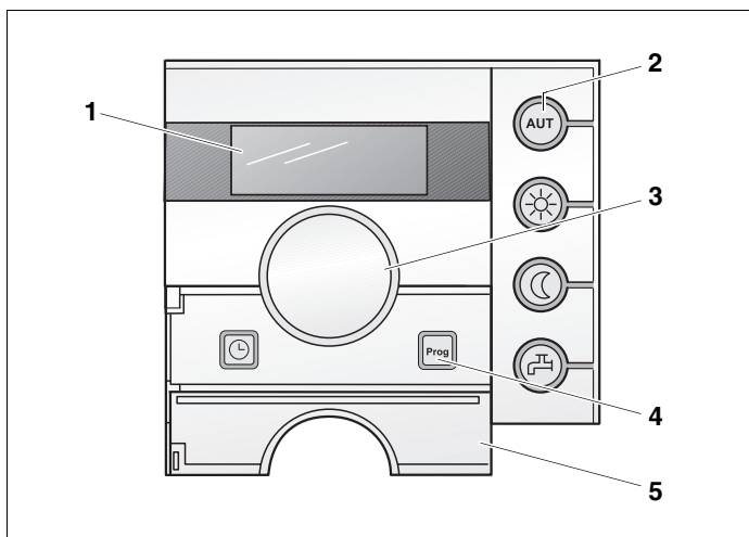
Obr. 4 Ovládací prvky RC20RF
