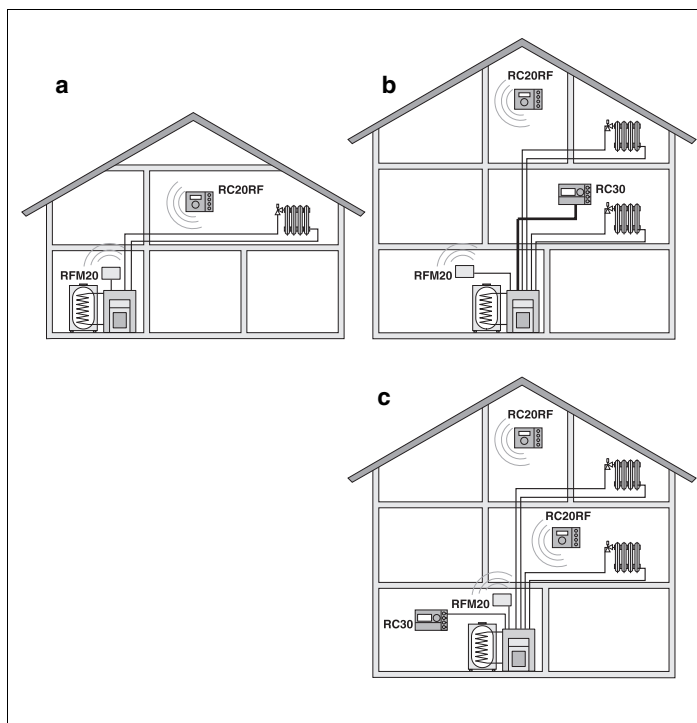
Obr. 3 Bezdrátový regulační přístroj pro montáž do místnosti RC20RF jako jediná obsluhovaná jednotka (a) nebo jako dálkové ovládání pro jeden vytápěcí okruh v dvougeneračním rodinném domě (b nebo c)
