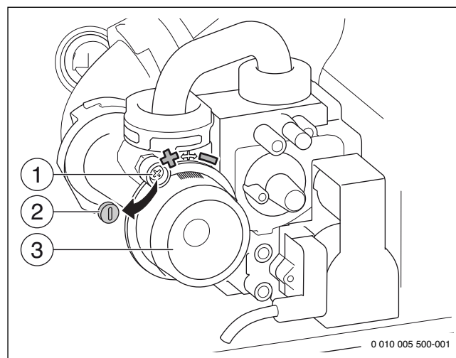
Obr. 86 Nastavení poměru plyn-vzduch
