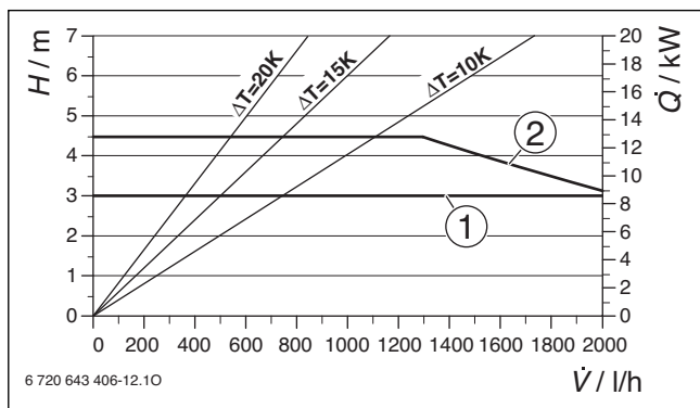
Obr. 123 Charakteristiky čerpadla
