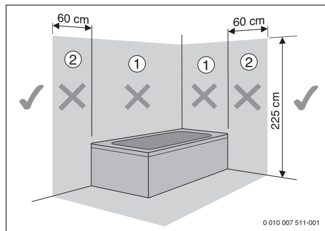
Obr. 63 Ochranné úseky
