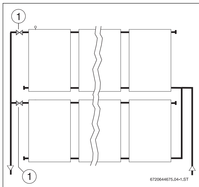
Obr. 73 Výplach paralelně propojených kolektorových polí
