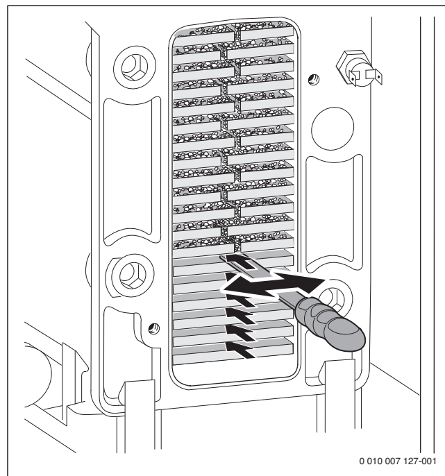
Obr. 97 Čisticí nůž
