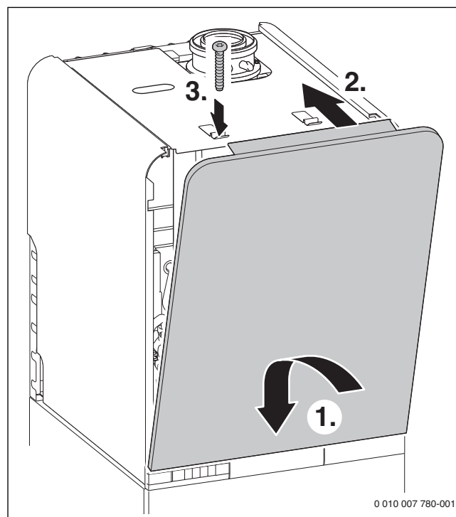
Obr. 79 Zavěšení předního opláštění a zajištění šroubem z rozsahu dodávky
