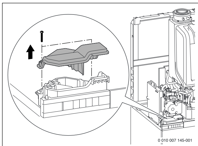
Obr. 64 Odstranění krytu připojovacího boxu
