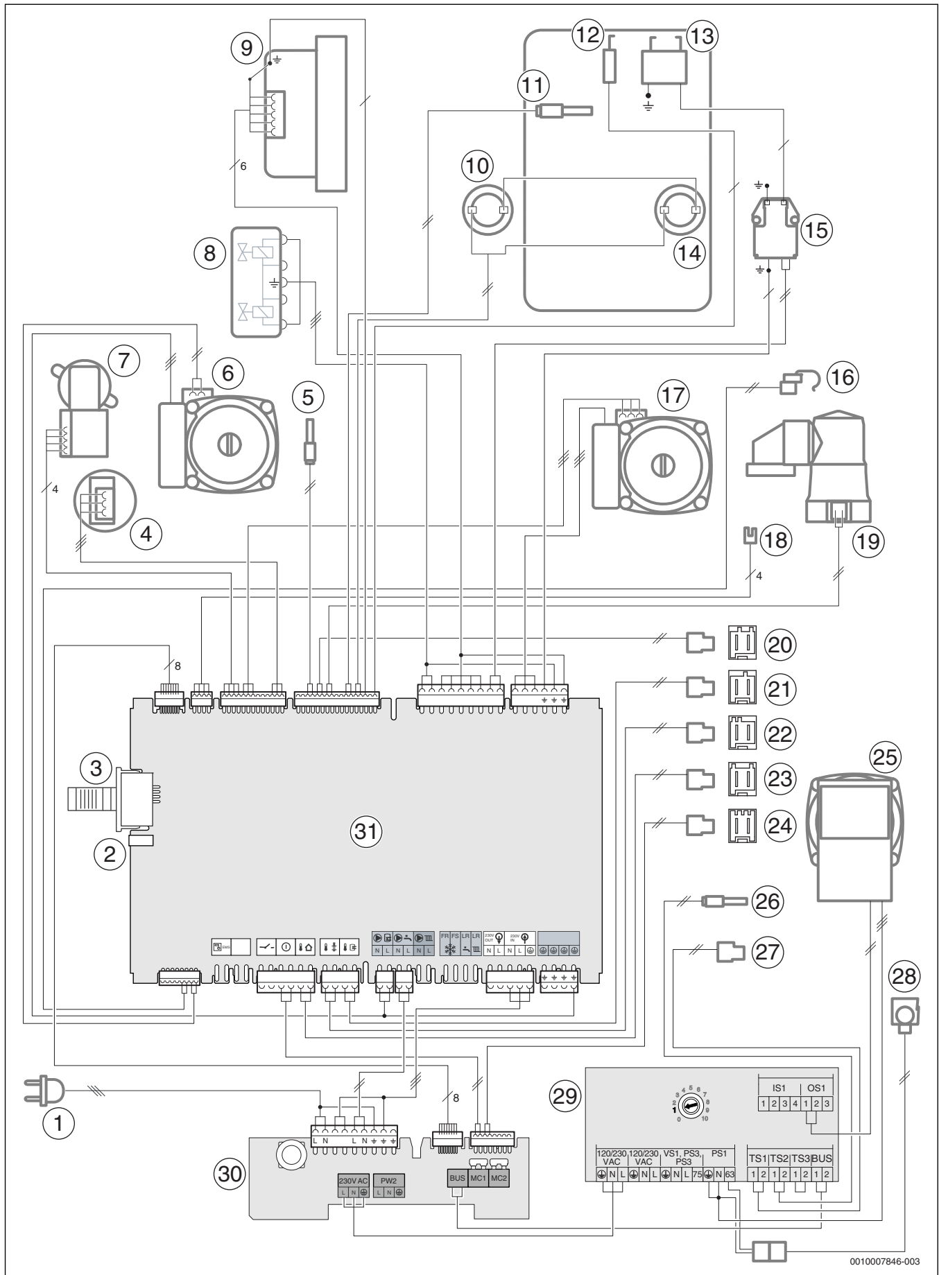
Obr. 113 Elektrické kabelové propojení
