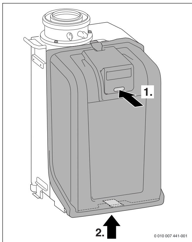
Obr. 85 Sejmutí krytu hořáku
