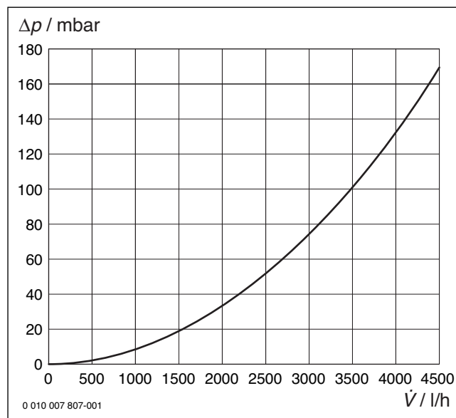
Obr. 116 Graf tlakové ztráty směšovaného otopného okruhu (HK2)
