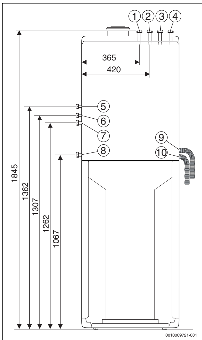
Obr. 7 Připojovací rozměry příslušenství CS 12 - Rozšíření otopného okruhu 1 (rozměry v mm)
