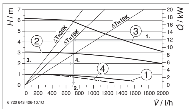
Obr. 119 Charakteristiky čerpadla
