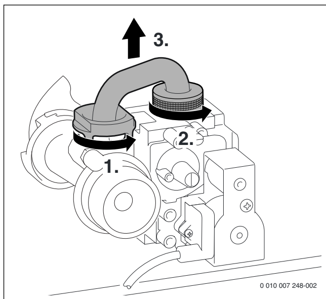
Obr. 107 Demontáž přívodního potrubí plynu
