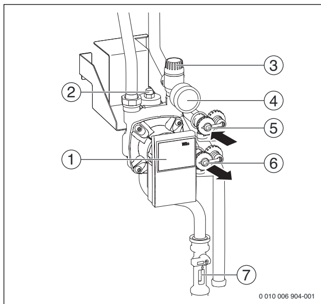
Obr. 75 Přehled solární skupiny
