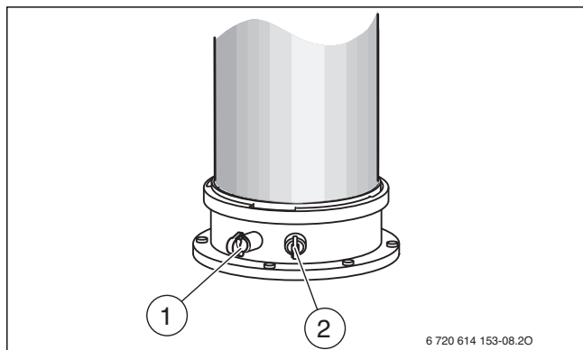
Obr. 90 Měřící hrdlo spalin a měřící hrdlo spalovacího vzduchu
