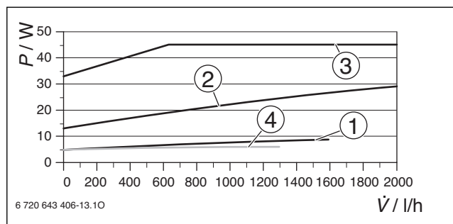
Obr. 120 Příkon
