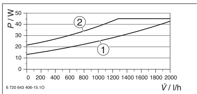
Obr. 124 Příkon
