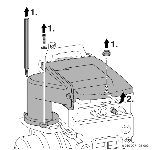
Obr. 93 Uvolnění vrchní části hořáku
