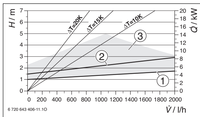
Obr. 121 Charakteristiky čerpadla
