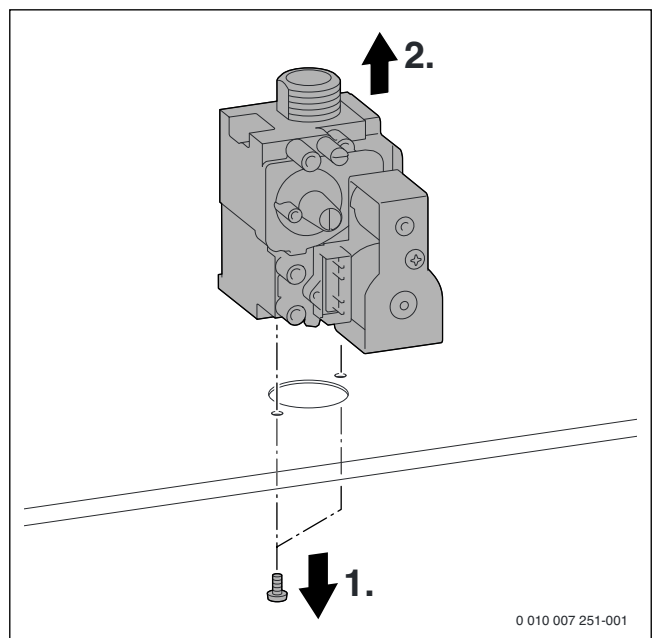
Obr. 109 Demontáž plynové armatury
