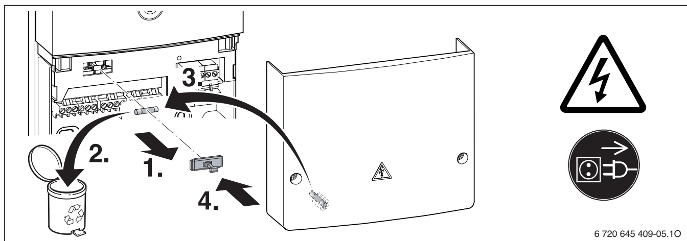
Obr. 112 Výměna pojistky modulu
