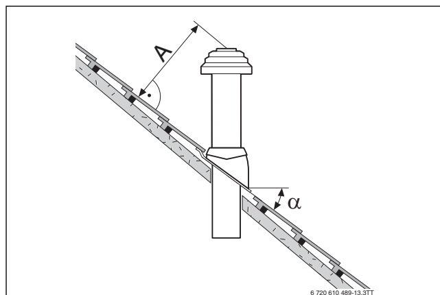
Obr. 15 Vzdálenosti a střešní sklonu u šikmé střechy
