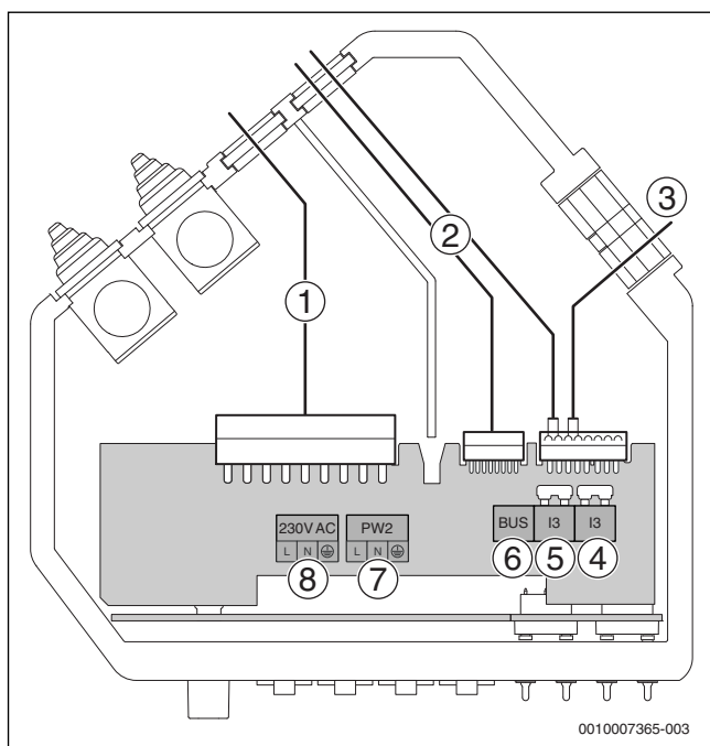
Obr. 66 Připojovací box
