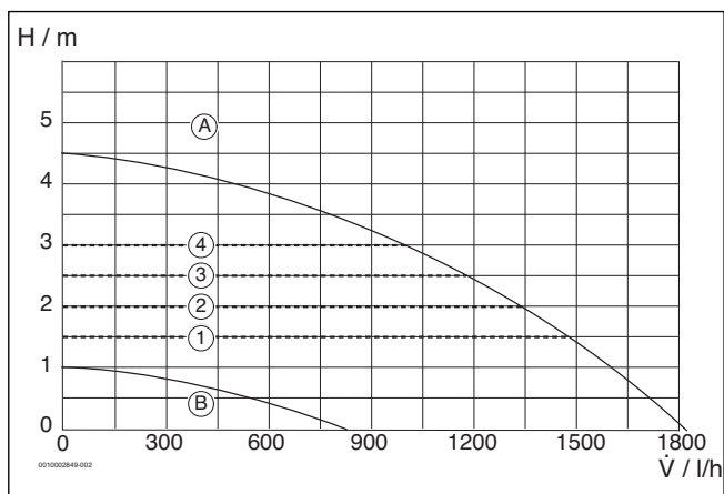
Obr. 114 Pole charakteristik čerpadla a charakteristiky čerpadla
