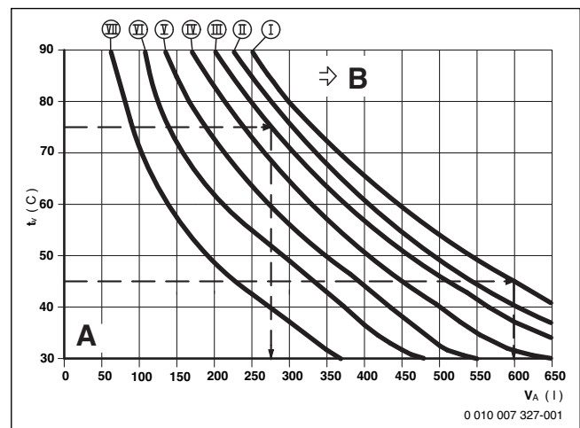
Obr. 30 Charakteristiky expanzní nádoby 18 l
