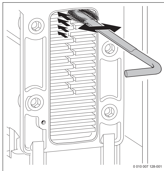
Obr. 98 Čištění tepelného bloku kartáčem
