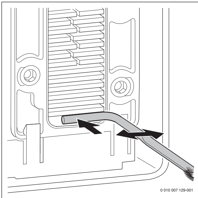
Obr. 100 Čištění vany kondenzátu
