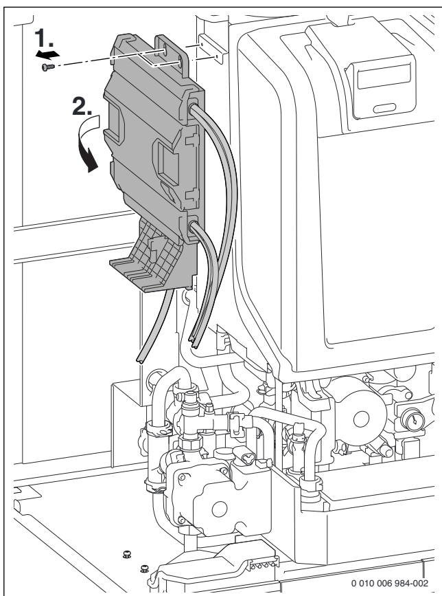
Obr. 46 Sejmутí řídicí jednotky
