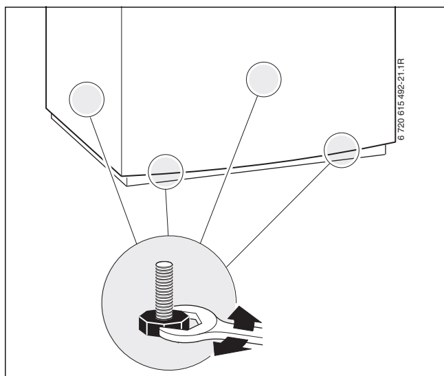
Obr. 37 Vyrovnání zásobníku
