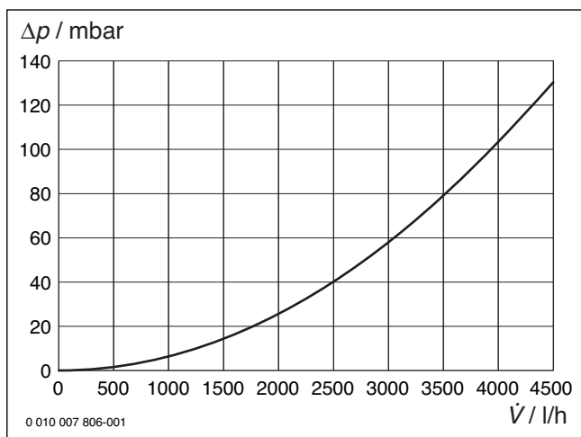
Obr. 115 Graf tlakové ztráty nsměšovaného otopného okruhu (HK1)
