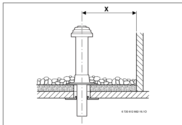
Obr. 14 Odstupy u ploché střechy
