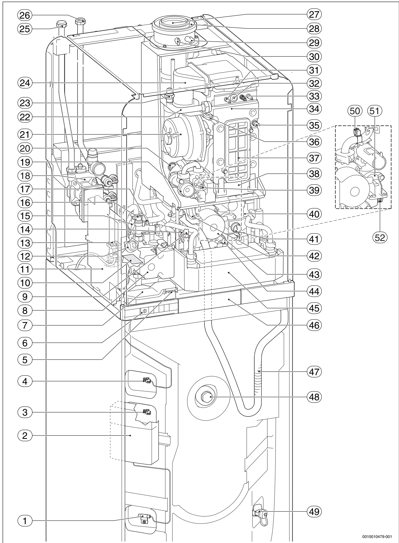
Obr. 12 GC9000iWM.../210 S zařízení
