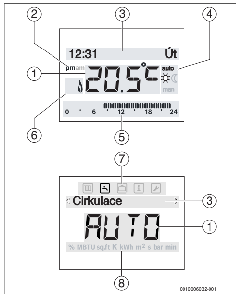
Obr. 2 Symboly na displeji (vzorová znázornění)
