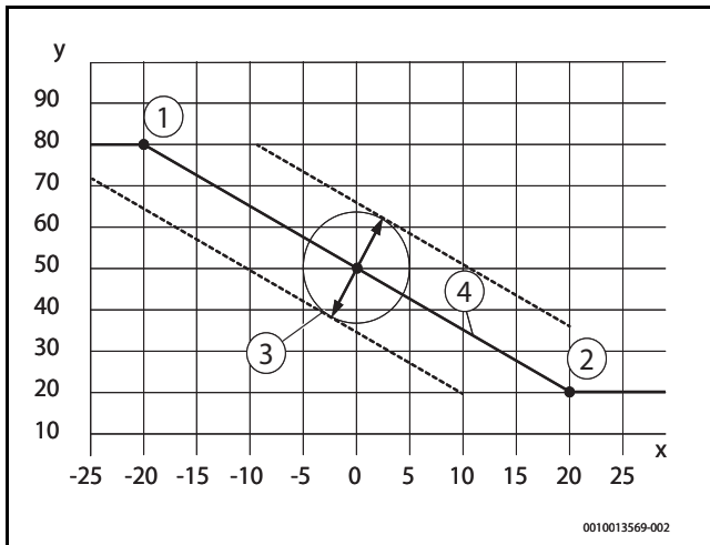
Obr. 4 Ekvitermní křivka
