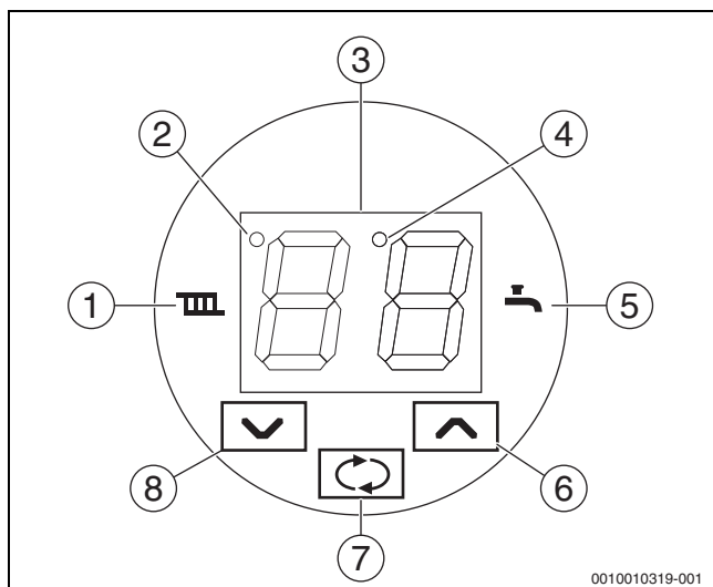
Obr. 3 Ovládací panel
