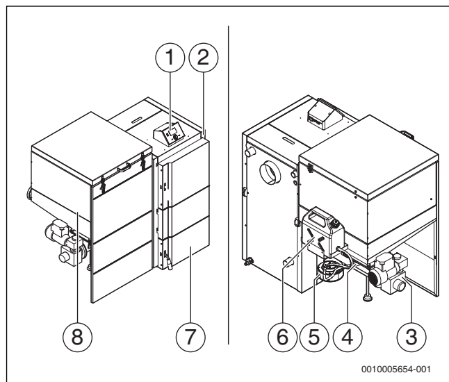
Obr. 59 Konstrukční uspořádání
