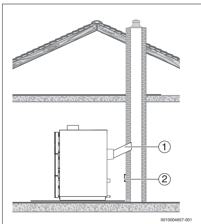
Obr. 48 Připojení odtahu spalin
