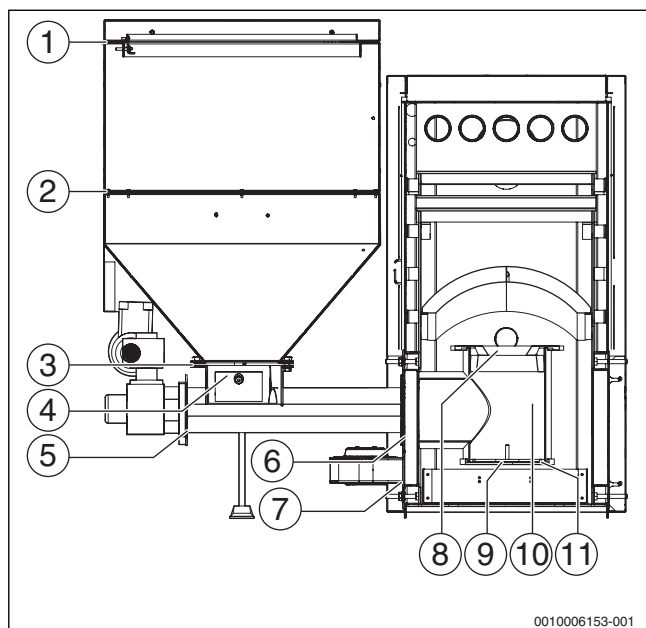
Obr. 68 Těsnicí místa
