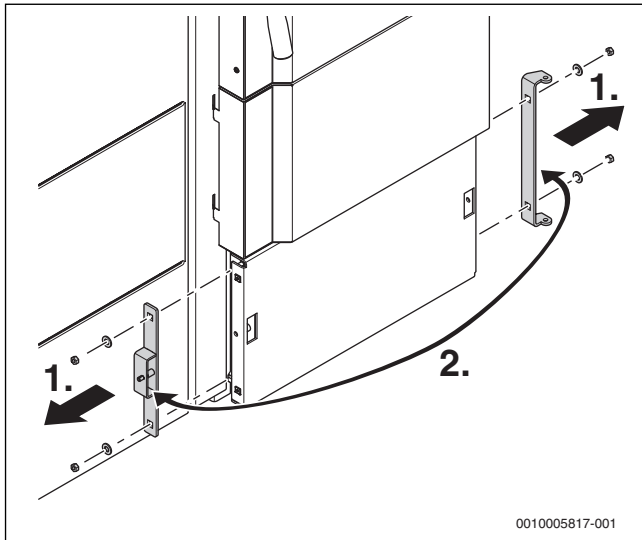
Obr. 37 Přestavba závěsů a třmenů madla
