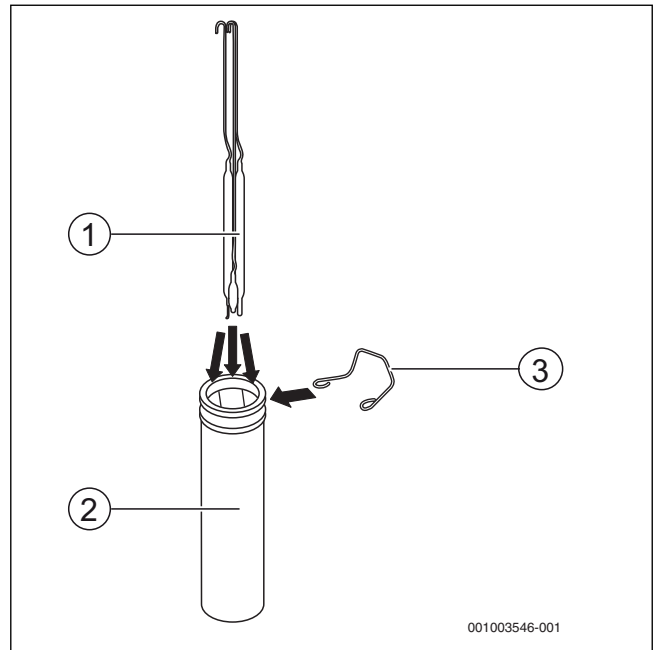
Obr. 38 Montáž čidel teploty
