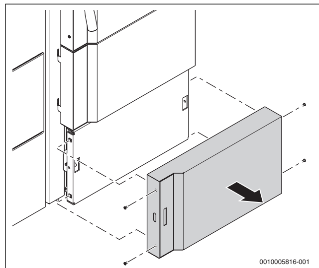
Obr. 36 Demontáž opláštění dvířek
