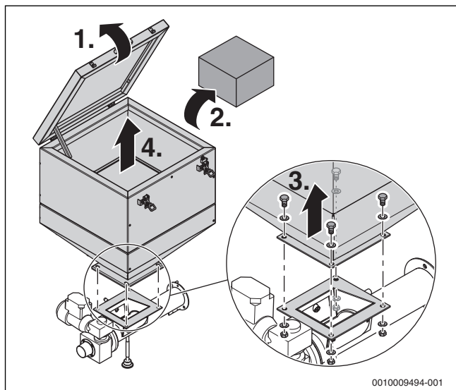
Obr. 11 Demontáž zásobníku
