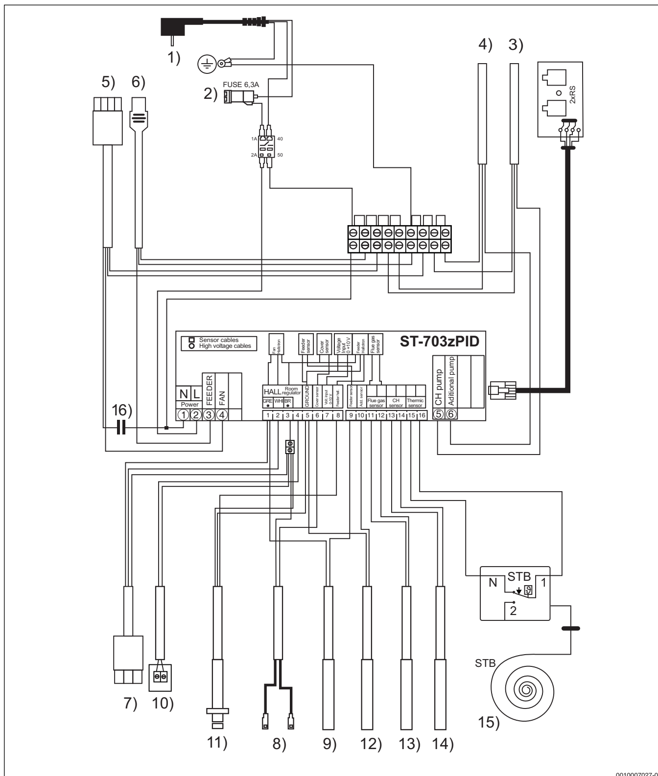
Obr. 72 Schéma zapojení regulačního přístroje
