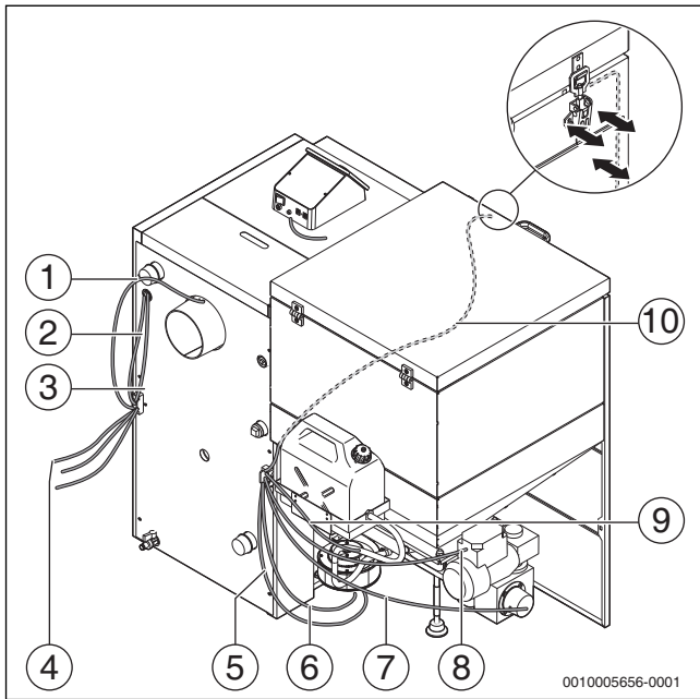
Obr. 44 Připojky
