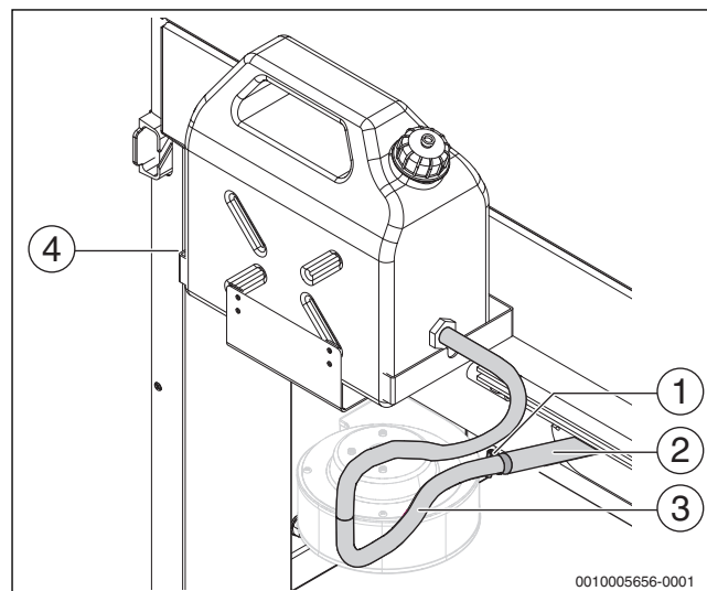
Obr. 49 Hasicí systém (pohled zezadu)
