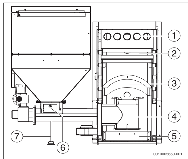
Obr. 9 Řez kotlem
