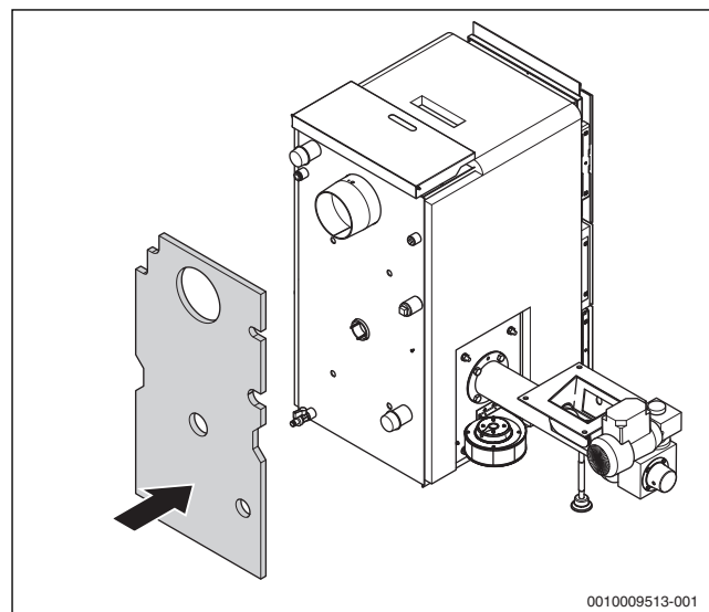
Obr. 26 Nasazení zadní izolace na kotel
