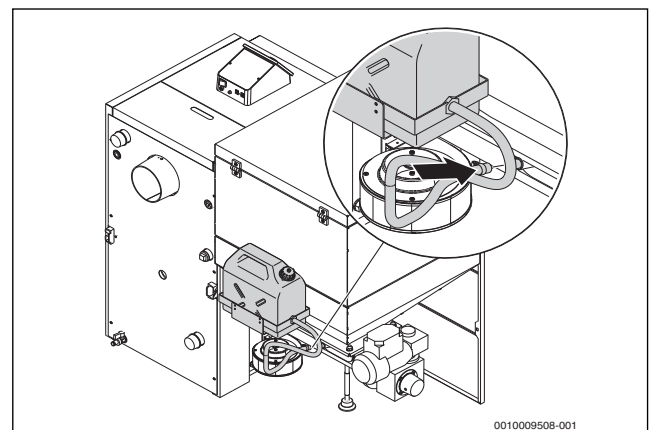
Obr. 47 Instalace hasičího systému
