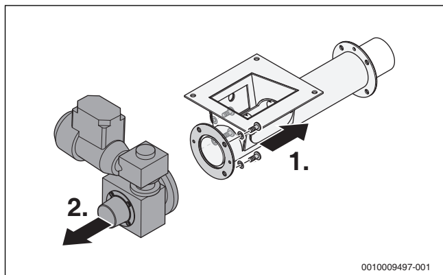
Obr. 12 Demontáž pohonu
