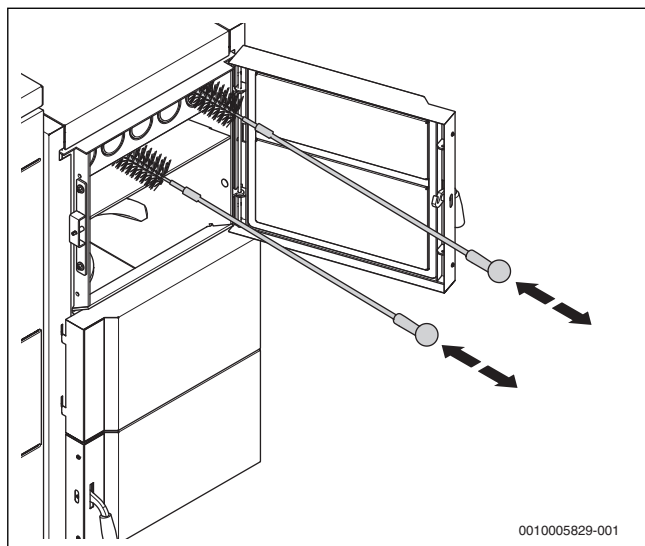
Obr. 63 Čištění trubek
