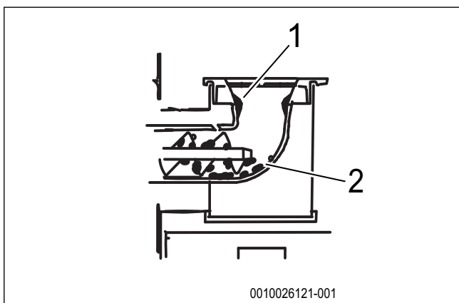
Obr. 52 Tvorba nápeků a strusky v retortě hořáku
