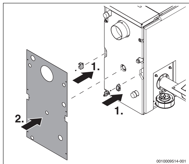
Obr. 27 Přišroubování kabelových držáků a zavěšení opláštění
