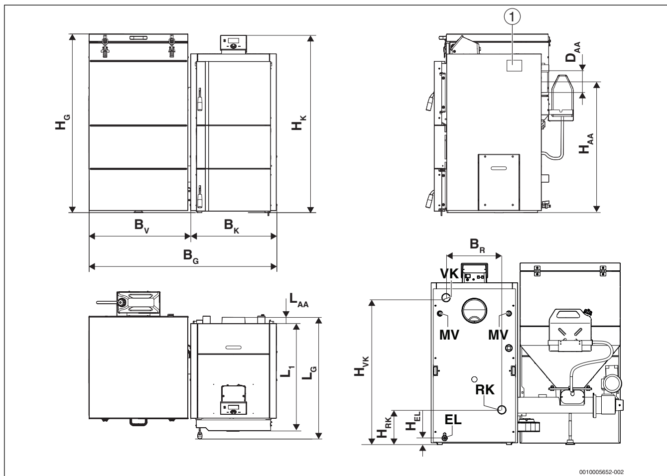
Obr. 7 Rozměry
