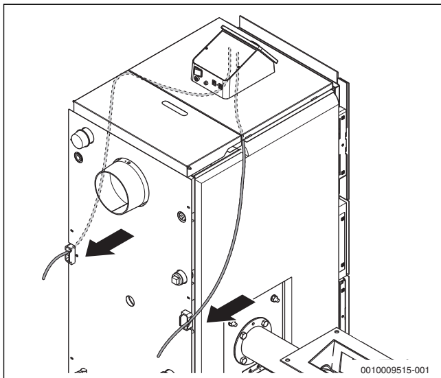
Obr. 28 Protahení kabelu kabelovým držákem
