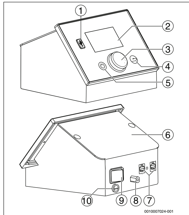
Obr. 22 Popis regulačního přístroje
