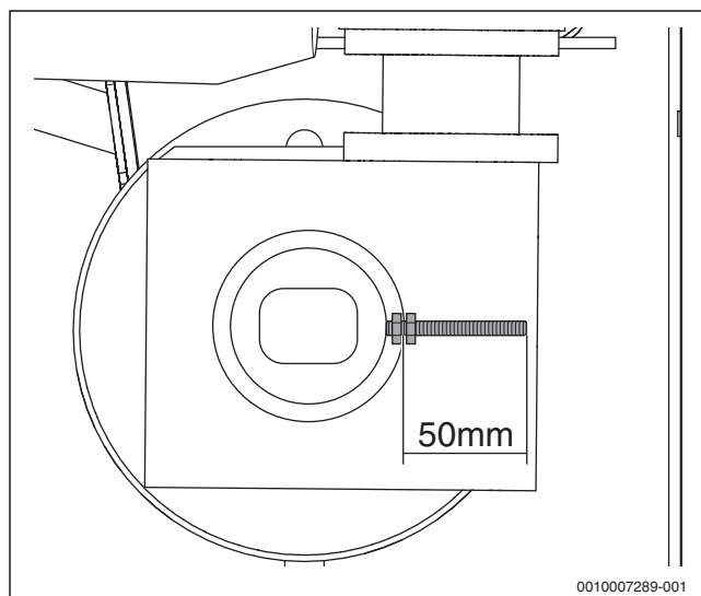
Obr. 43 Nastavení čidla šnekového dopravníku
