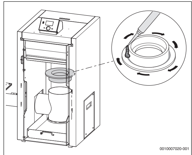
Obr. 45 Zatmelení spalovacího roštu
