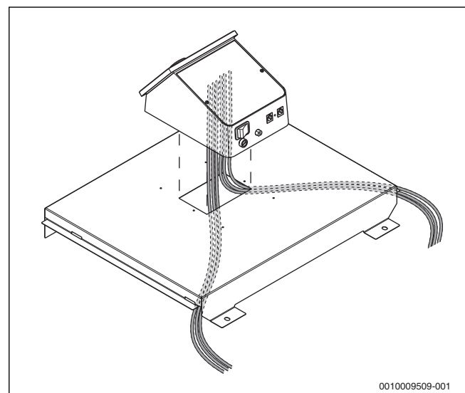
Obr. 23 Protažení kabelu a kabelu čidla krytem kotle
