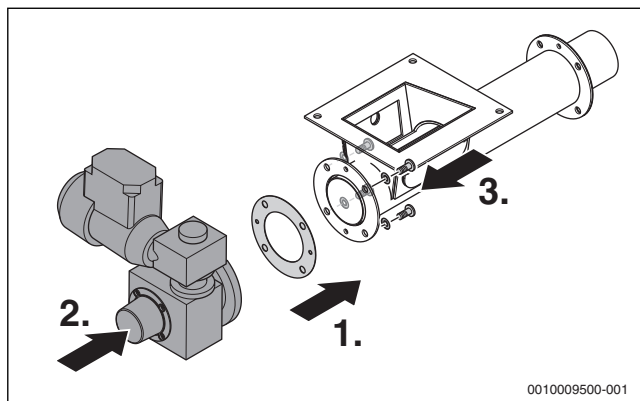
Obr. 14 Vložení těsnicího kroužku
