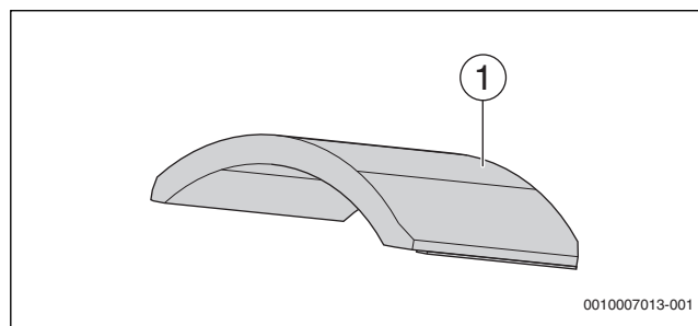
Obr. 2 Vestavné části spalovacího prostoru pro velikost kotle 15 kW
