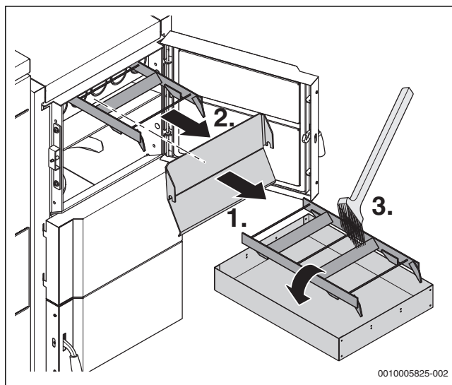
Obr. 62 Čištění turbulátoru
