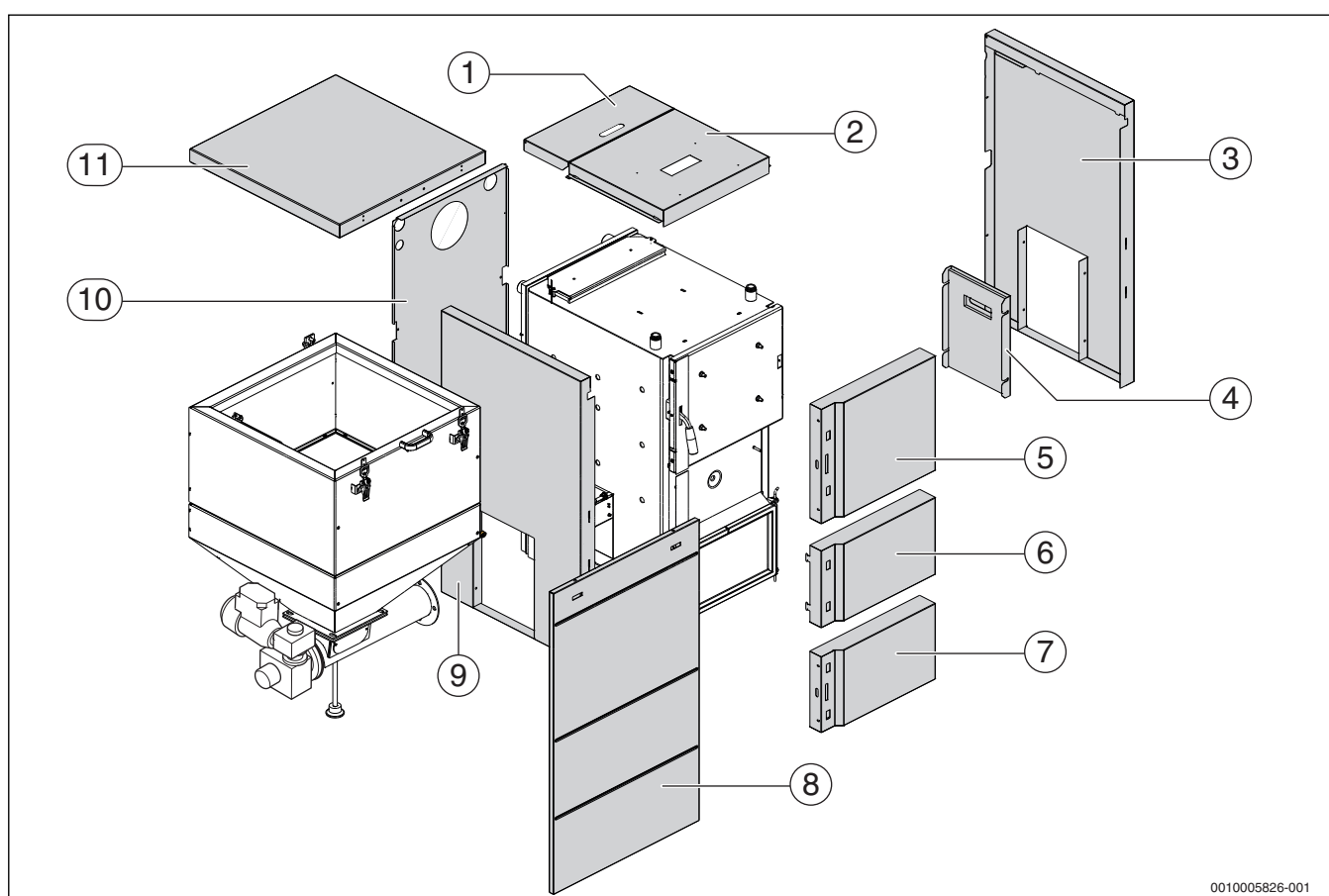
Obr. 10 Opláštění kotle
