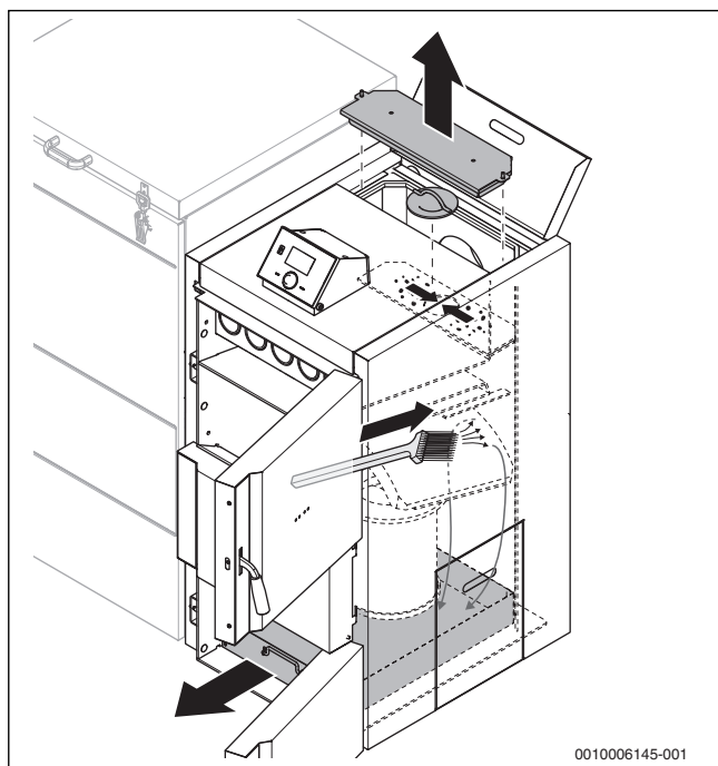
Obr. 64 Čištění cihel spalovacího prostoru
