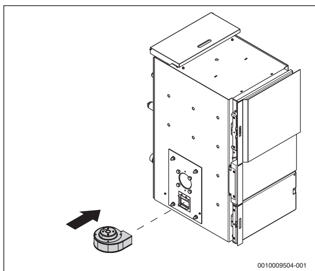
Obr. 18 Montáž ventilátoru
