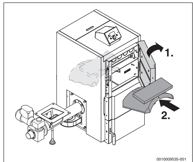
Obr. 46 Vložení cihel spalovacího prostoru
