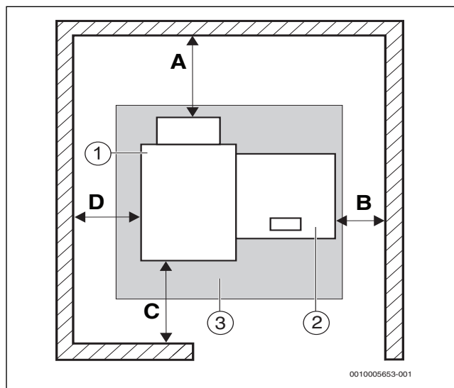
Obr. 8 Minimální odstupy od stěn
