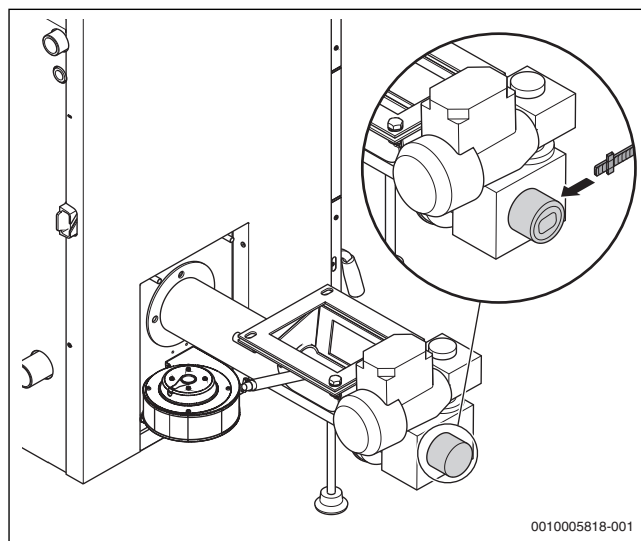
Obr. 42 Připojení čidla šnekového dopravníku
