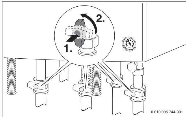
Obr. 2 Otevření servisních kohoutů
