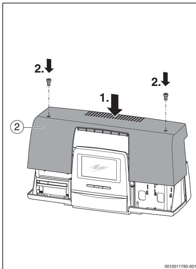
Obr. 40 Namontování ochranného krytu na regulační přístroj
