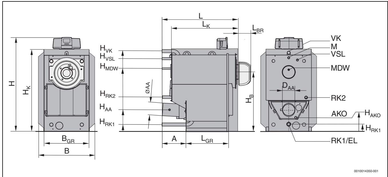
Obr. 3 Přípojky a rozměry
