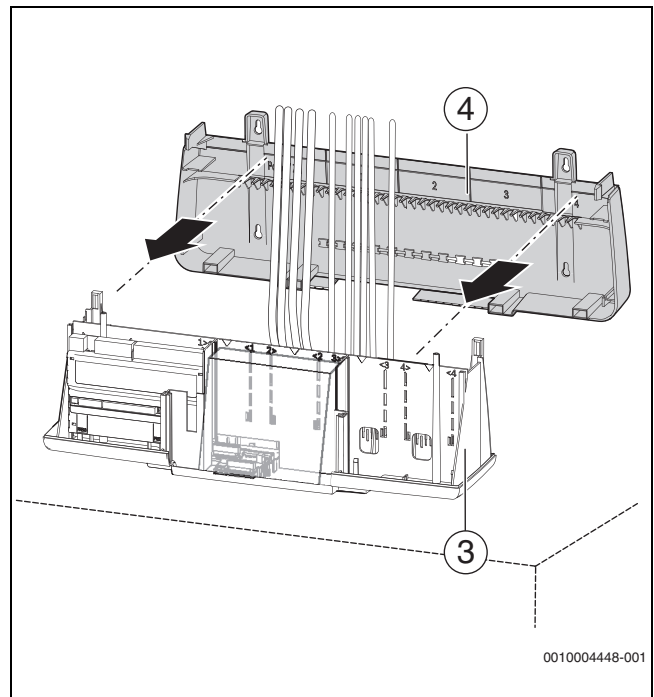
Obr. 35 Montáž na kotel, nasazení a zaklesnutí zadní stěny
