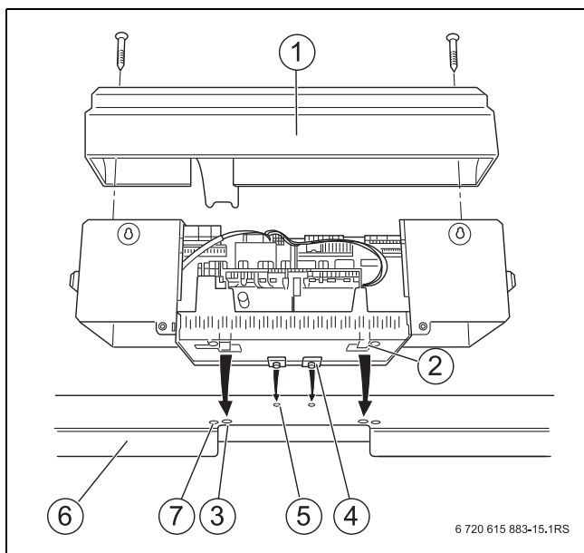
Obr. 29 Montáž regulačního přístroje
