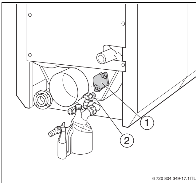
Obr. 44 Víčko čistícího otvoru sběrače spalin
