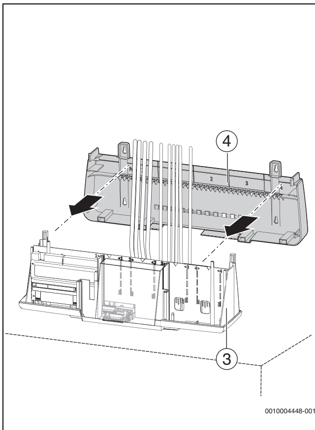
Obr. 37 Připevnění zadní stěny na spodní díl skříně
