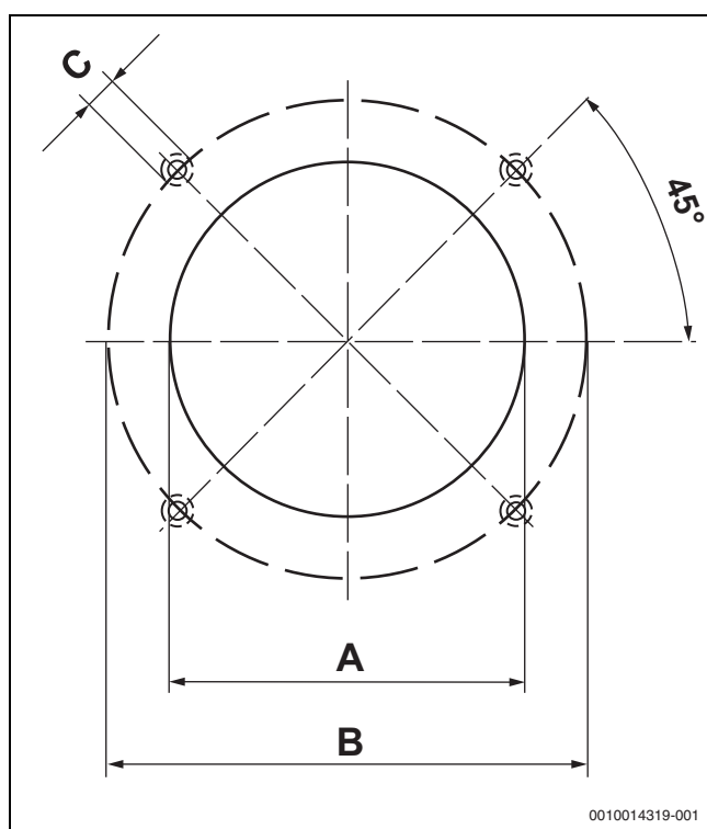
Obr. 24 Připojovací rozměry ve dvířkách spalovacího prostoru
