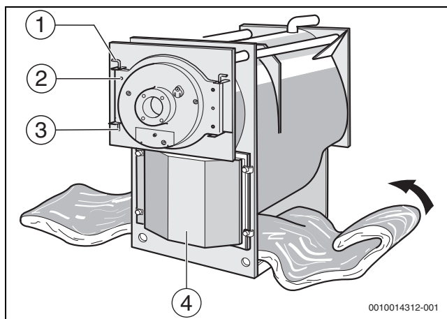
Obr. 9 Protáhnutí tepelněizolační rohože pod kotlem
