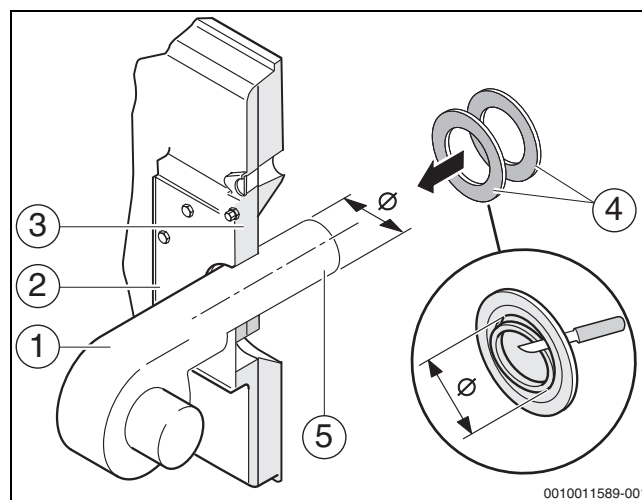
Obr. 25 Montáž hořáku
