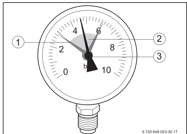
Obr. 45 Tlakoměr pro uzavřené otopné soustavy
