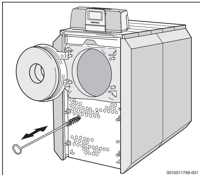
Obr. 43 Čištění kotle štětkou
