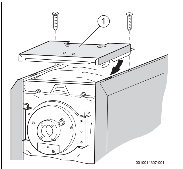
Obr. 21 Montáž předního krytu kotle
