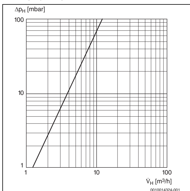
Obr. 47 Průtokový odpor vody
