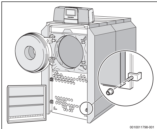
Obr. 42 Sejmutí usměrňovací krytu a otevření dvířek spalovacího prostoru
