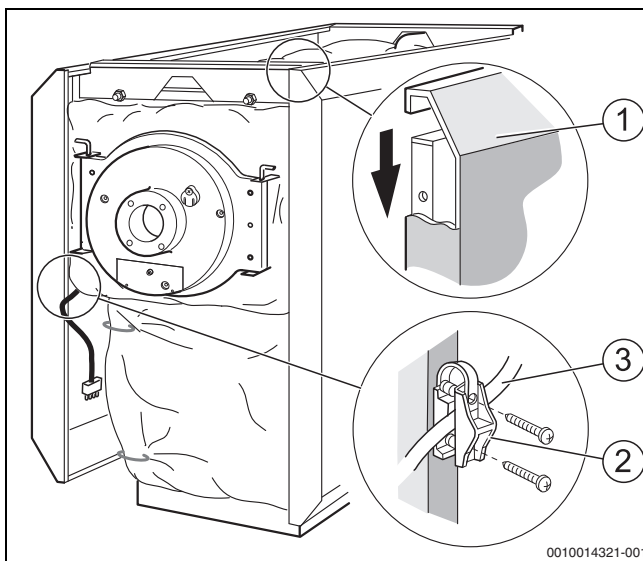
Obr. 19 Zavěšení bočních stěn a připevnění kabelu hořáku
