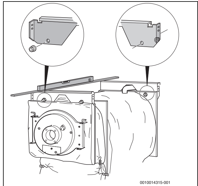
Obr. 16 Nasazení a přišroubování přední a zadní traverzy
