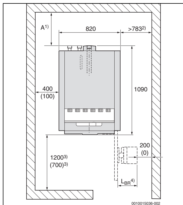
Obr. 7 Rozměry místa instalace v mm → tab. 10, str. 16 (hodnoty v závorkách jsou minimální odstupy)
