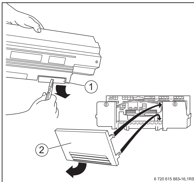
Obr. 30 Příprava kabelového průchodu
