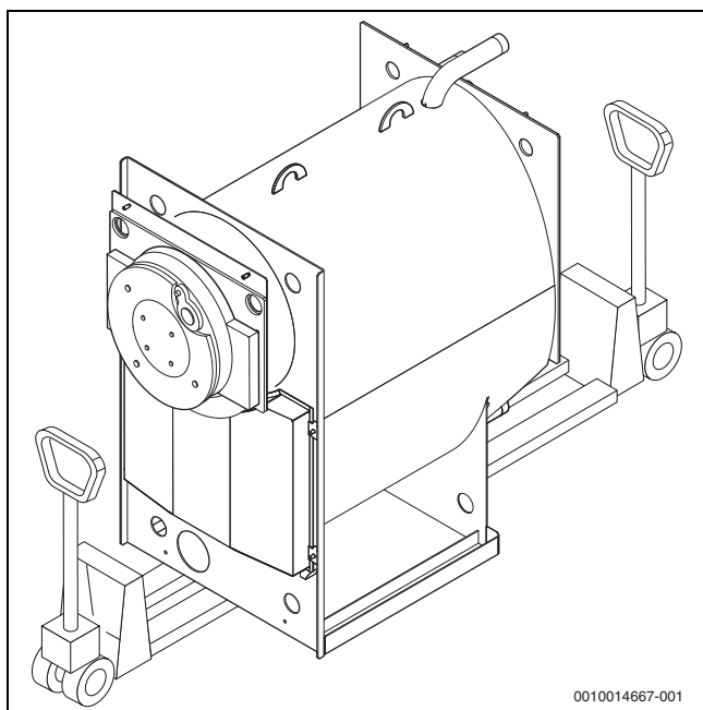
Obr. 6 Přeprava kotle 2 nízkozdvížnými vozíky
