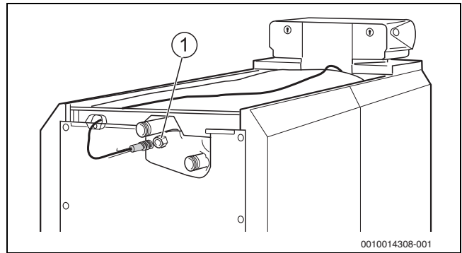
Obr. 27 Zavedení teplotních čidel do jímky
