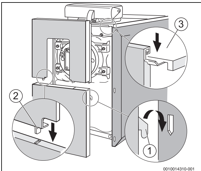
Obr. 22 Připevnění horní a dolní přední stěny
