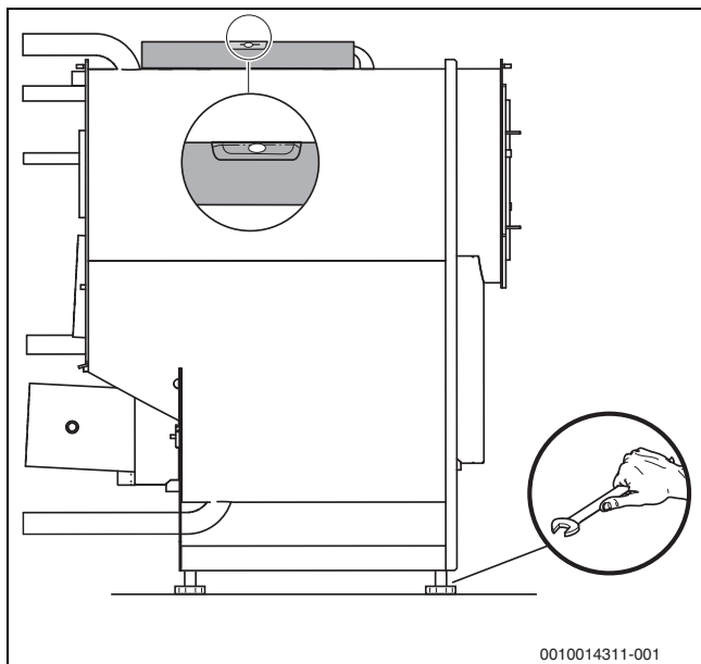
Obr. 8 Vyrovnání kotle
