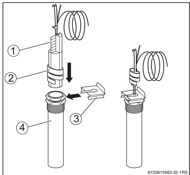
Obr. 28 Vložení plastové spirály do jímky
