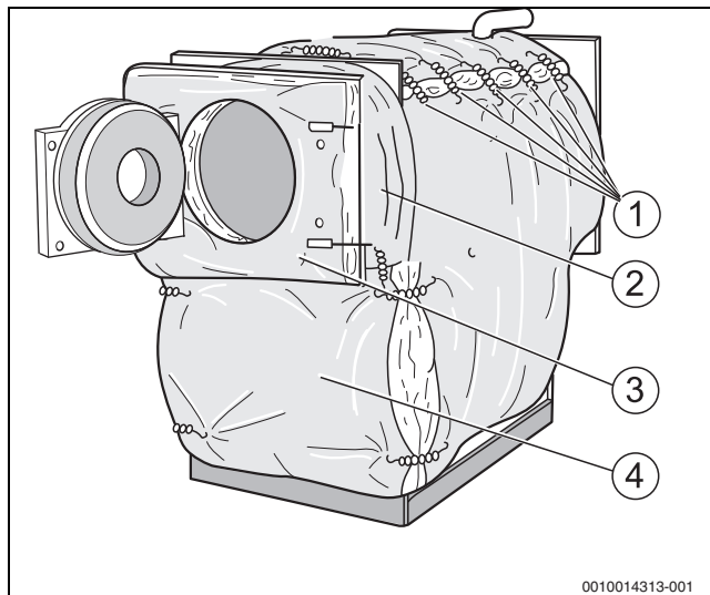
Obr. 10 Přiložení a upevnění tepelné izolace
