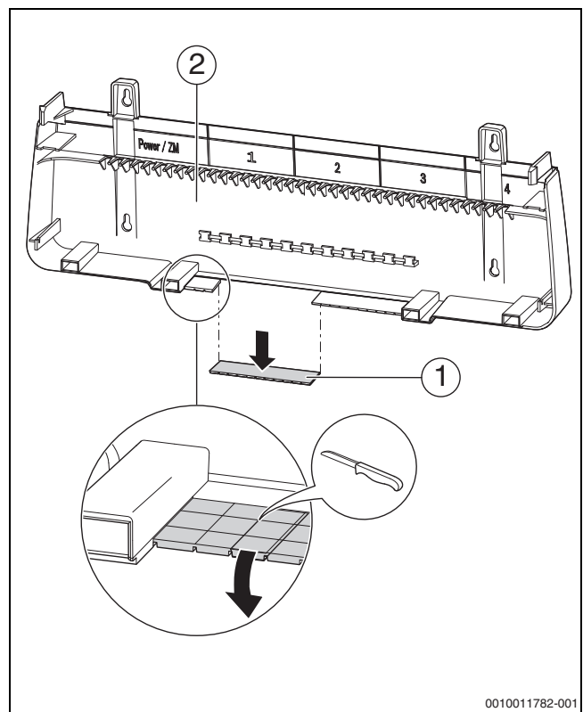
Obr. 36 Příprava kabelového průchodu
