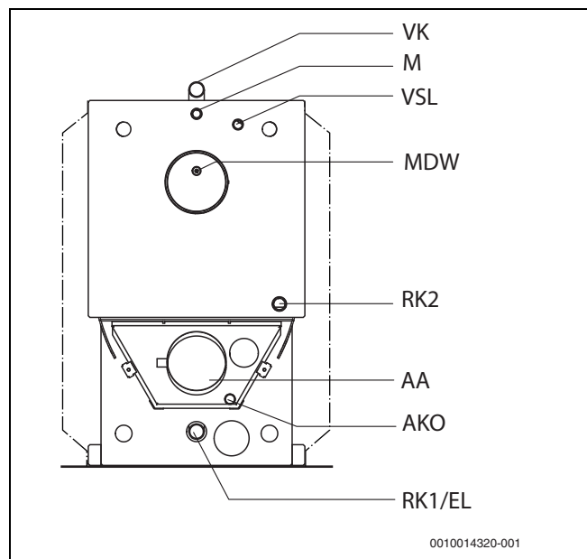
Obr. 12 Připojky kotle
