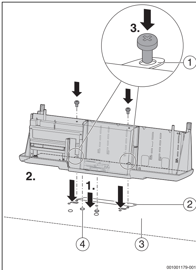
Obr. 33 Montáž regulačního přístroje
