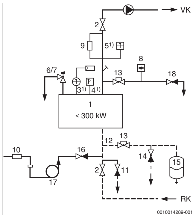
Obr. 46 Bezpečnostní výbava podle EN 12828:2012 pro kotle \leq 300 kW s havarijním termostatem (STB) \leq 110 °C
