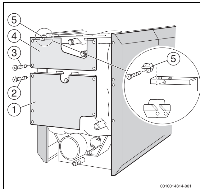
Obr. 20 Přišroubování 2dílné zadní stěny
