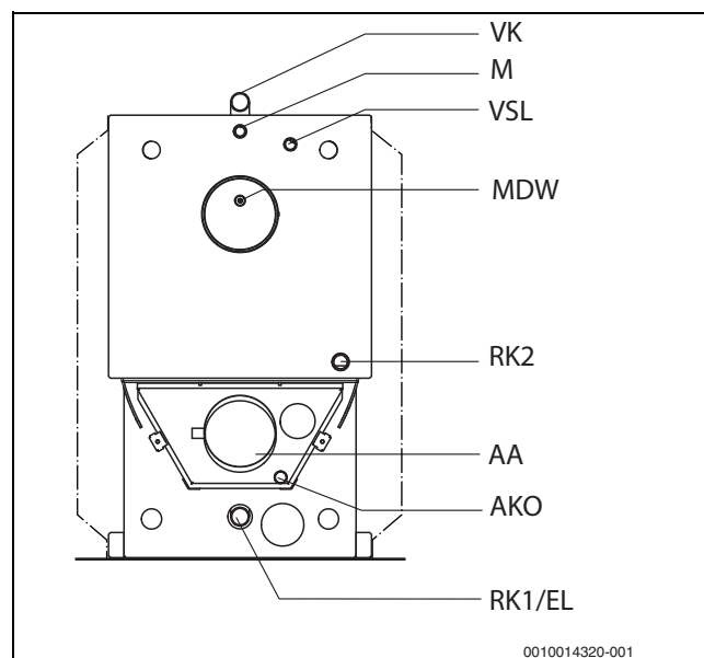
Obr. 15 Připojky na kotli Logano plus SB325
