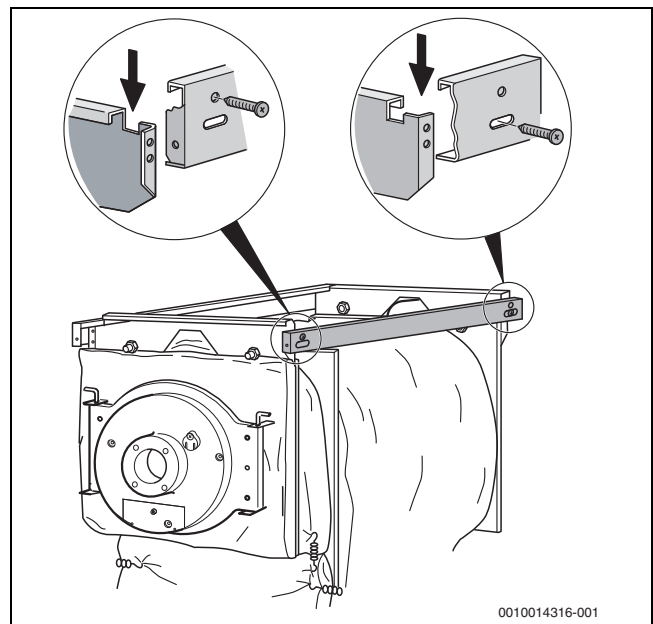
Obr. 17 Zavěšení a našroubování bočních traverz
