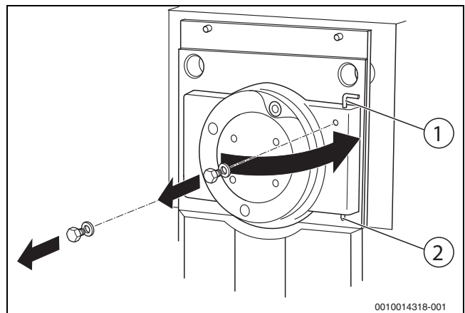
Obr. 23 Otevření dvířek spalovací komory
