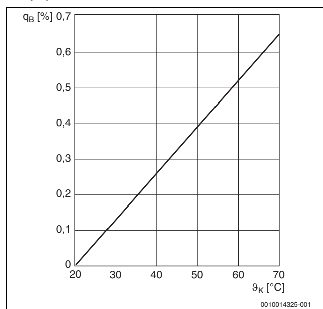
Obr. 48 Ztráty v pohotovostním režimu v závislosti na střední teplotě kotlové vody
