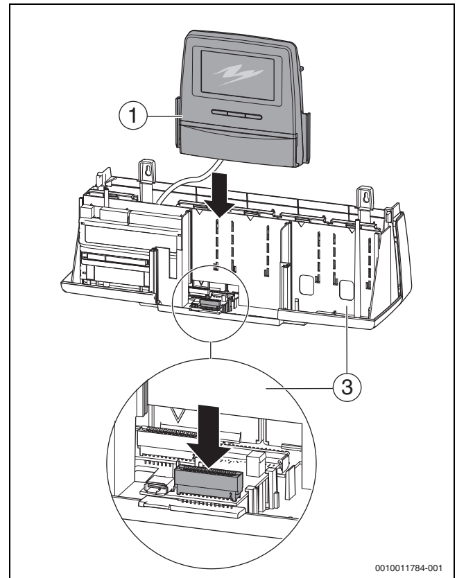
Obr. 39 Nasazení obslužné regulační jednotky na spodní díl skříně
