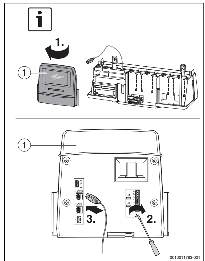
Obr. 38 Nastavení adresy řídicí jednotky
