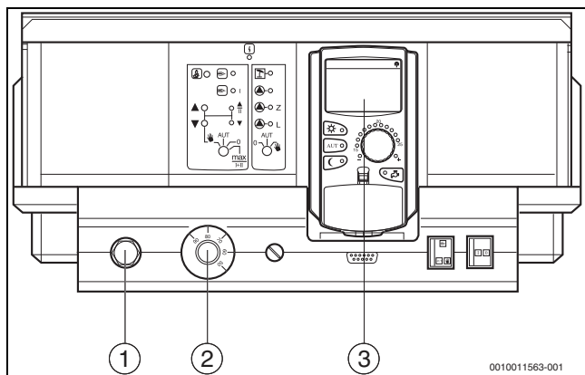
Obr. 32 Nastavení na řídicí jednotce
