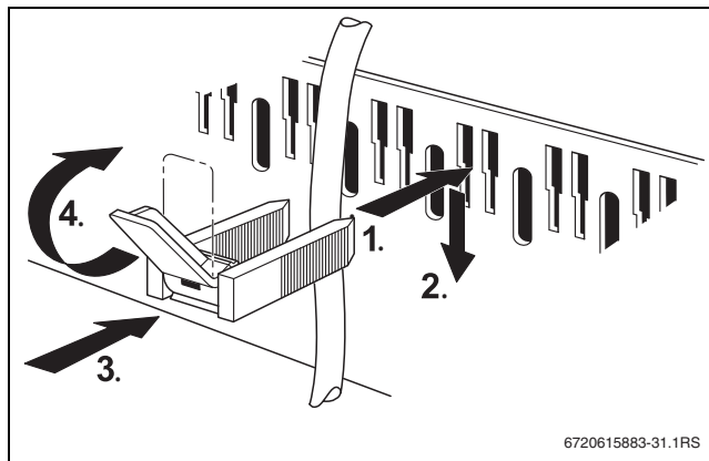
Obr. 31 Zajištění kabelu kabelovou sponou
