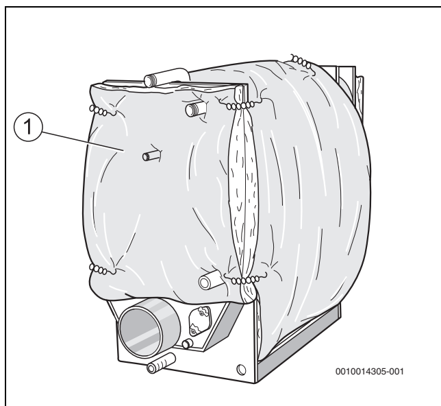
Obr. 11 Přiložení a upevnění tepelné izolace zadního panelu
