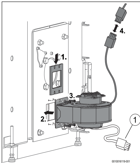
Obr. 1 Montáž ventilátoru
