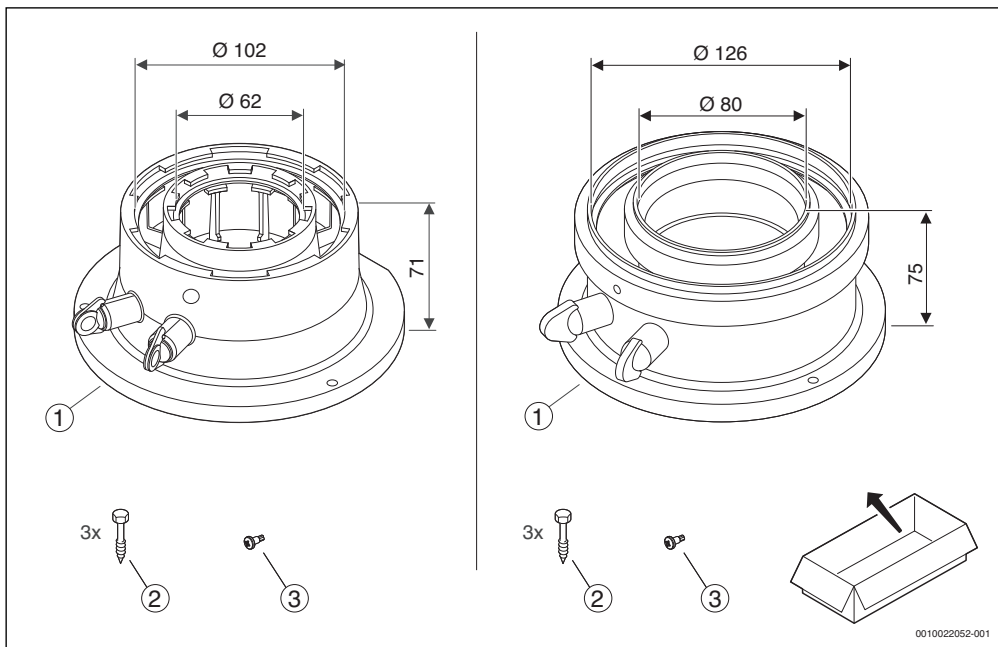
1 \text{Ø } 60/100 : 7738112636, \text{Ø } 80/125 : 7738112714
