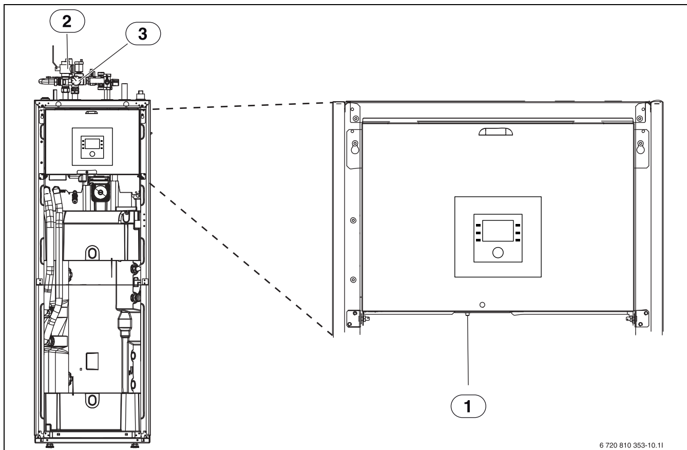
Obr. 5 Vnitřní jednotka AWMS / AWMSS
