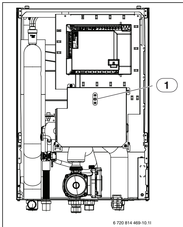
Obr. 6 Vnitřní jednotka IDUS E
