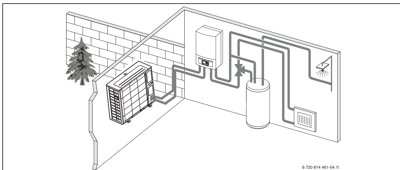
Obr. 2 Tepelné čerpadlo s venkovní jednotkou, vnitřní jednotkou IDUS E s elektrickou pomocnou topnou tyčí, s externím zásobníkem teplé vody
