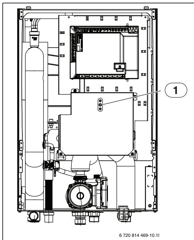
Obr. 6 Vnitřní jednotka AWES
