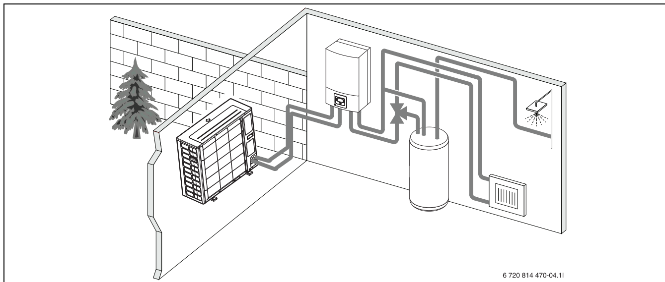
Obr. 2 Tepelné čerpadlo s venkovní jednotkou, vnitřní jednotkou AWES s elektrickou pomocnou topnou tyčí, s externím zásobníkem teplé vody
