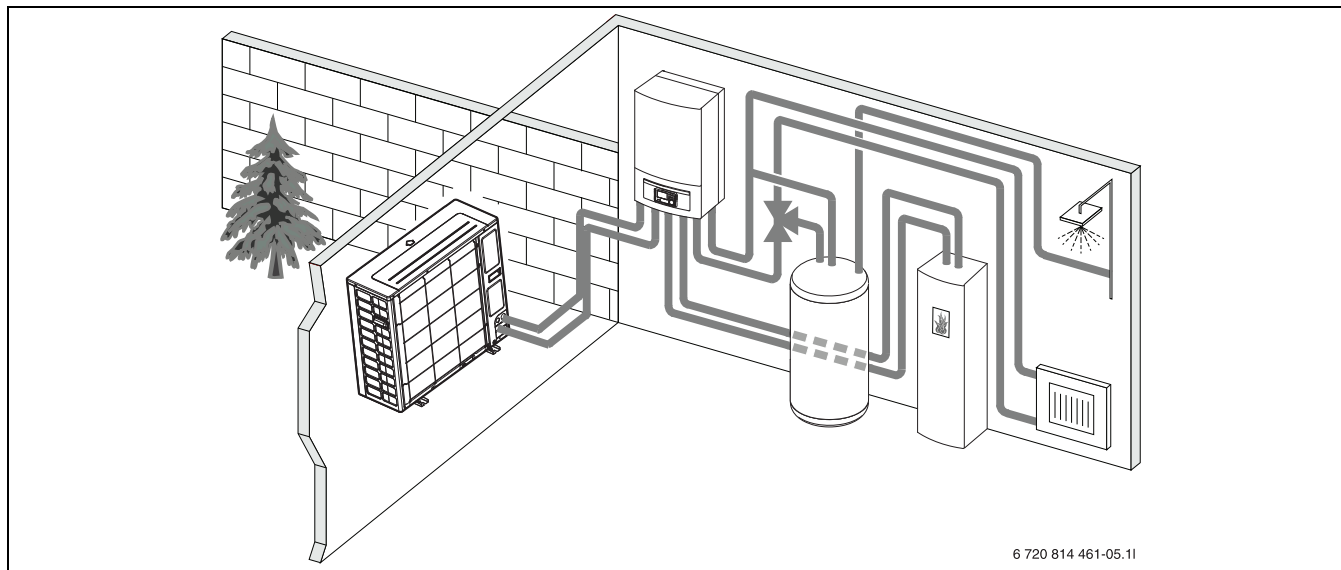
Obr. 2 Tepelné čerpadlo, venkovní jednotka, vnitřní jednotka IDUS B bez elektrické pomocné topné tyče, externí zásobník teplé vody a externí dohřev
