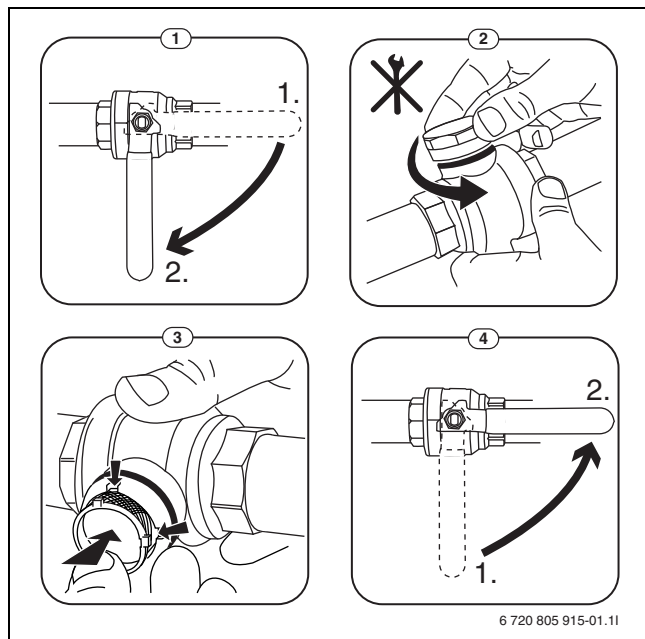
Obr. 6 Čištění sítka
