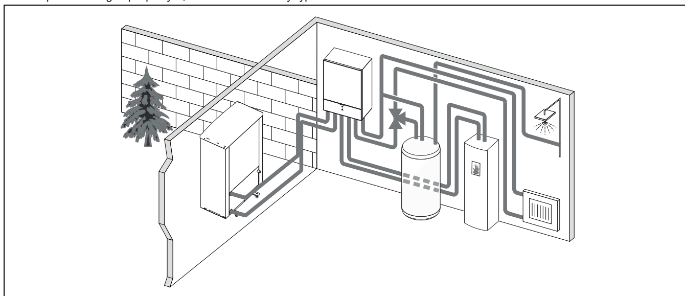
Obr. 3 Tepelné čerpadlo WLW196i.2 AR/IR, vnitřní jednotka IDU-..iB bez elektrické pomocné topné tyče, externí zásobník teplé vody a externí dohřev
