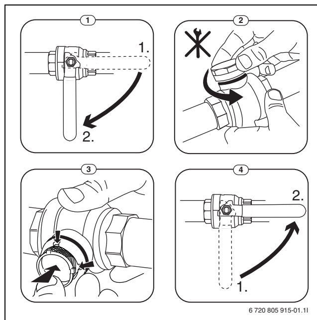
Obr. 8 Čištění sítka
