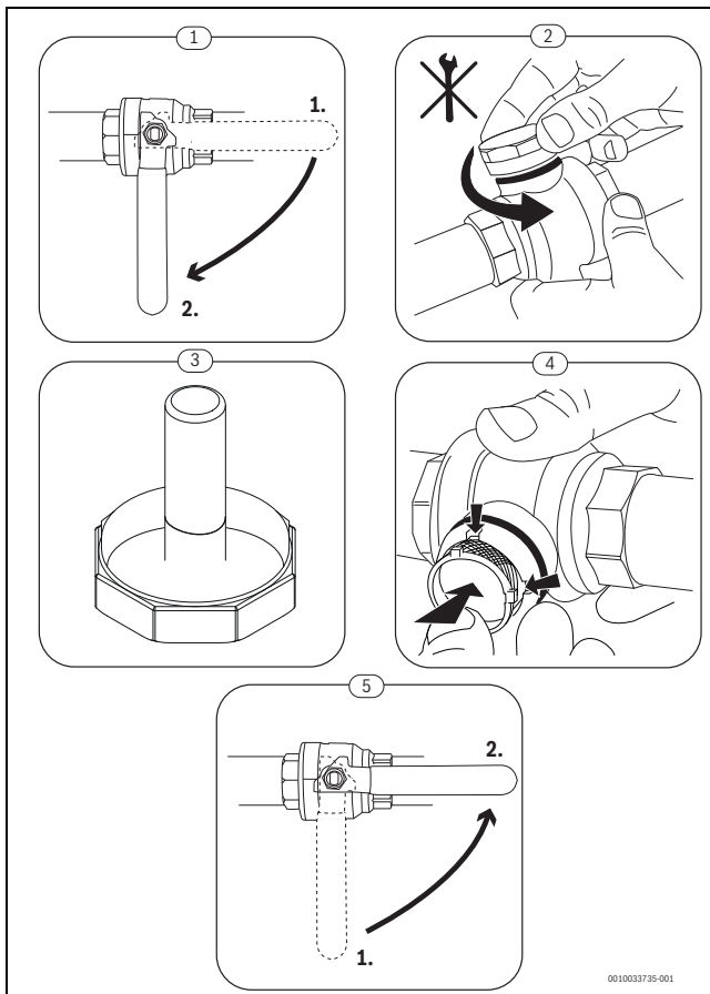
Obr. 20 Čištění sítka
