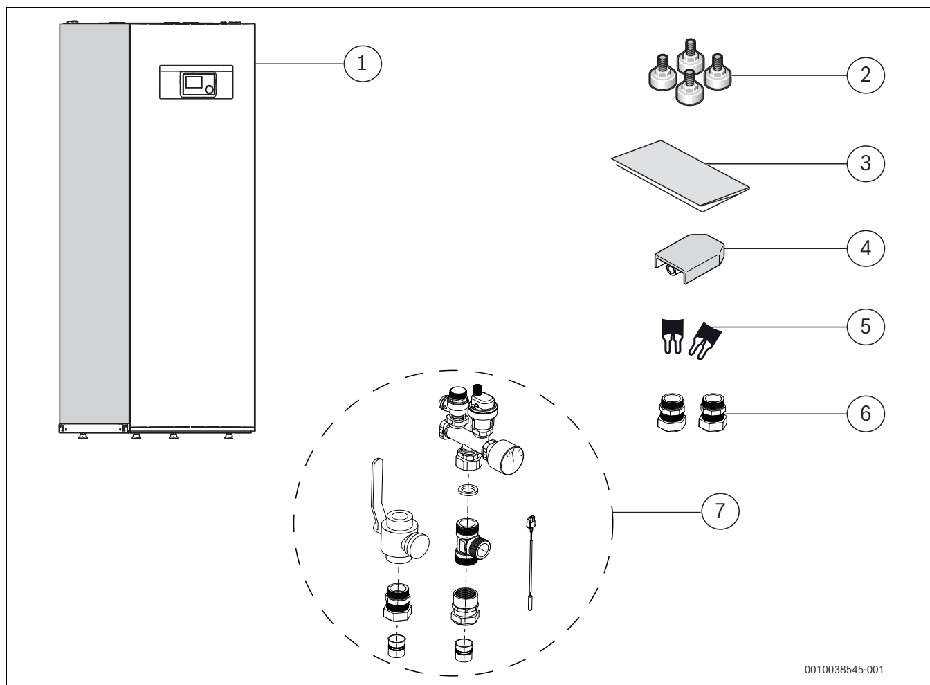
Obr. 2 Rozsah dodávky
