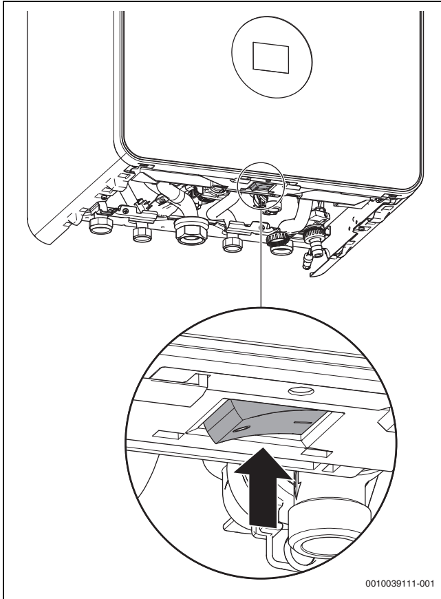
Obr. 1 Hlavní vypínač
