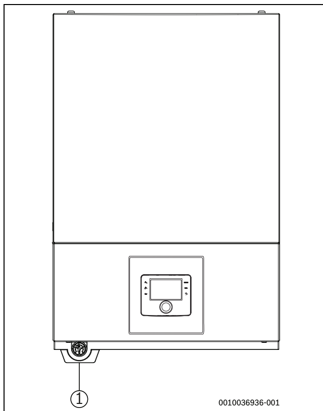
Obr. 5 Vnitřní jednotku AWS E (zobrazení s odkapávacím zásobníkem)
