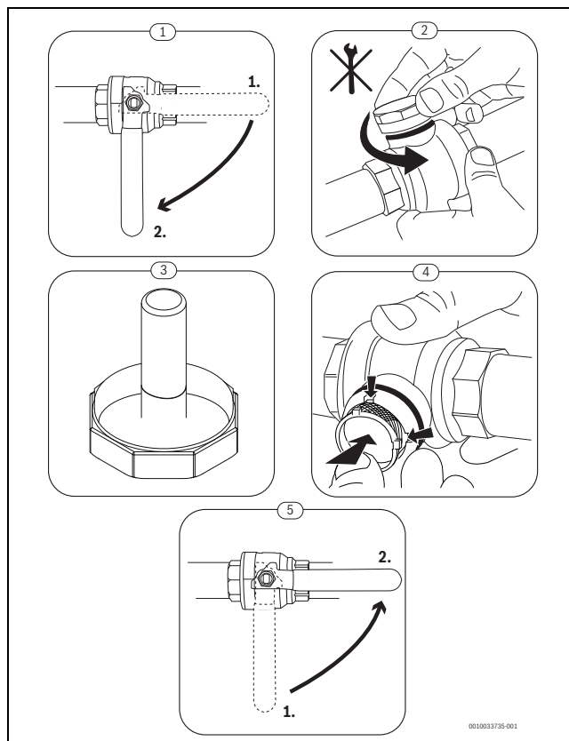
Obr. 6 Čištění sítka
