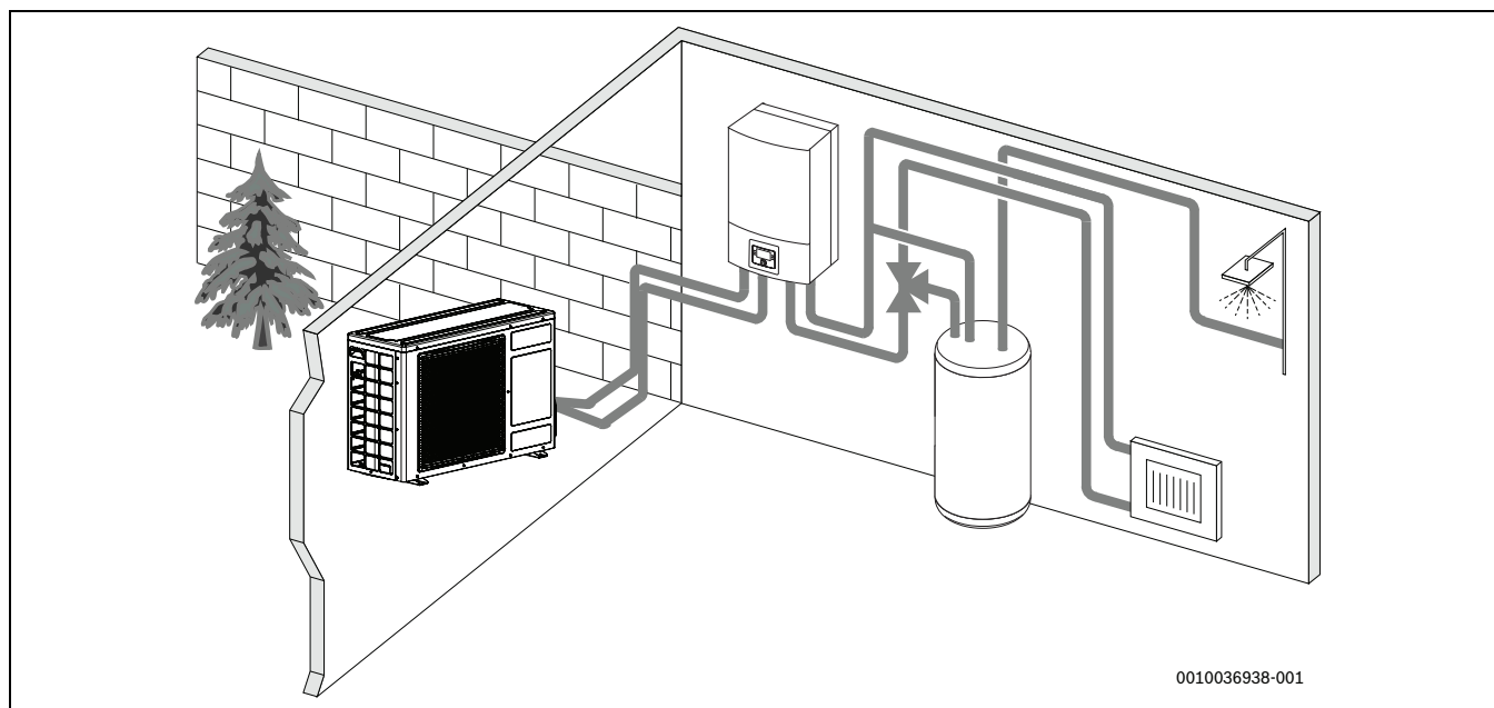
Obr. 2 Venkovní jednotka tepelného čerpadla, vnitřní jednotka AWS E s elektrickou pomocnou topnou tyčí a externím zařízením na přípravu teplé vody
