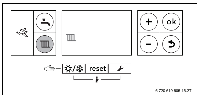
Obr. 4 Displej Vytápění
