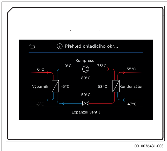
Obr. 9 Přehled chladicího okruhu
