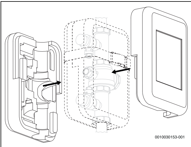
Obr. 55 Izolace plnicího zařízení
