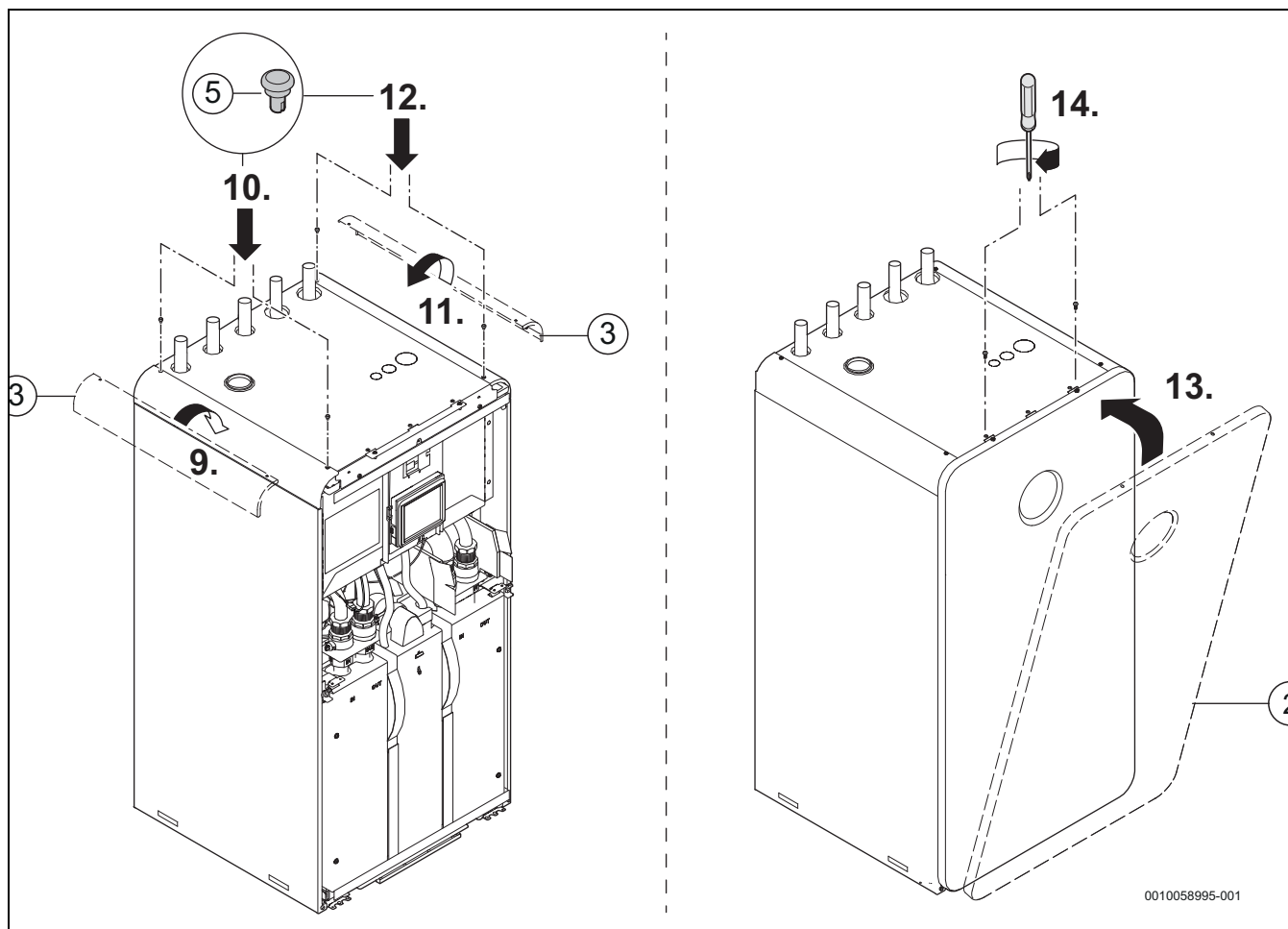
Obr. 8 Sestava designové sady
