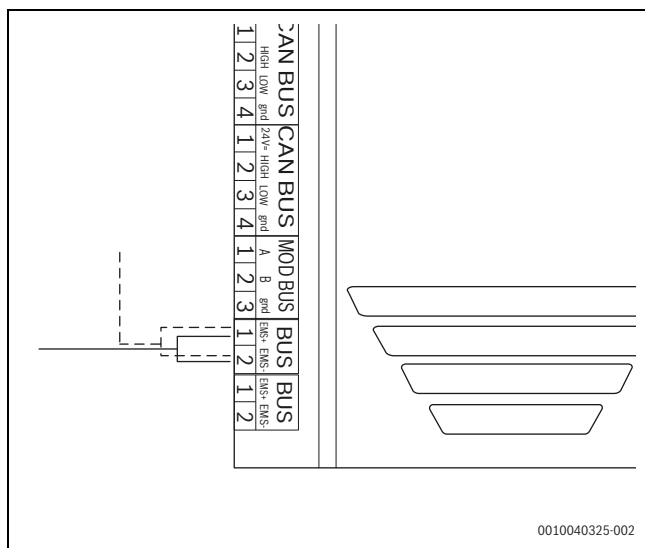
Obr. 64 Připojení EMS
