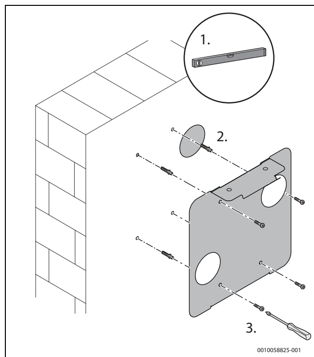
Obr. 33 Namontujte konzolu
