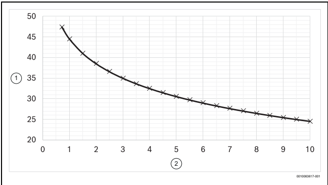
Obr. 28 Úroveň nepřetržitého akustického tlaku vyjádřená jako energetický ekvivalent ( L_p(r, Q=4) ) pro výstup potrubí evakuačního ventilátoru umístěného venku, v závislosti na vzdálenosti od výstupu potrubí k místu imise (místu posuzování). Celková doba měření činí 8 hodin a graf
