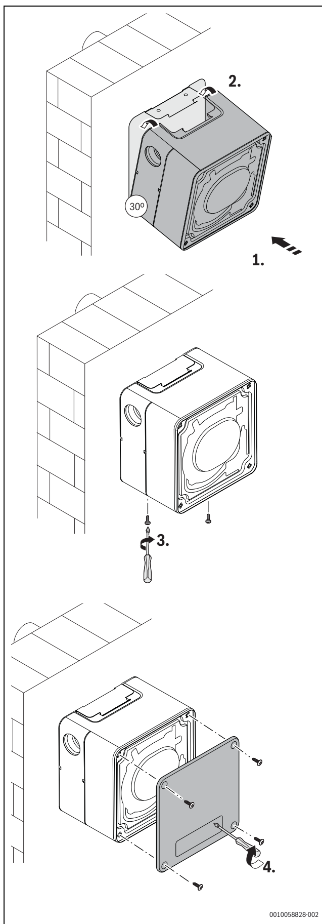
Obr. 42 Jak zavřít skříň ventilátoru
