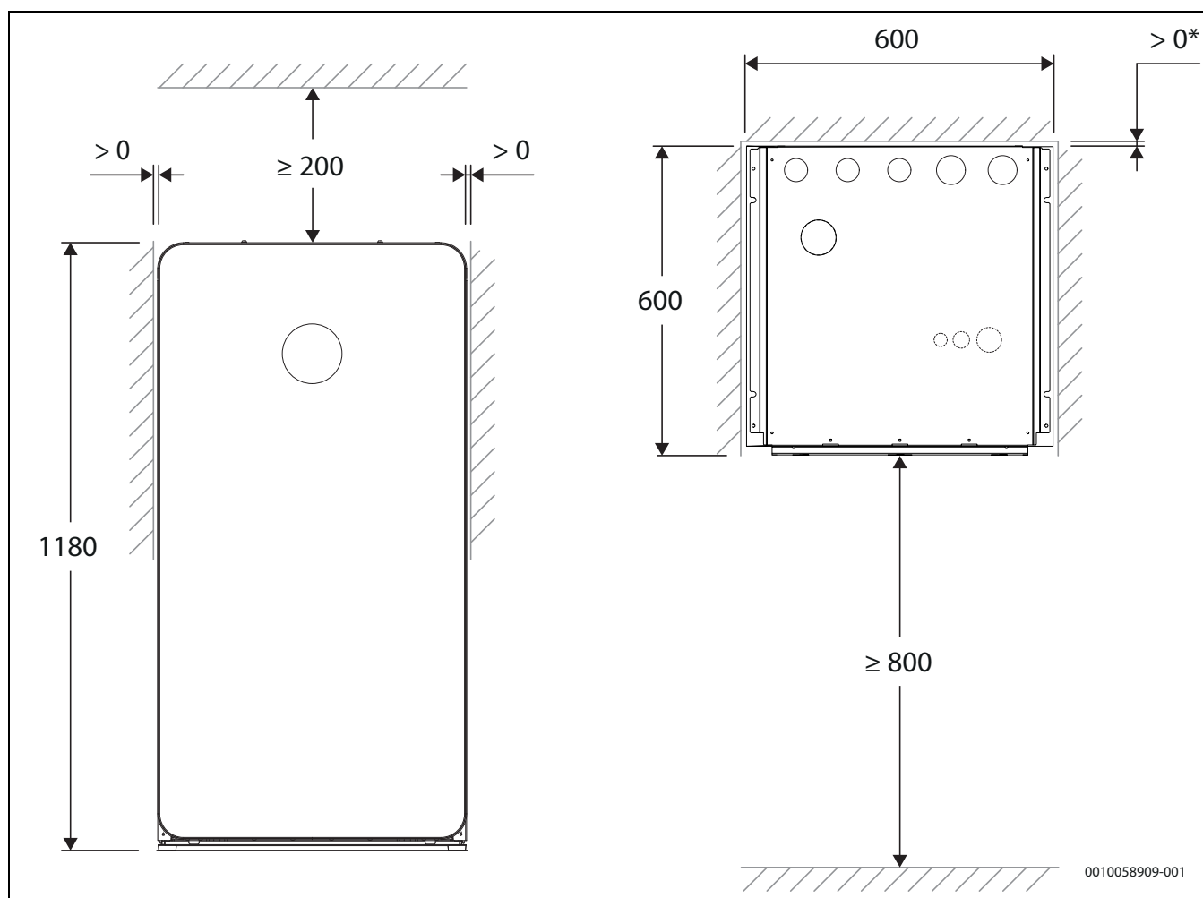
Obr. 2 Rozměry a minimální vzdálenosti
