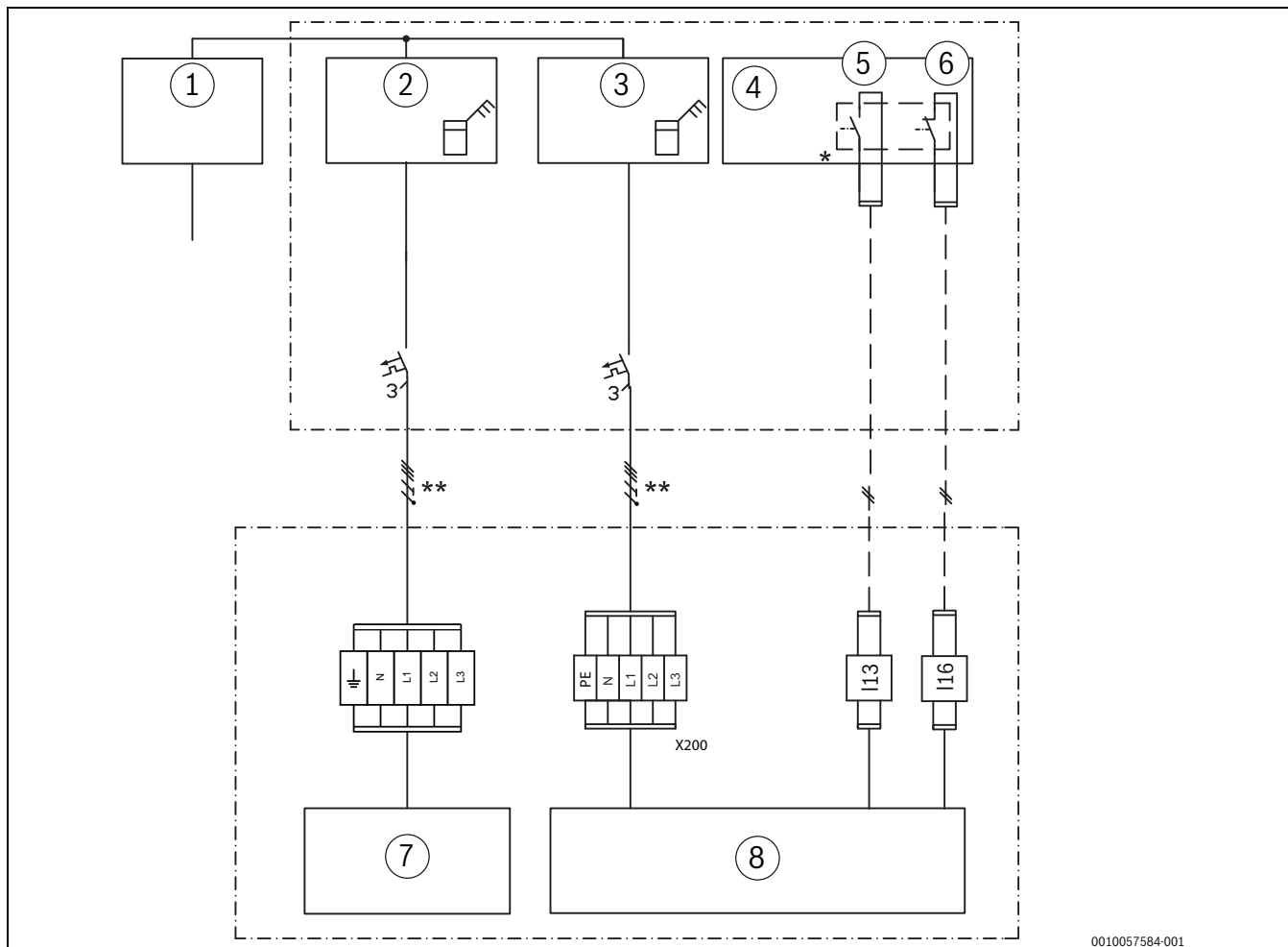
Obr. 65 Doporučené řešení
