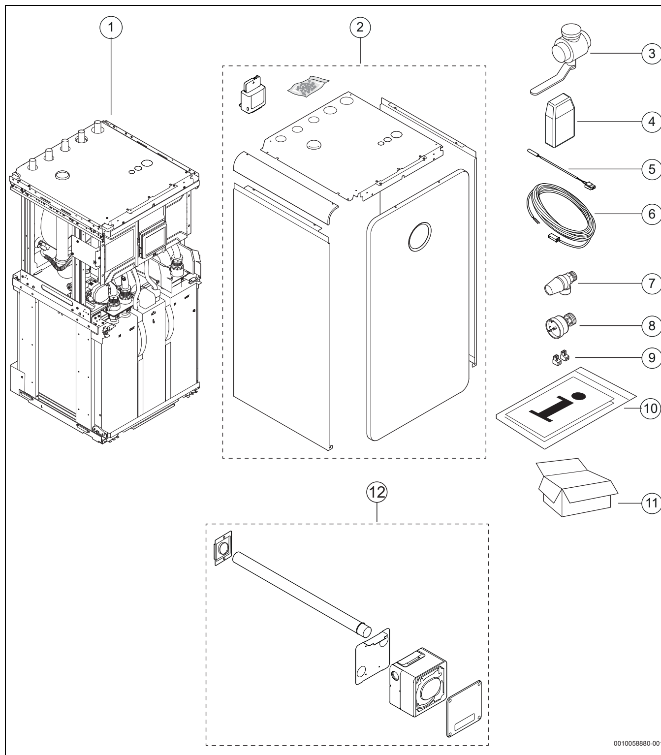
Obr. 1 Rozsah dodávky
