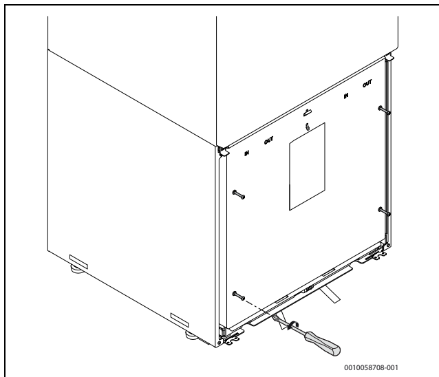
Obr. 17 Povolte 4 šrouby
