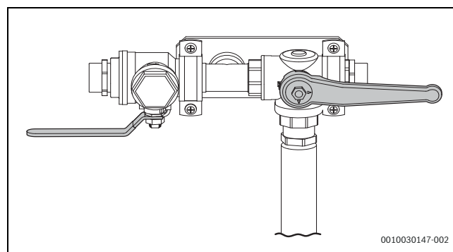
Obr. 52 Plnicí stanice v plnicí poloze
