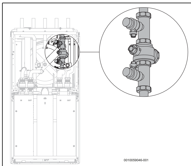
Obr. 48 Plnicí skupina
