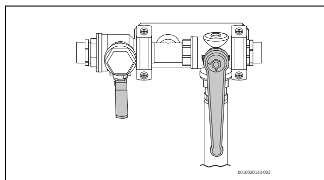
Obr. 51 Plnicí stanice ve směšovací poloze
