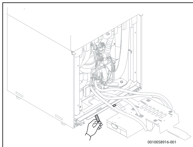
Obr. 21 Odstraňte označovací pásky
