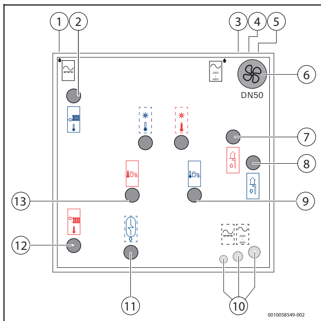
Afb. 5 Warmtepompaansluitingen, bovenaanzicht
