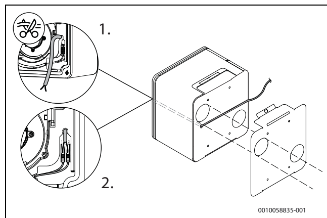
Afb. 42 Hoe de kabels in de ventilatorunit geleiden
