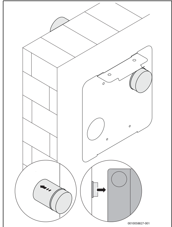
Afb. 36 Stop de schacht in de wand
