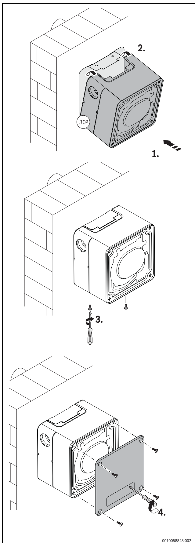
Afb. 43 Hoe de ventilatorunit sluiten
