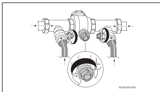
Afb. 51 Vulinrichting in vulstand
