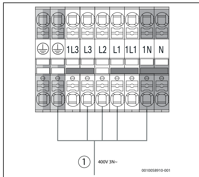
Afb. 59 Standaard voedingsaansluiting af fabriek ingesteld (6 kW, 8 kW, 13 kW, 17 kW)
