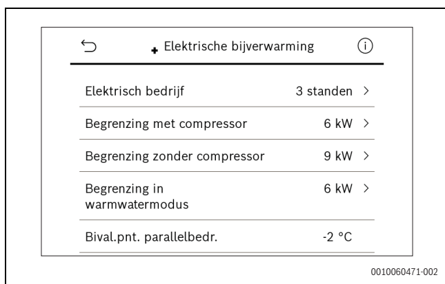
Afb. 66 Instellingen voor elektrische bijverwarming
