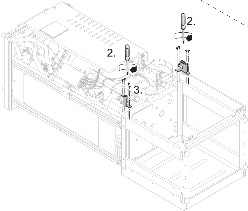
Afb. 15 Opsplitsen warmtepomp
