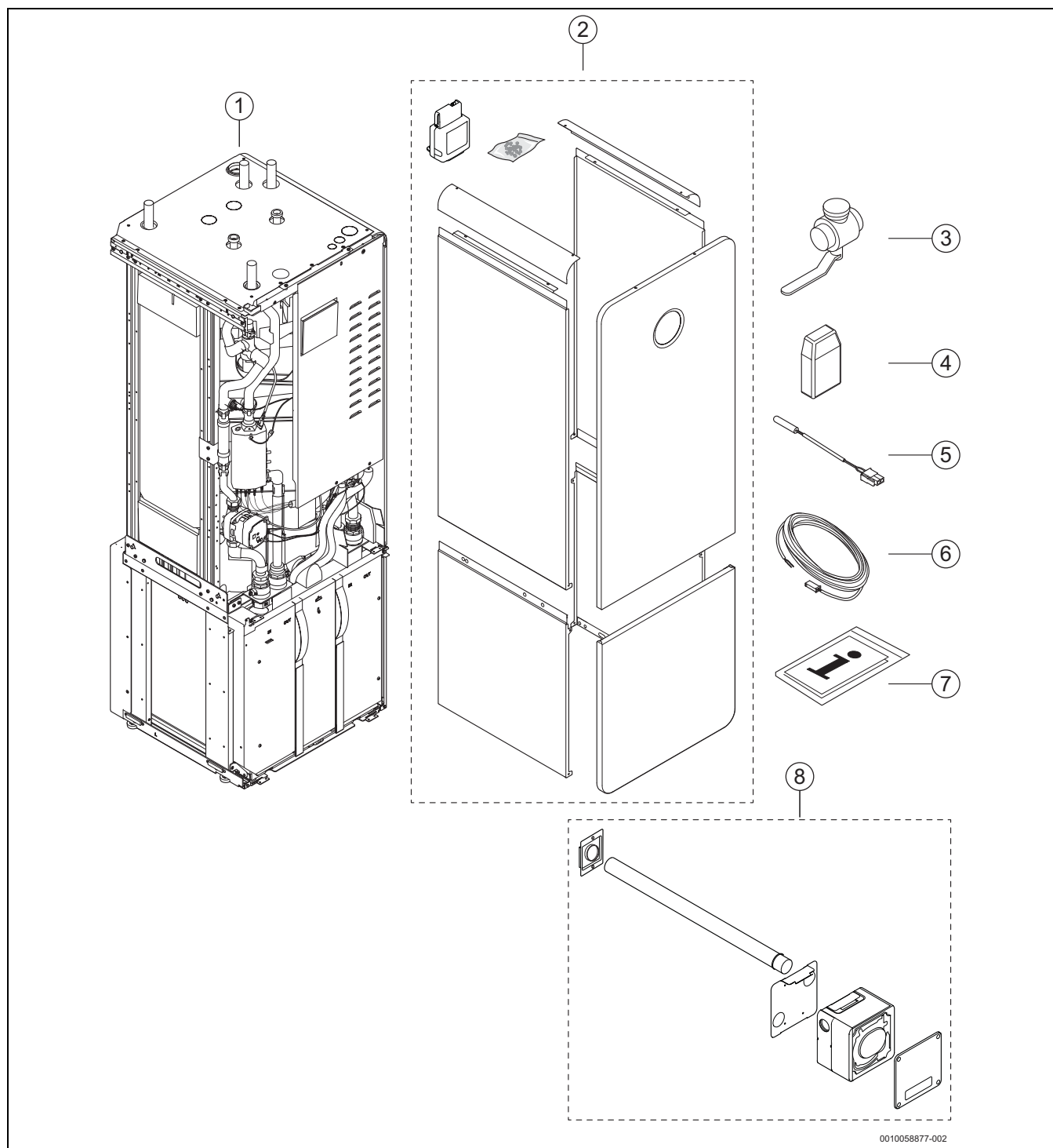
Afb. 1 Leveringsomvang
