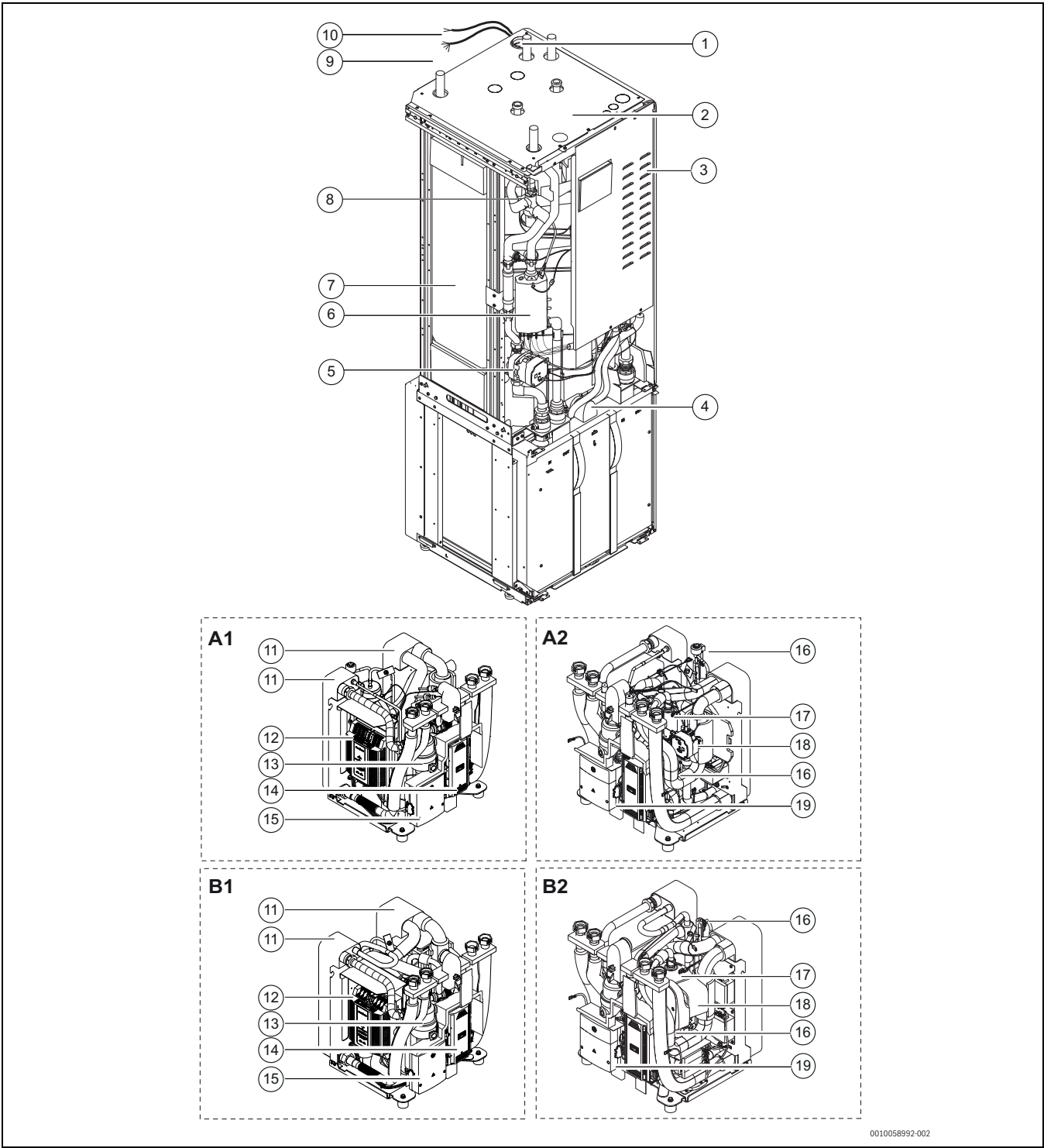
Afb. 4 Productoverzicht
