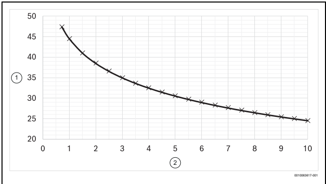
Afb. 29 Energie-equivalent continu geluidsdrukkniveau ( L_r(r, Q=4) ) voor de buiten geplaatste uitlaat van het afvoerkanaal van de afzuigventilator, als functie van de afstand van de uitlaat naar het immissiepunt (locatie van beoordeling). Totale beoordelingsperiode is 8 uur en de grafiek toont het gemiddelde geluidsdrukkniveau gedurende de hele beoordeling
