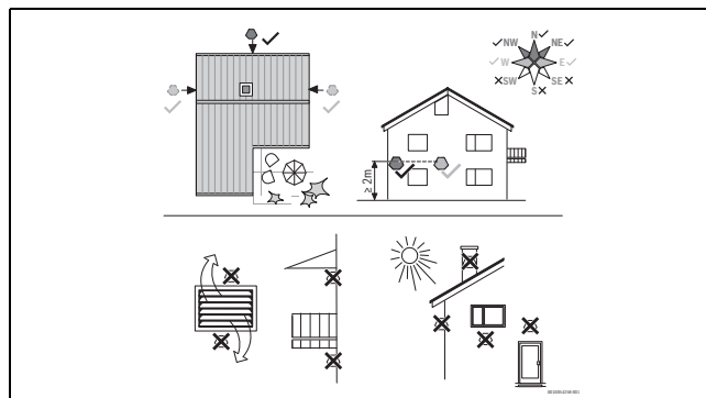
Afb. 63 Positie van de buitentemperatuursensor
