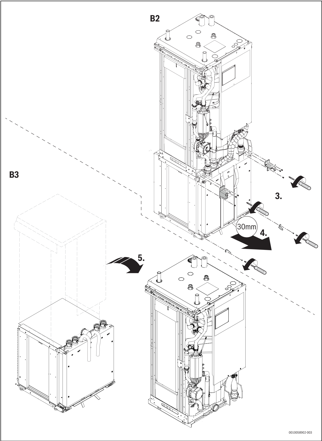
Afb. 13 Opsplitsen warmtepomp
