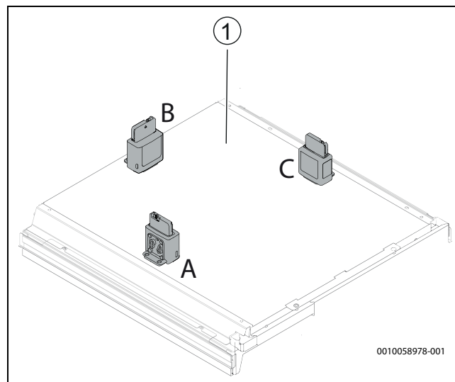
Afb. 28 Plaatsingsvoorbeeld van Connect-Key
