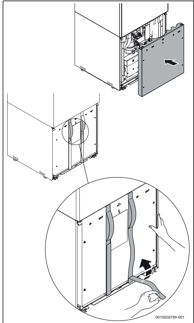
Afb. 26 Plaats het frontmantel terug.
