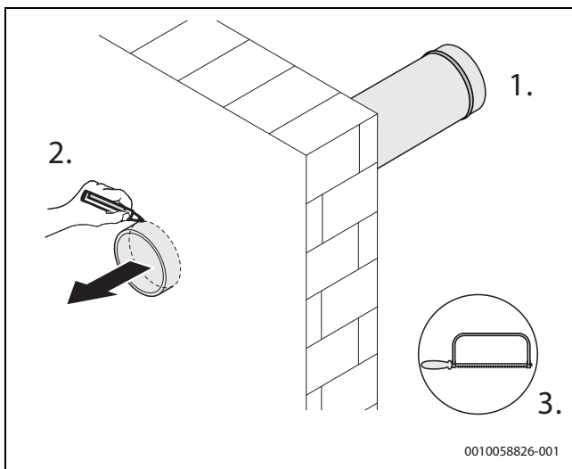
Afb. 35 Snijd de leiding door.
