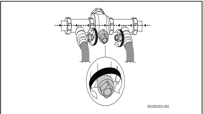
Afb. 55 Vulinrichting in de normale stand
