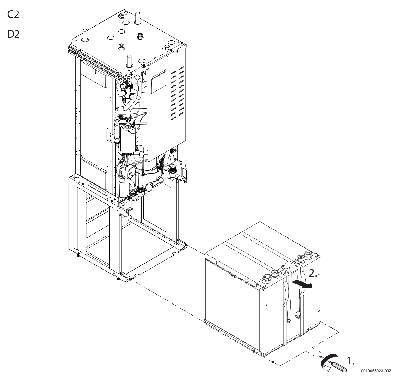
Afb. 14 Opsplitsen warmtepomp
