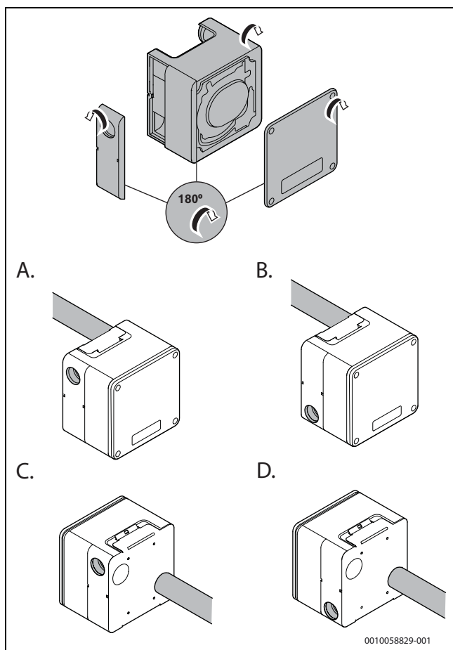
Afb. 32 Manieren om de ventilatorunit te monteren
