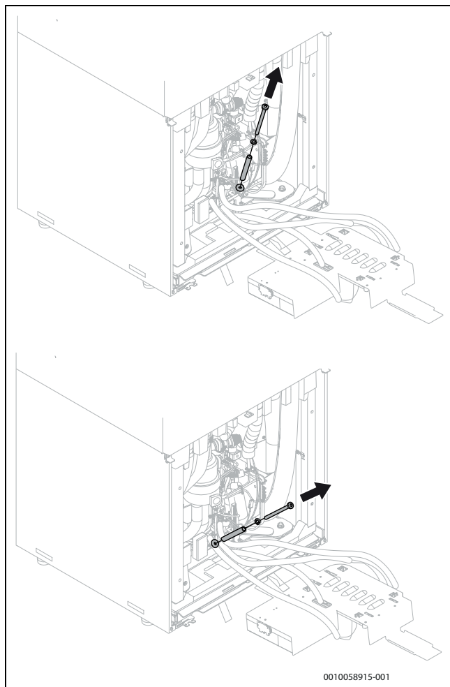
Afb. 21 Verwijder de schroeven die de beugel vasthouden.
