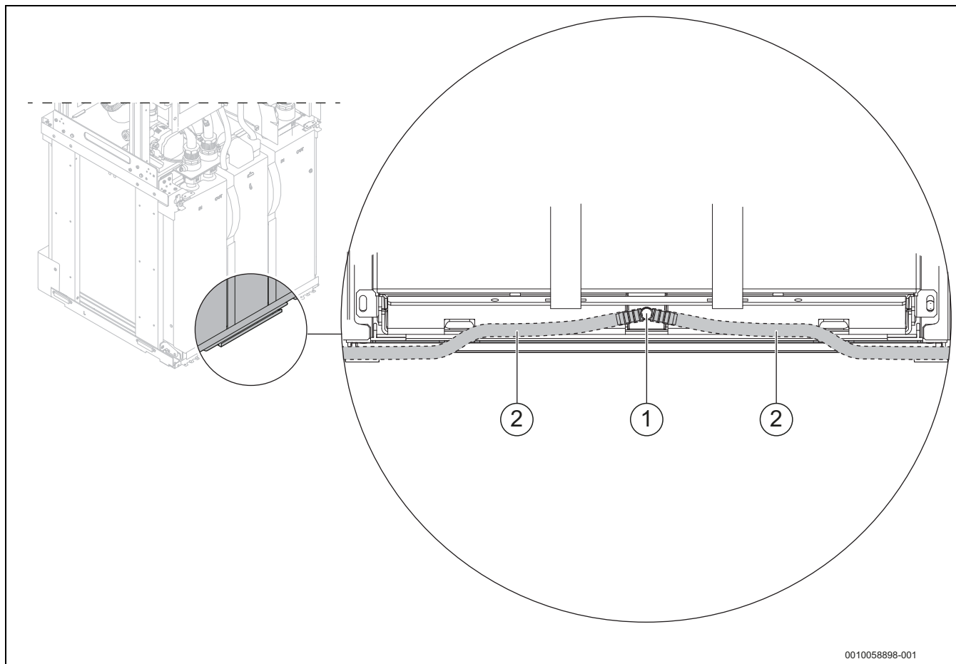
Afb. 45 Sluit de afvoerslang aan
