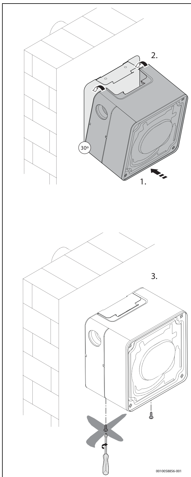
Afb. 38 Bevestig de ventilatorunit aan de console.
