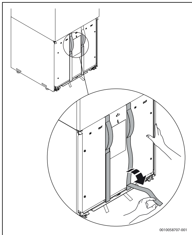
Afb. 17 Maak de banden los.
