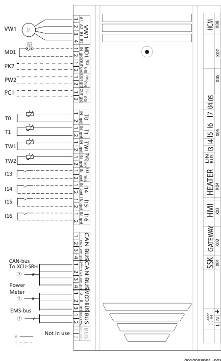
Afb. 61 Aansluitingen XCU-THH
