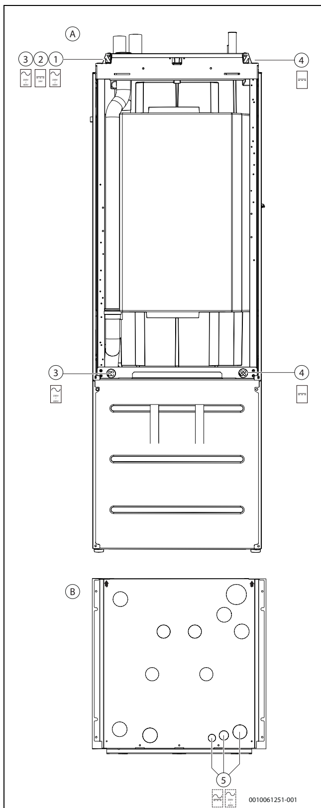
Afb. 58 Kabelinvoeren
