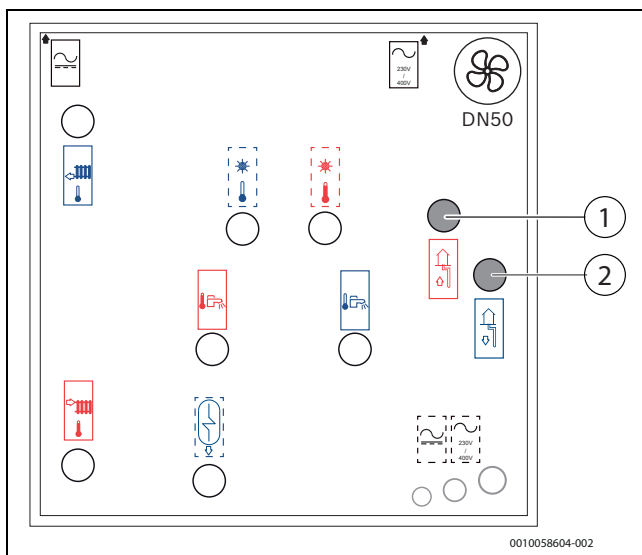
Afb. 46 Aansluitingen van de warmtepomp op het bronsysteem
