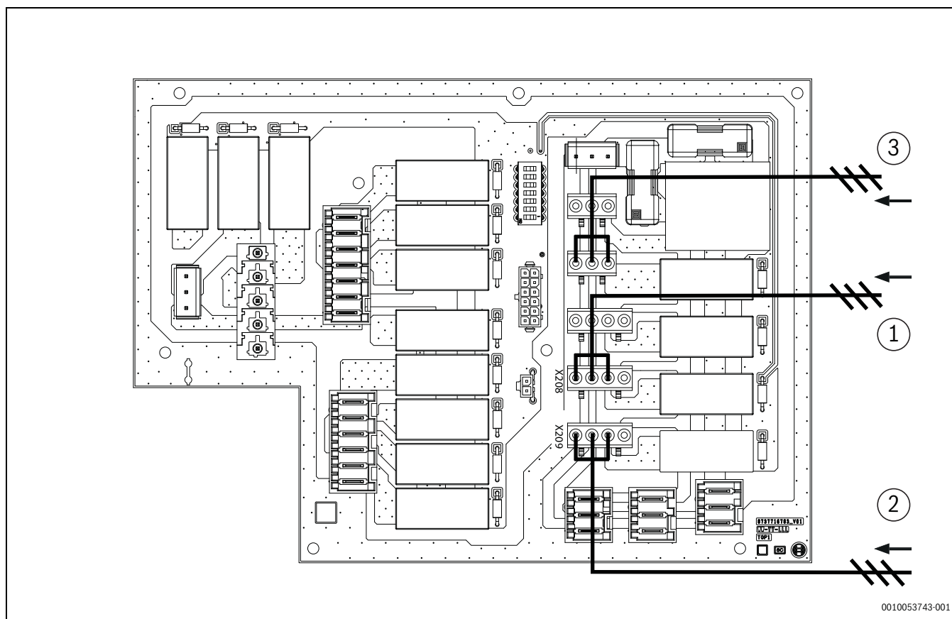
Afb. 60 Elektrische aansluitingen voor accessoires
