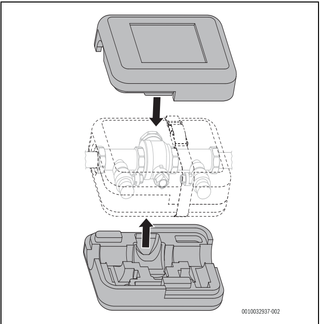
Afb. 56 Isolatie vulinrichting
