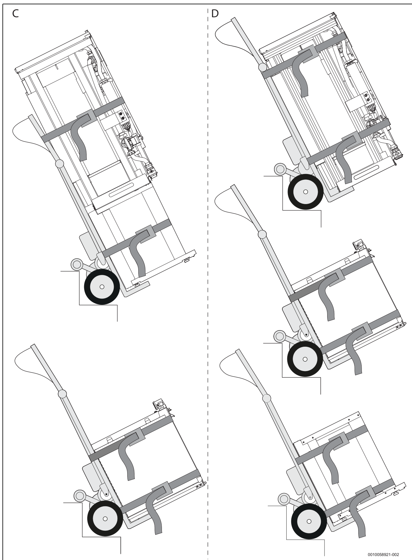
Afb. 11 Transportmogelijkheden C en D
