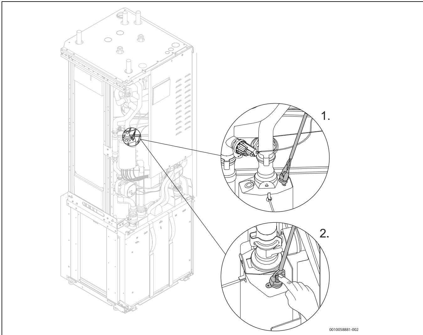
Afb. 69 Reset de oververhittingsbeveiliging.
