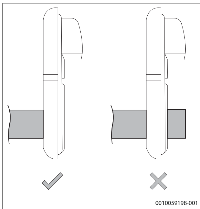
Afb. 40 Plaats de schacht niet te diep in de ventilatorunit
