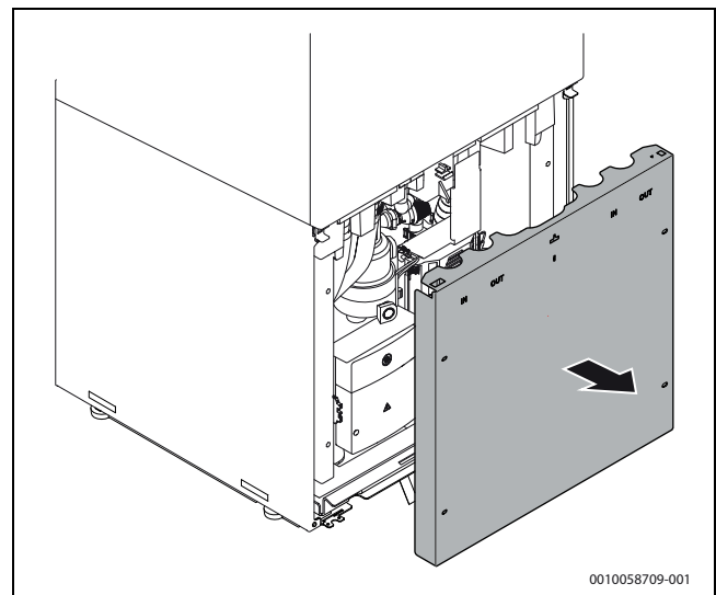
Afb. 19 Verwijder het frontmantel
