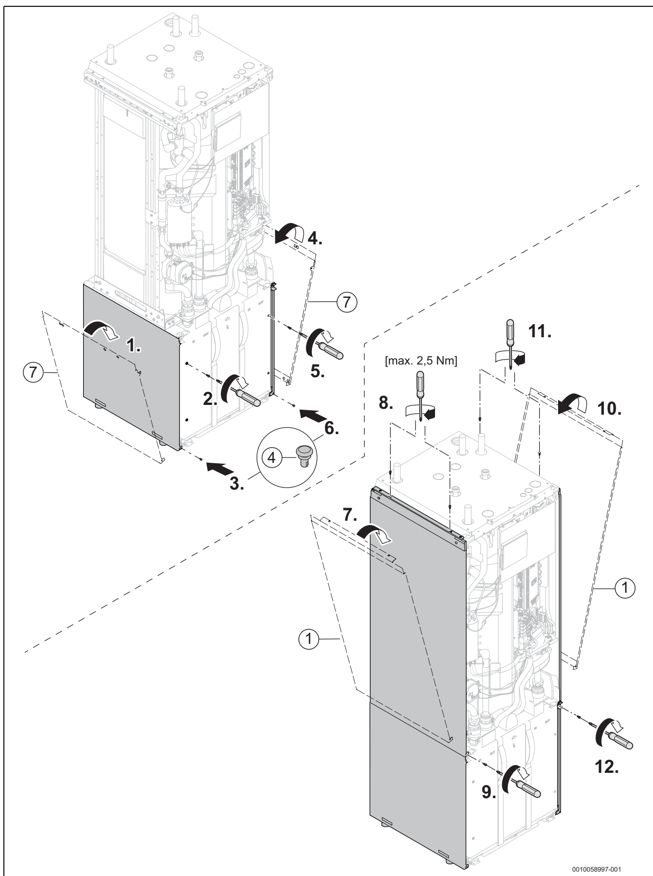
Afb. 7 Bemanteling
