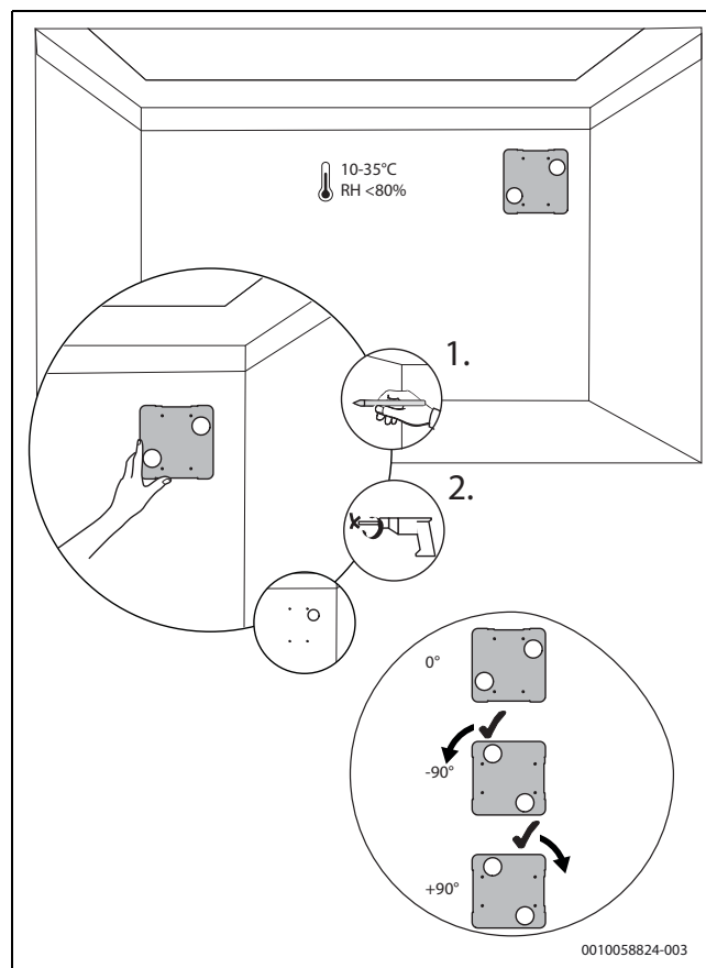
Afb. 33 Markeer waar de console moet worden gemonteerd en waar geboord moet worden
