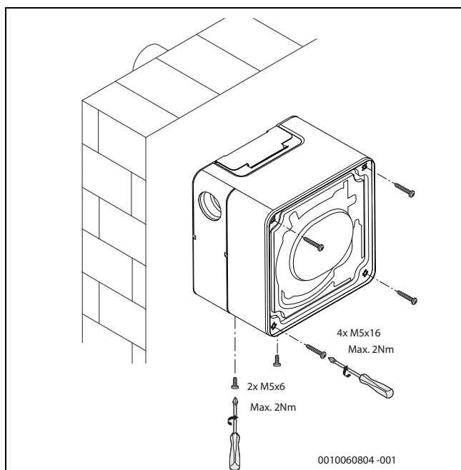
Afb. 44 Hoe de schroeven aandraaien
