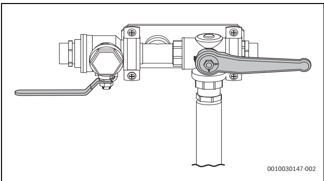
Afb. 53 Vulstation in vulstand
