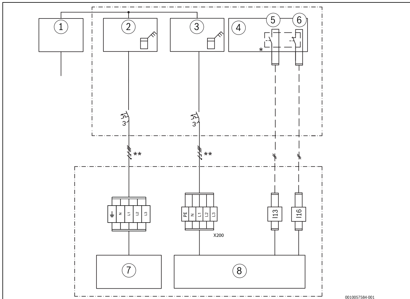
Afb. 65 Aanbevolen oplossing
