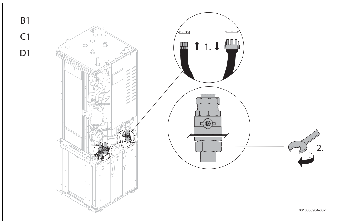
Afb. 12 Opsplitsen warmtepomp
