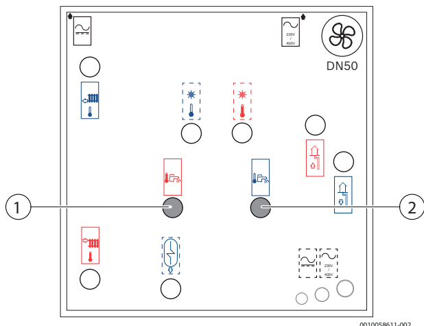
Afb. 48 Wateraansluitingen op de warmtepomp
