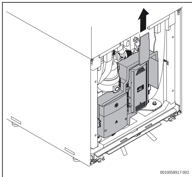
Afb. 20 Verwijder het elektrische paneel.
