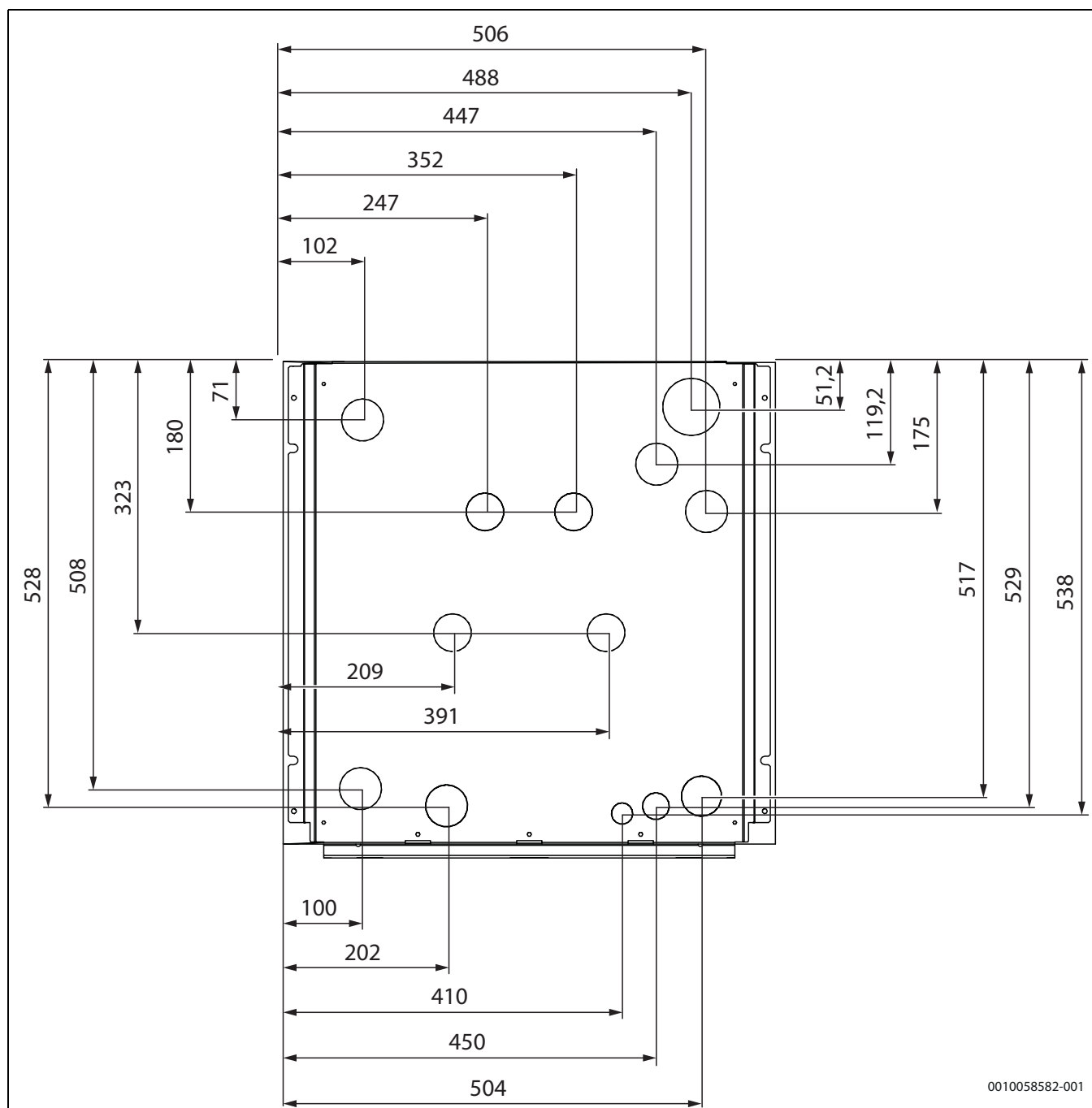
Afb. 3 Afmetingen, aansluitingen, bovenaanzicht
