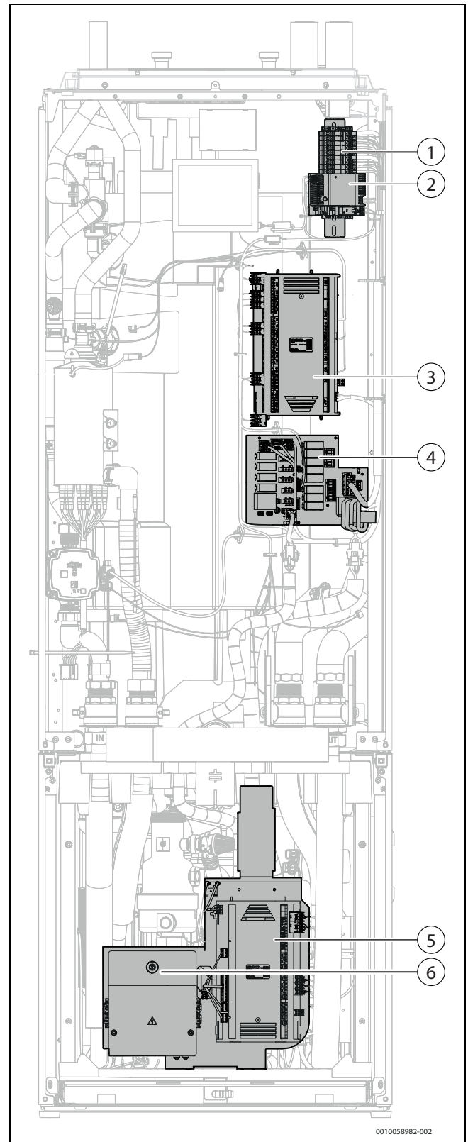
Afb. 57 Elektrische componenten en besturingsunits
