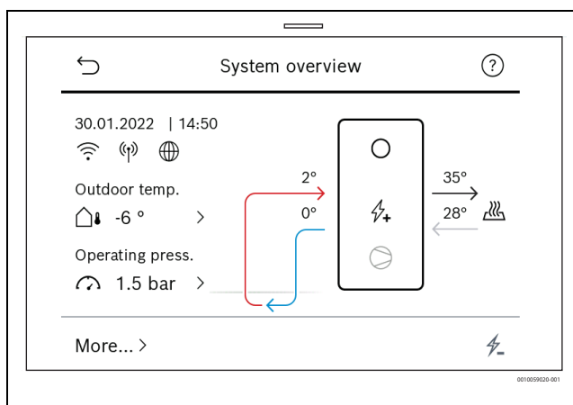
Afb. 67 Overzicht van de warmtepomp
