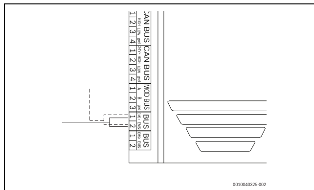
Afb. 64 EMS-verbinding
