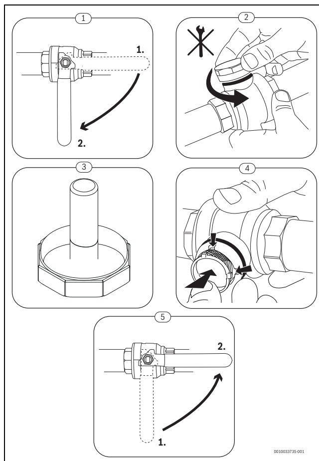
Afb. 68 Deeltjesfilter reinigen
