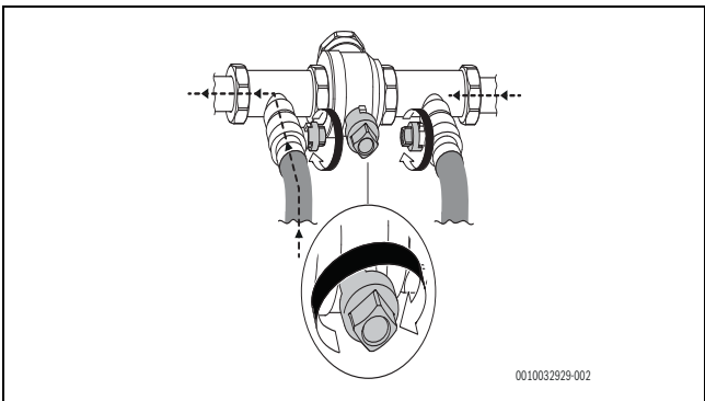
Afb. 54 Vulinrichting in de drukverhogingsstand
