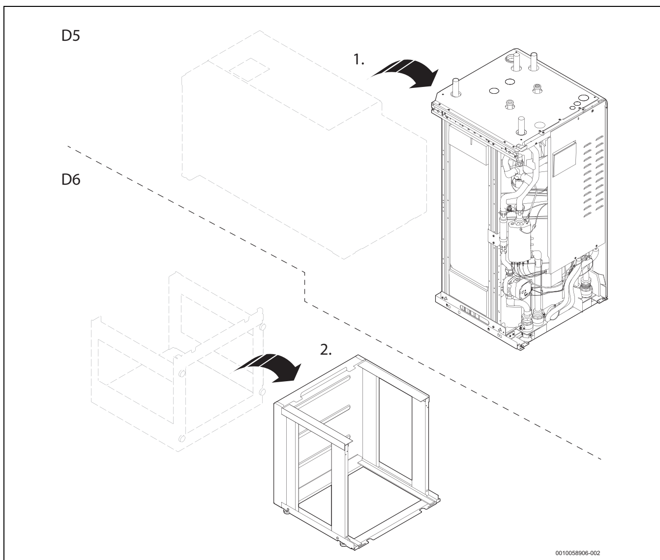
Afb. 16 Opsplitsen warmtepomp
