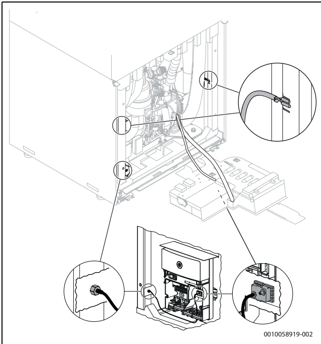
Afb. 24 Controleer de slang en aardingskabel.
