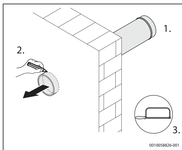
Rys. 35 Przyciąć szacht
