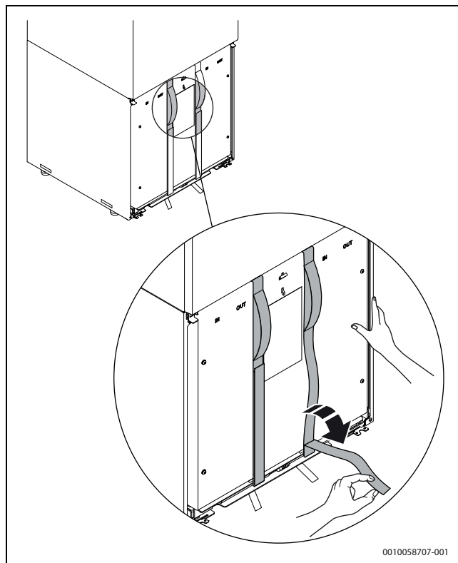
Rys. 17 Poluzować paski
