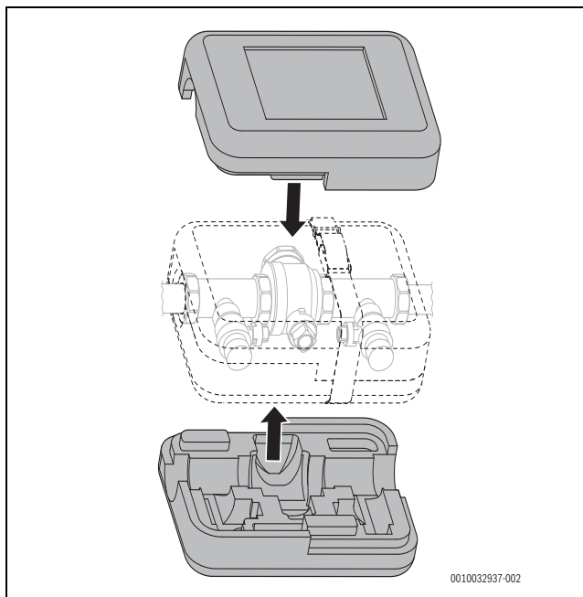
Rys. 56 Izolacja urządzenia napełniającego
