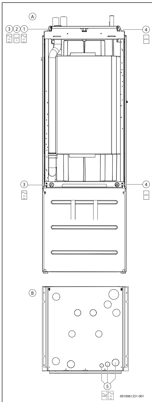
Rys. 58 Przepusty kablowe
