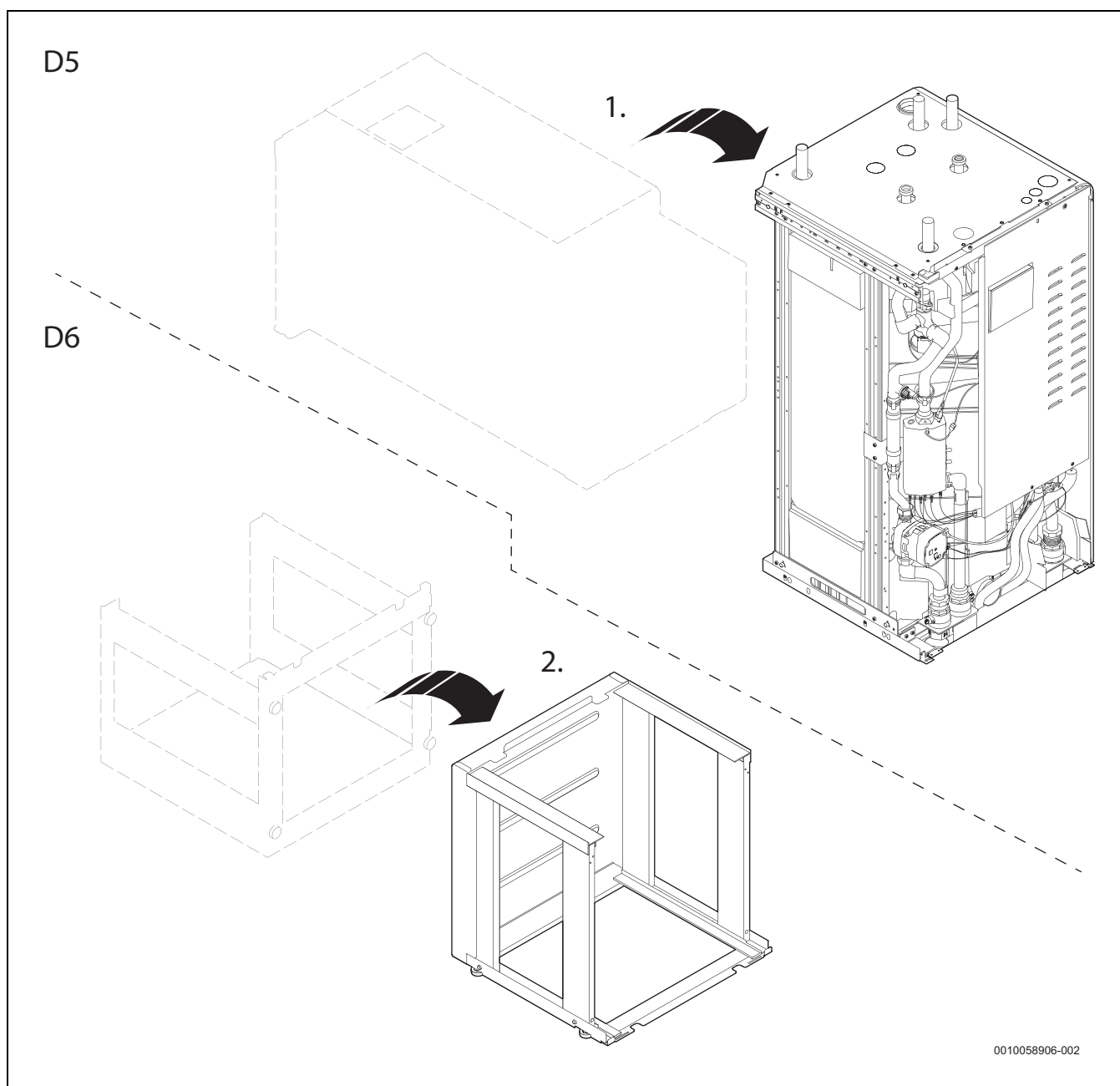
Rys. 16 Podział pompy ciepła
