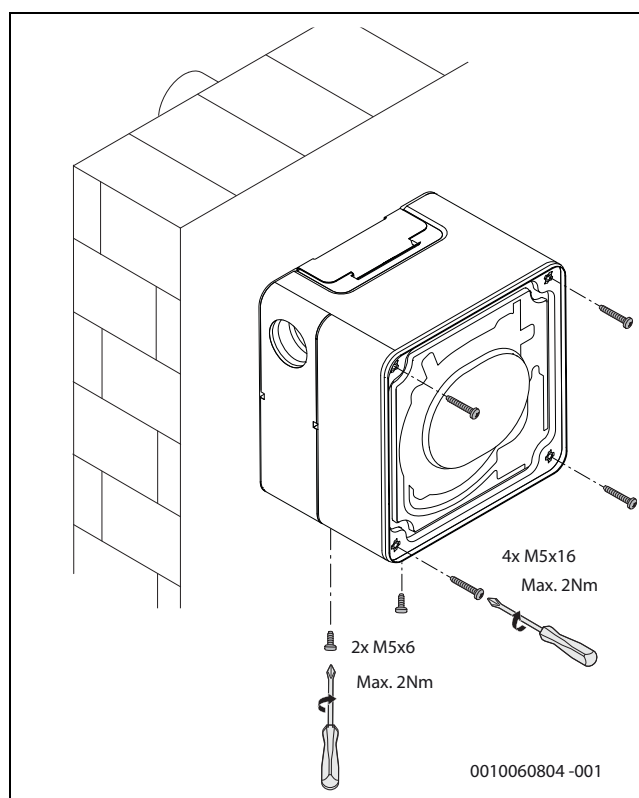
Rys. 44 Jak dokręcić śruby
