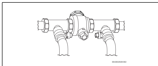
Rys. 49 Zespół napełniający
