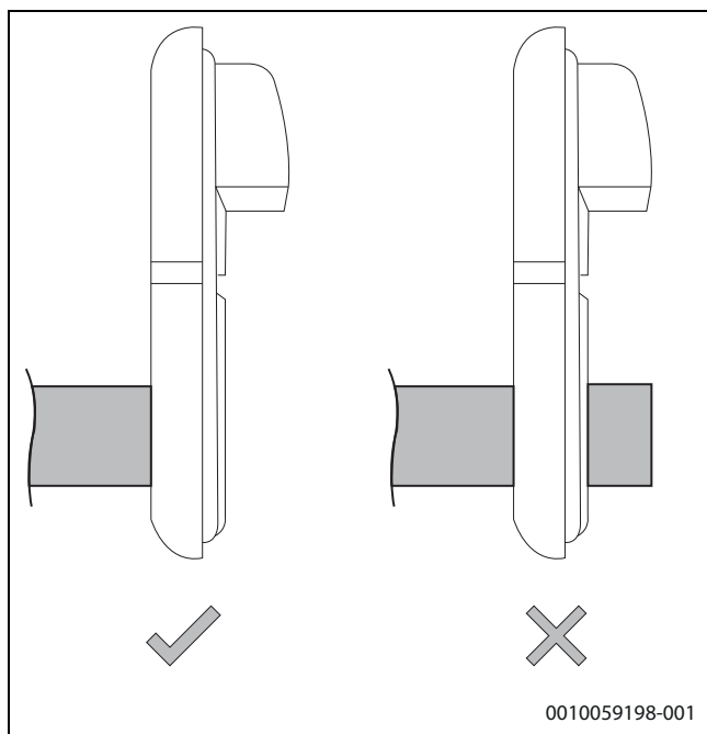
Rys. 40 Nie wsuwać szachtu zbyt głęboko w obudowę wentylatora
