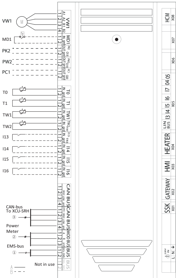
Rys. 61 Podłączenia XCU-THH
