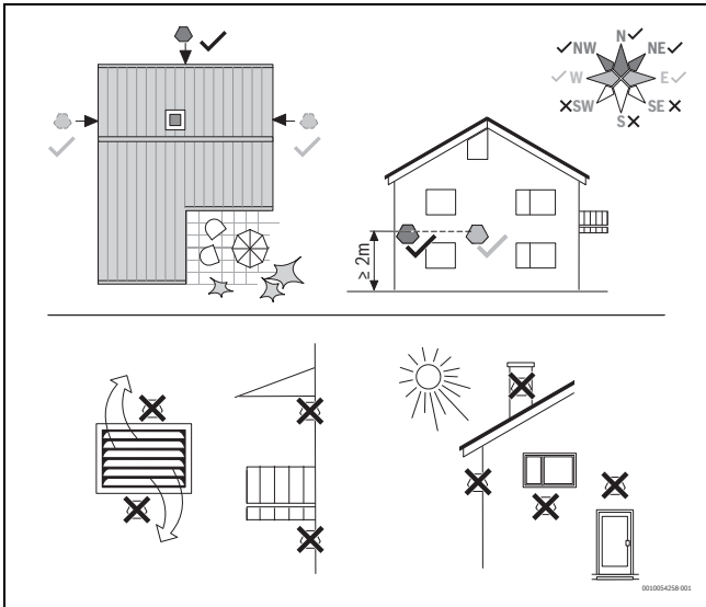
Rys. 63 Położenie czujnika temperatury zewnętrznej
