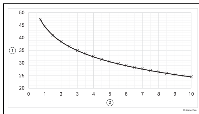
Rys. 29 Poziom ciśnienia akustycznego w trybie ciągłym w przeliczeniu na energię ( L_r(r, Q=4) ) dla wylotu szachtu wentylatora wentylacji awaryjnej umieszczonego na zewnątrz, w funkcji odległości od wylotu szachtu do punktu emisji (miejscu oceny). Całkowity czas oceny wynosi 8 godzin, a wykres przedstawia średni poziom ciśnienia akustycznego w całym okresie oceny
