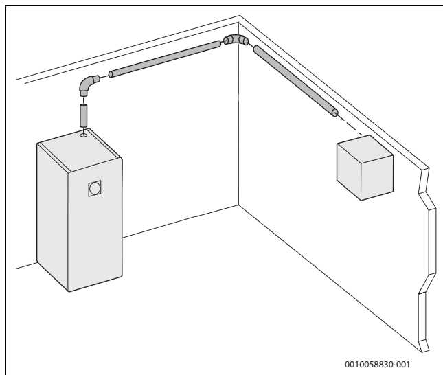
Rys. 39 Jak poprowadzić szachty
