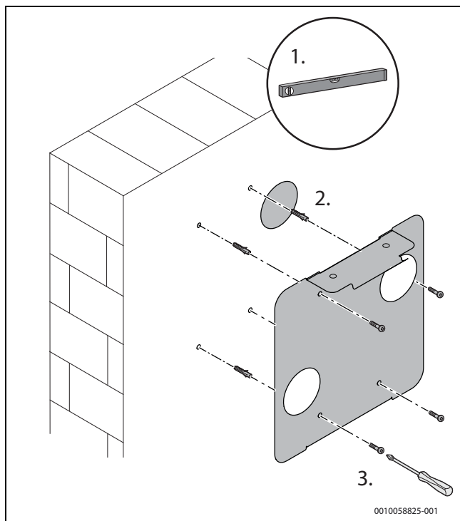
Rys. 34 Zamocować uchwyt
