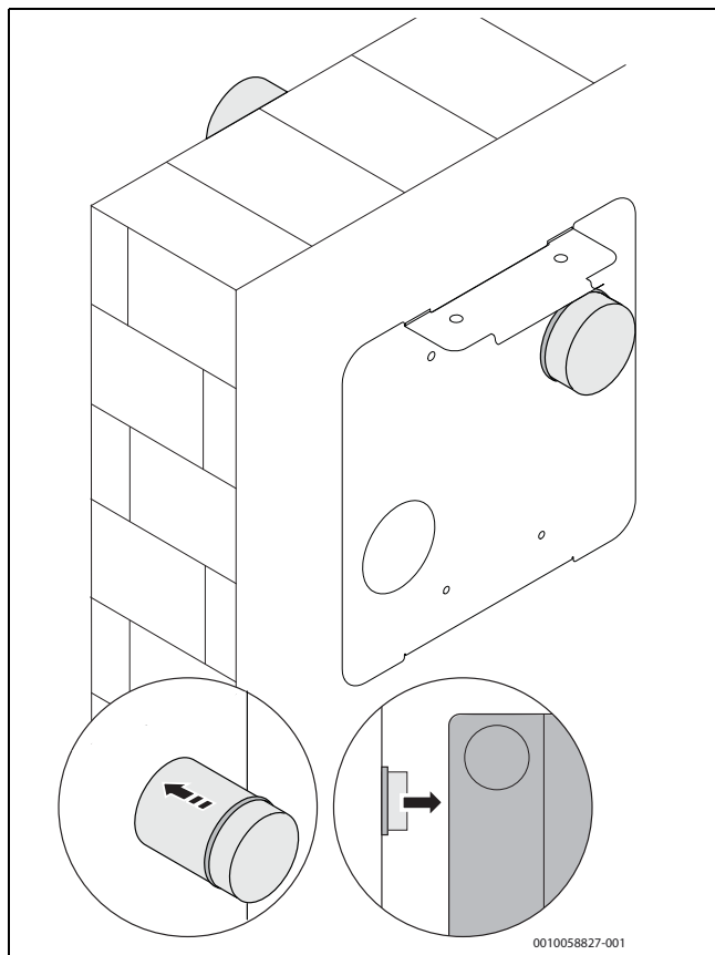
Rys. 36 Wsunąć szacht w otwór w ścianie
