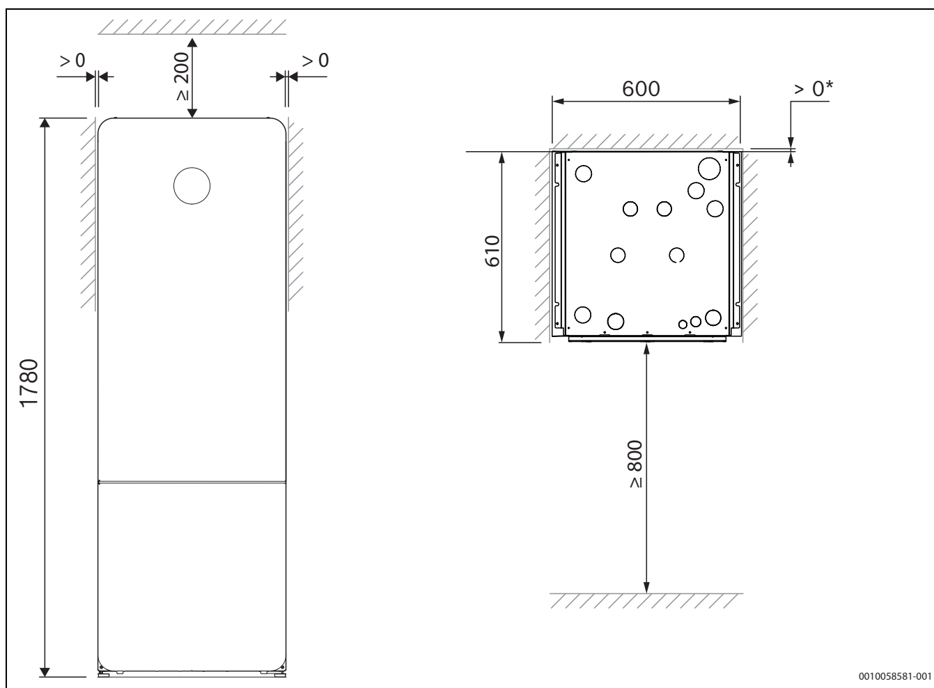
Rys. 2 Wymiary i odległości minimalne
