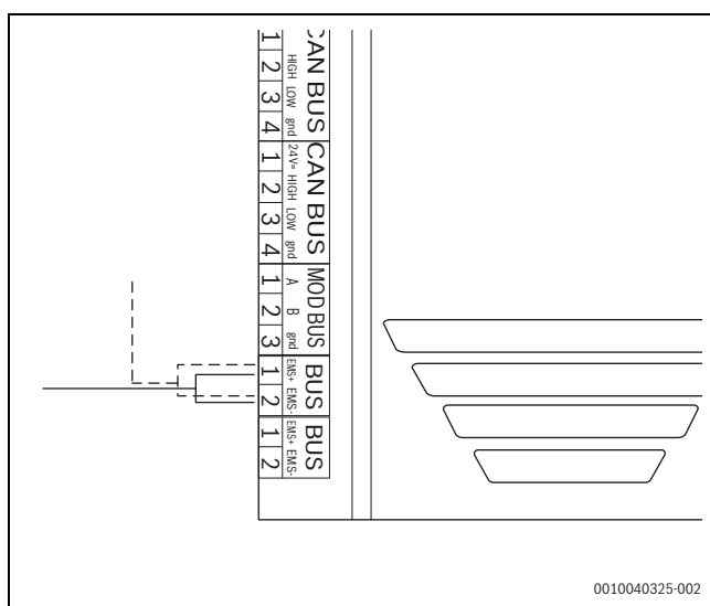
Rys. 64 Podłączanie EMS
