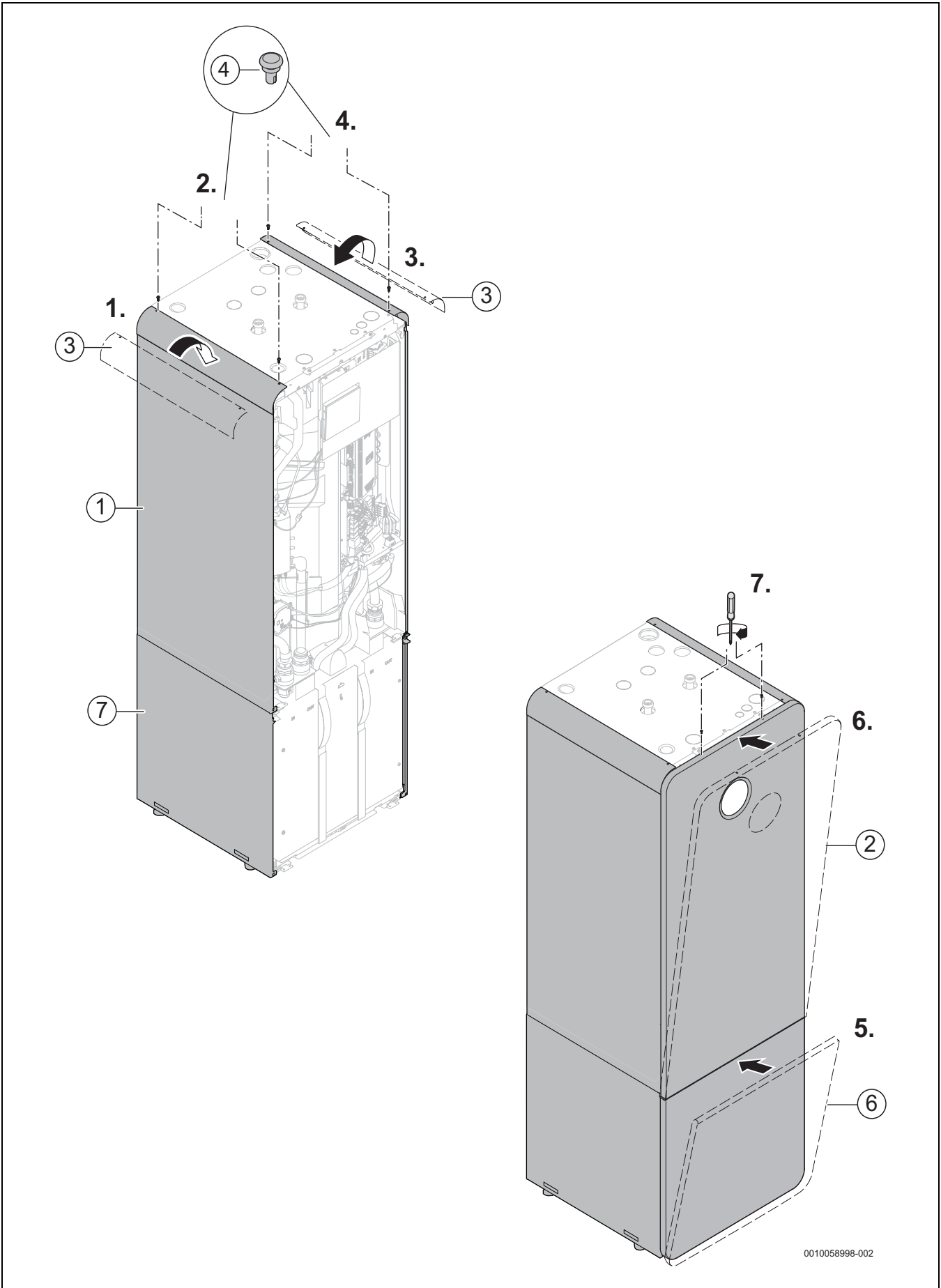
Rys. 8 Montaż zestawu ozdobnego
