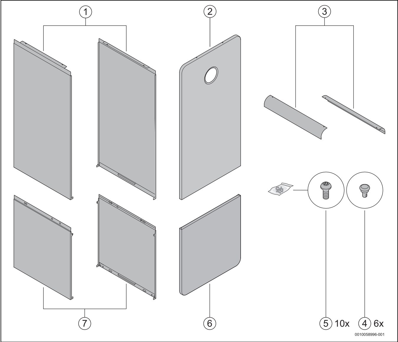
Rys. 6 Montaż zestawu ozdobnego
