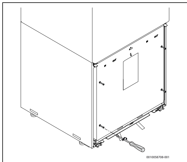
Rys. 18 Odkręcić 4 śruby
