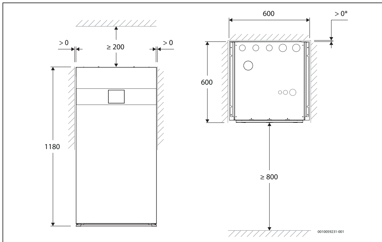
Rys. 2 Wymiary i odległości minimalne
