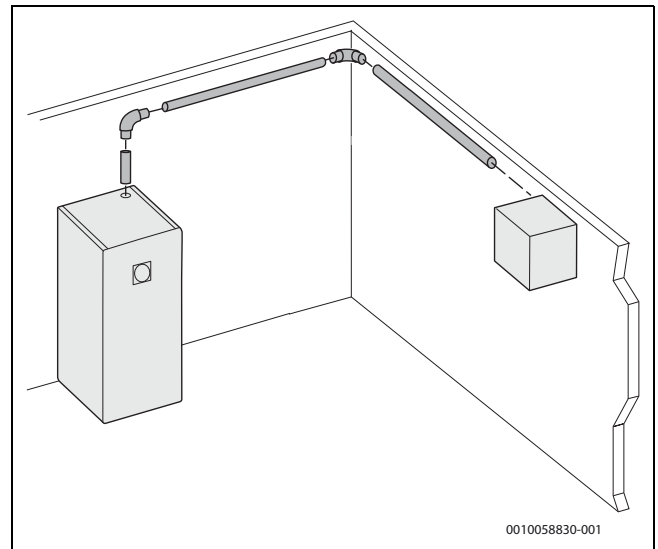
Rys. 38 Jak poprowadzić szachty
