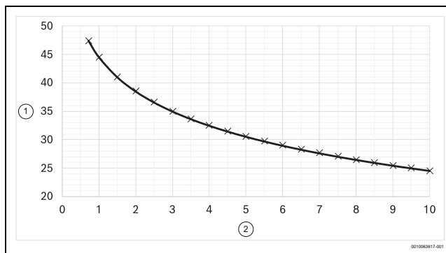
Rys. 28 Poziom ciśnienia akustycznego w trybie ciągłym w przeliczeniu na energię ( L_p(r, Q=4) ) dla wylotu szachtu wentylatora wentylacji awaryjnej umieszczonego na zewnątrz, w funkcji odległości od wylotu szachtu do punktu emisji (miejsca oceny). Całkowity czas oceny wynosi 8 godzin, a wykres przedstawia średni poziom ciśnienia akustycznego w całym okresie oceny
