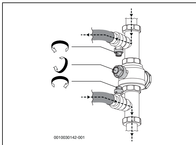
Rys. 50 Urządzenie napełniające w pozycji napełniania
