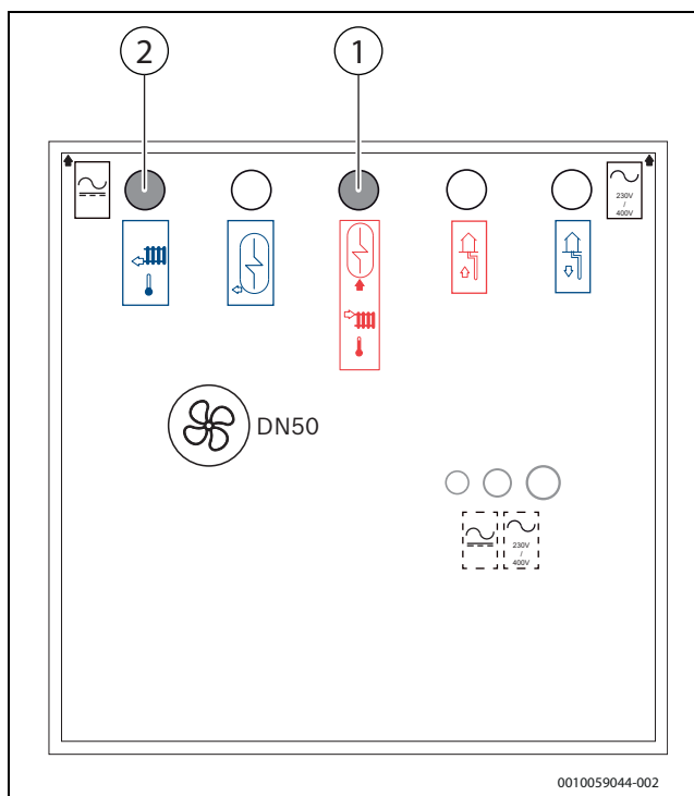
Rys. 46 Podłączenie pompy ciepła do instalacji grzewczej
