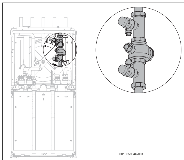
Rys. 48 Zespół napełniający
