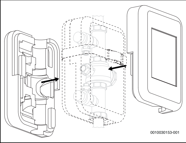
Rys. 55 Izolacja urządzenia napełniającego
