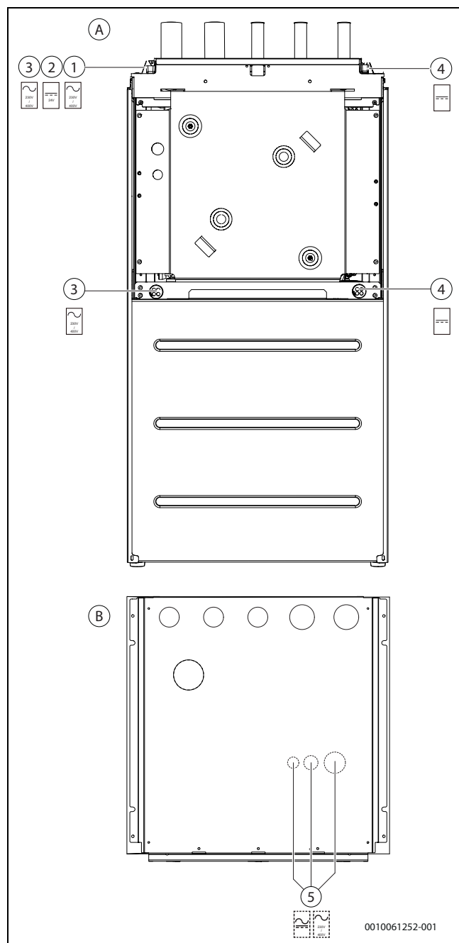
Rys. 57 Przepusty kablowe
