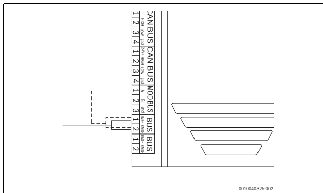
Rys. 63 Podłączenie EMS
