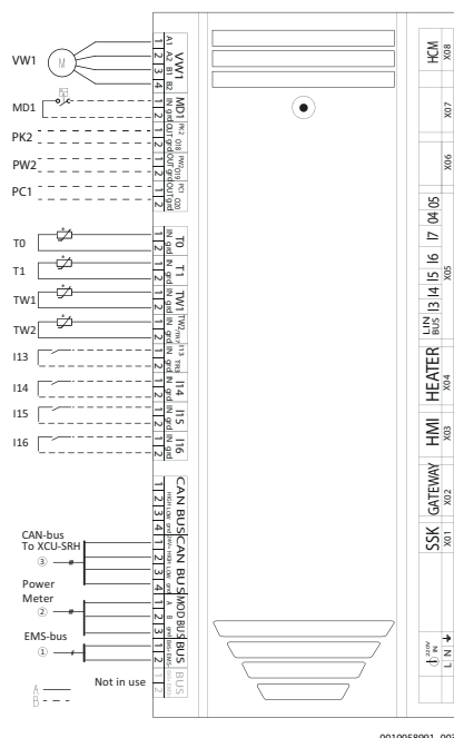
Rys. 60 Podłączenia XCU-THH (XCU HY)
