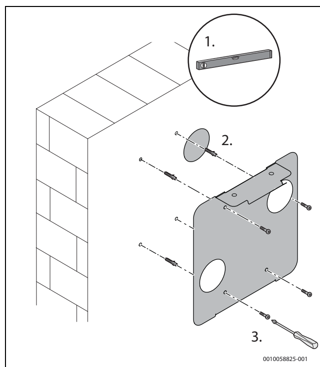
Rys. 33 Zamocować uchwyt
