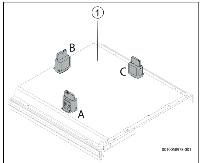
Rys. 27 Przykładowy sposób umieszczenia Modułu radiowy
