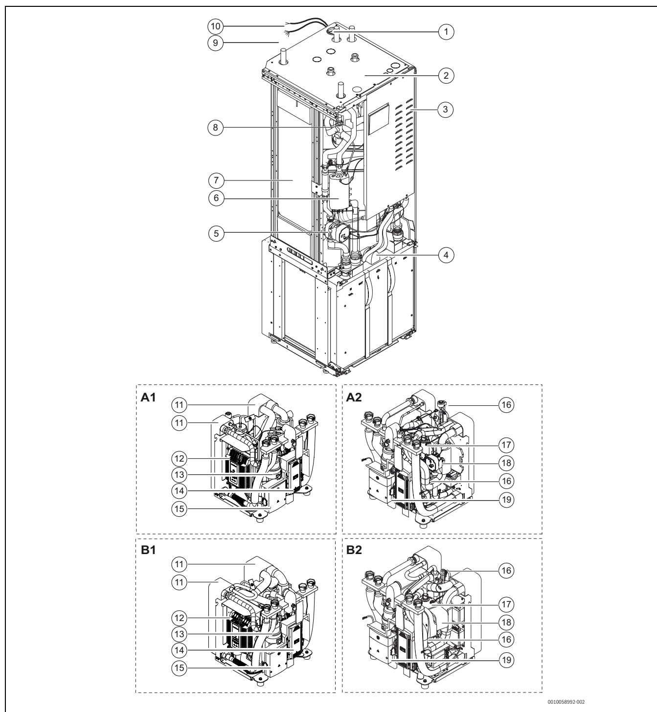
Rys. 4 Przegląd produktu
