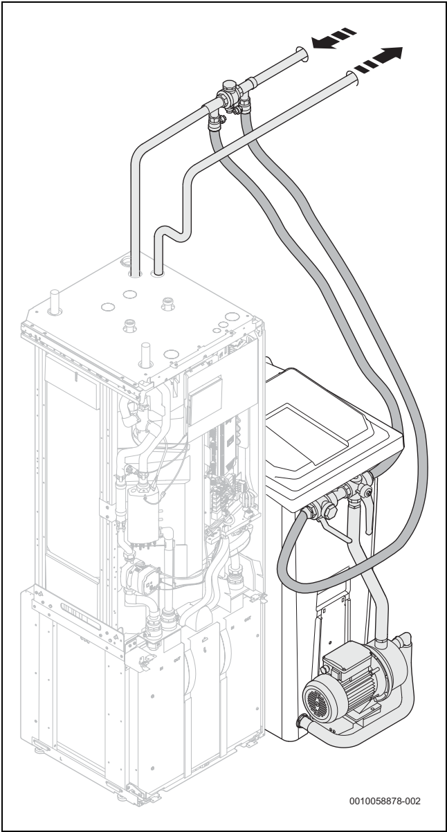
Rys. 50 Napełnianie za pomocą stacji napełniającej
