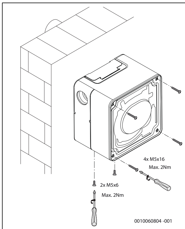
Rys. 44 Jak dokręcić śruby
