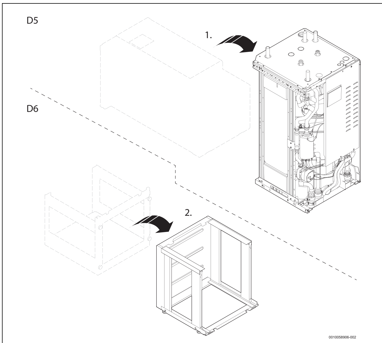
Rys. 16 Podział pompy ciepła
