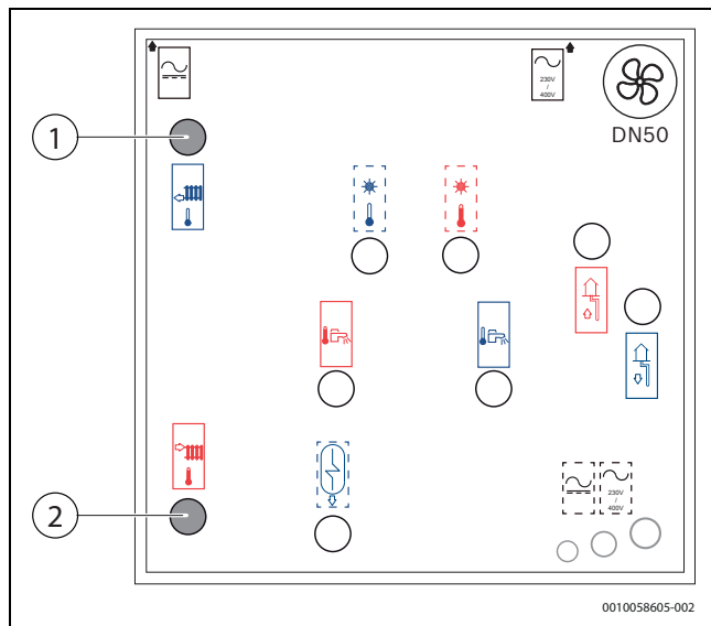
Rys. 47 Podłączenie pompy ciepła do instalacji grzewczej
