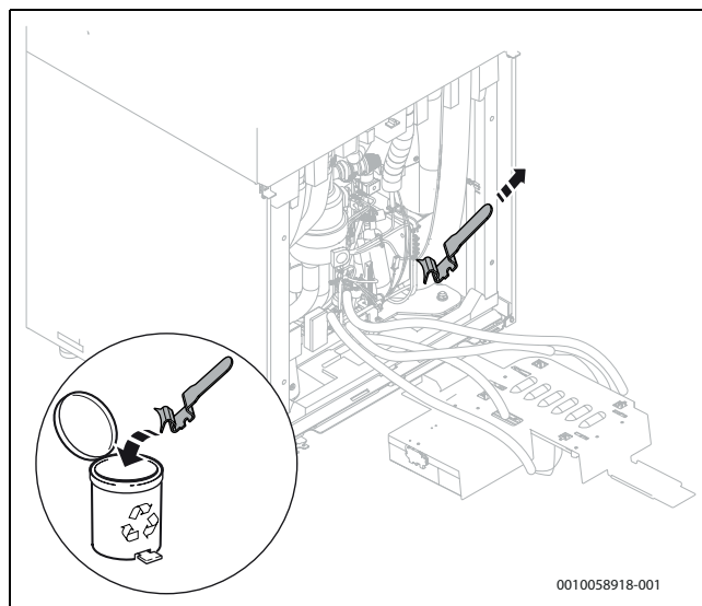
Rys. 23 Zdjąć uchwyt transportowy
