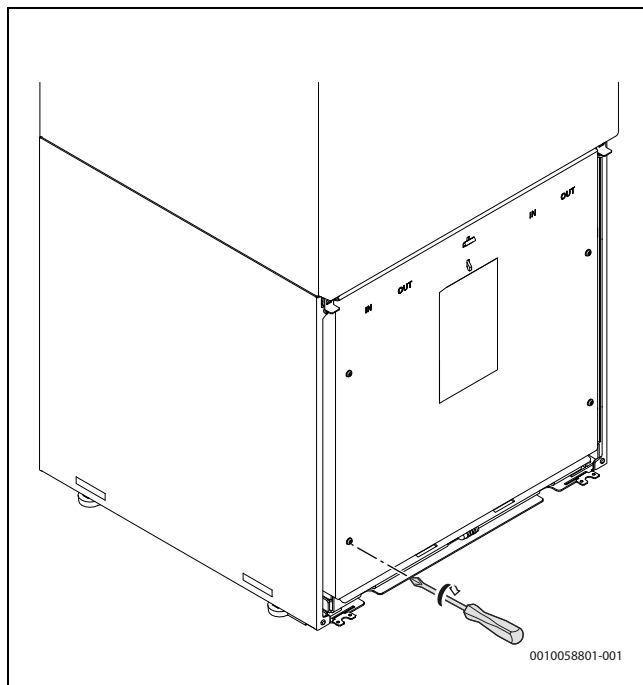
Rys. 27 Wkręcić i dokręcić 4 śruby
