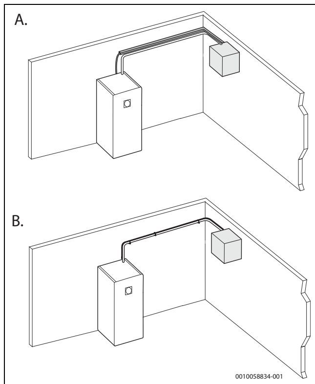
Rys. 41 Jak poprowadzić kable od urządzenia do obudowy wentylatora
