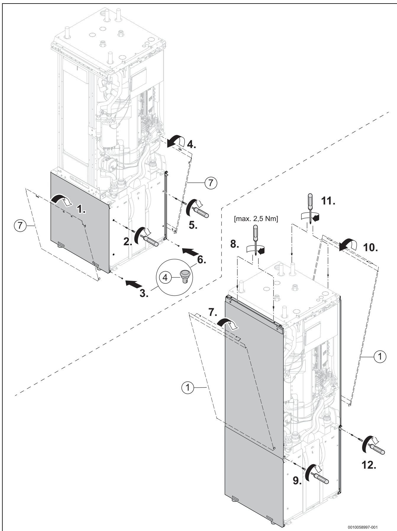
Rys. 7 Montaż zestawu ozdobnego
