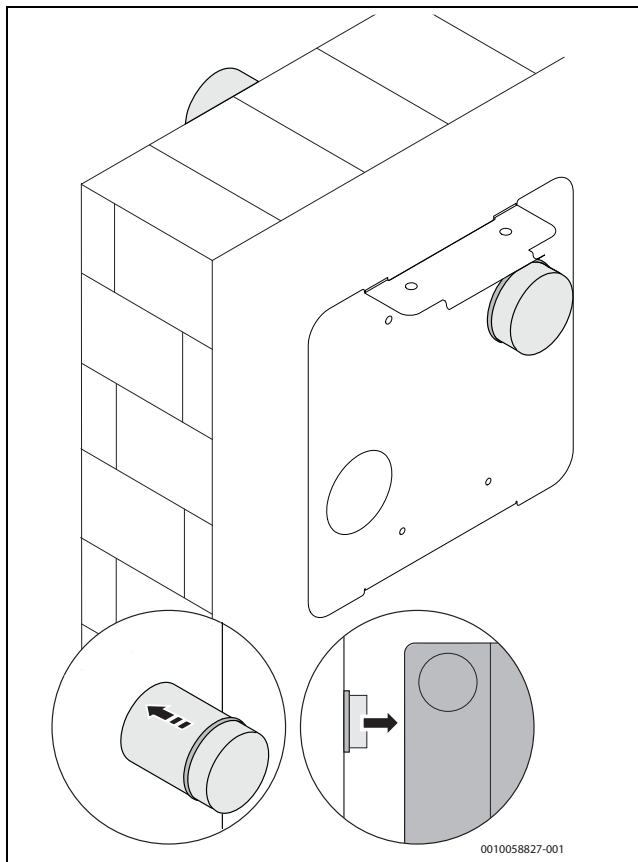
Rys. 36 Wsunąć szacht w otwór w ścianie
