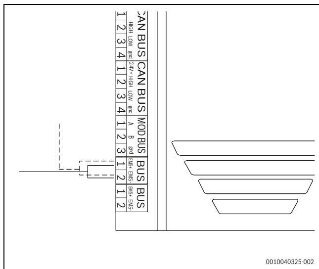
Rys. 64 Podłączenie EMS
