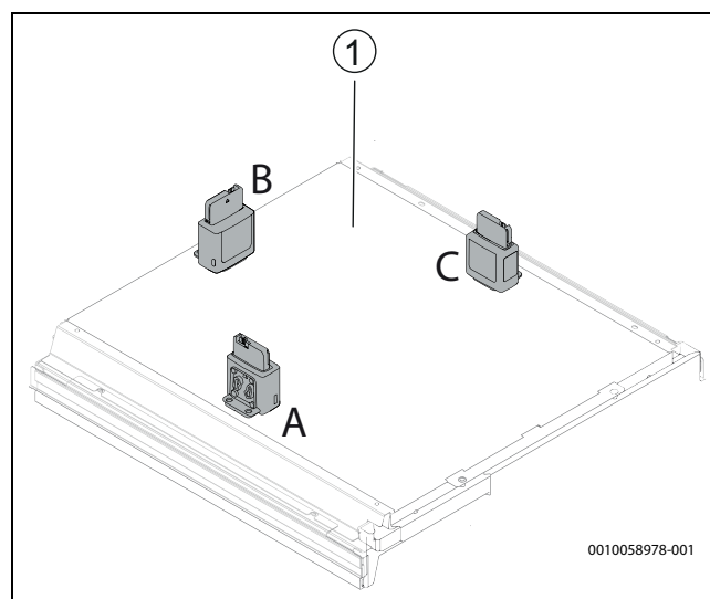
Rys. 28 Przykładowy sposób umieszczenia Modułu radiowy
