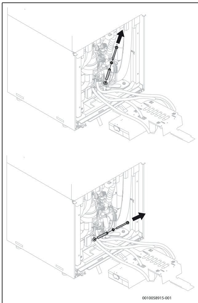
Rys. 21 Odkręcić śruby mocujące uchwyt
