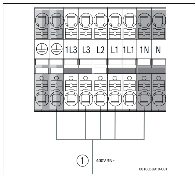
Rys. 59 Standardowe doprowadzenie zasilania ustawione fabrycznie (6 kW, 8 kW, 13 kW, 17 kW)
