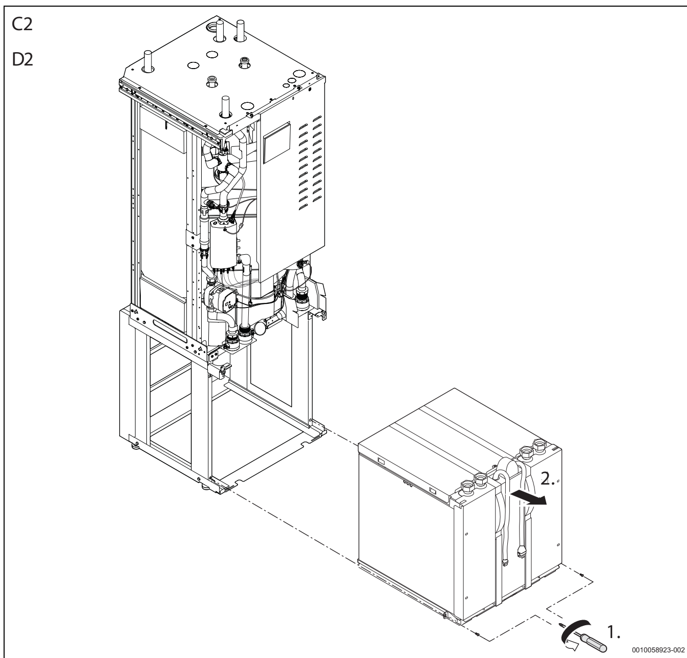
Rys. 14 Podział pompy ciepła
