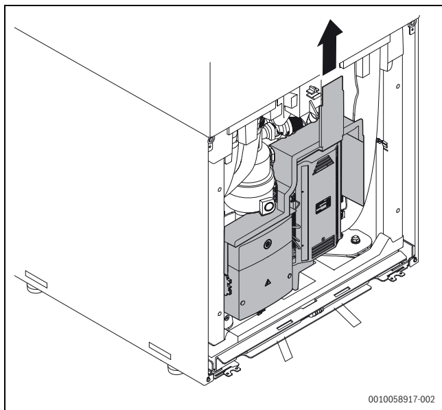
Rys. 20 Zdjąć panel elektryczny
