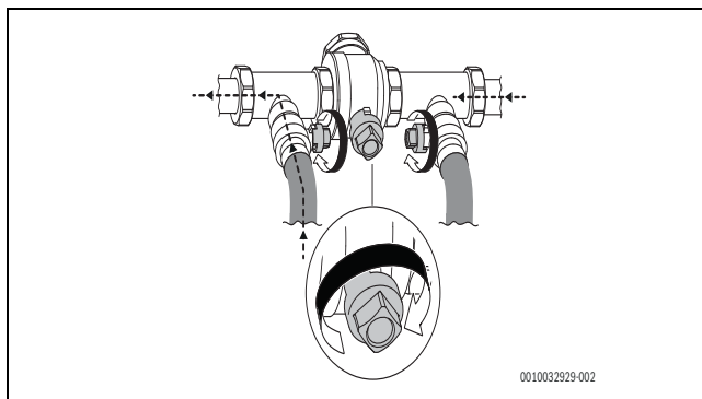
Rys. 54 Urządzenia napełniające w pozycji zwiększania ciśnienia
