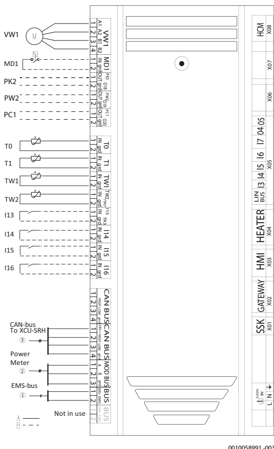
Rys. 61 Podłączenia XCU-THH (XCU HY)
