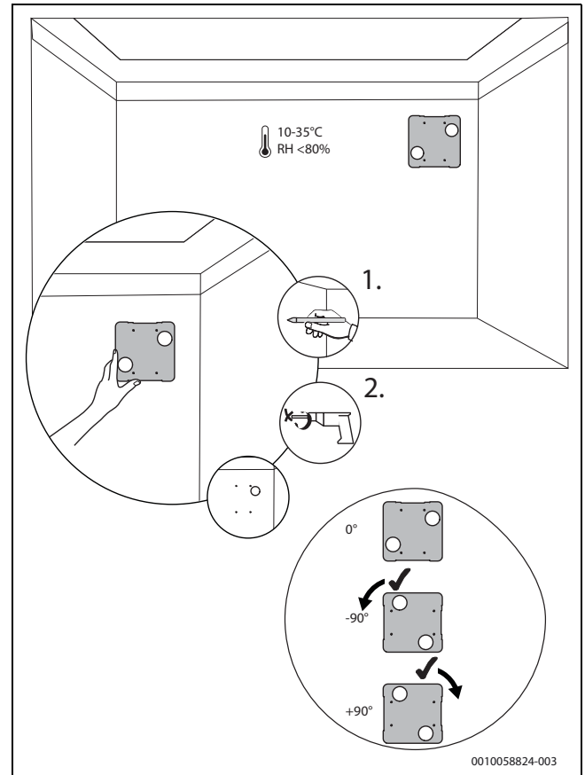
Rys. 33 Zaznaczyć miejsca montażu uchwytu oraz miejsca wiercenia
