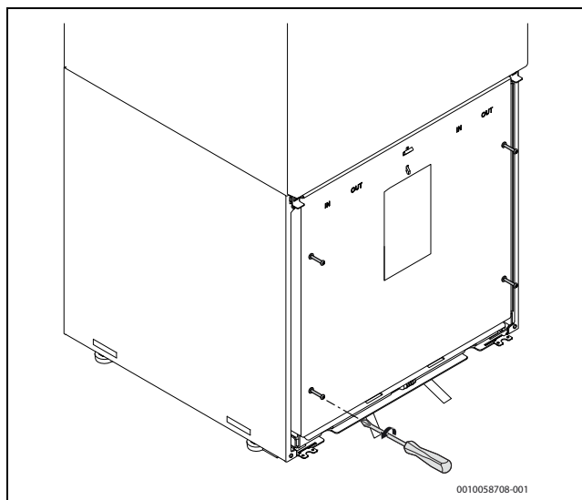
Rys. 18 Odkręcić 4 śruby
