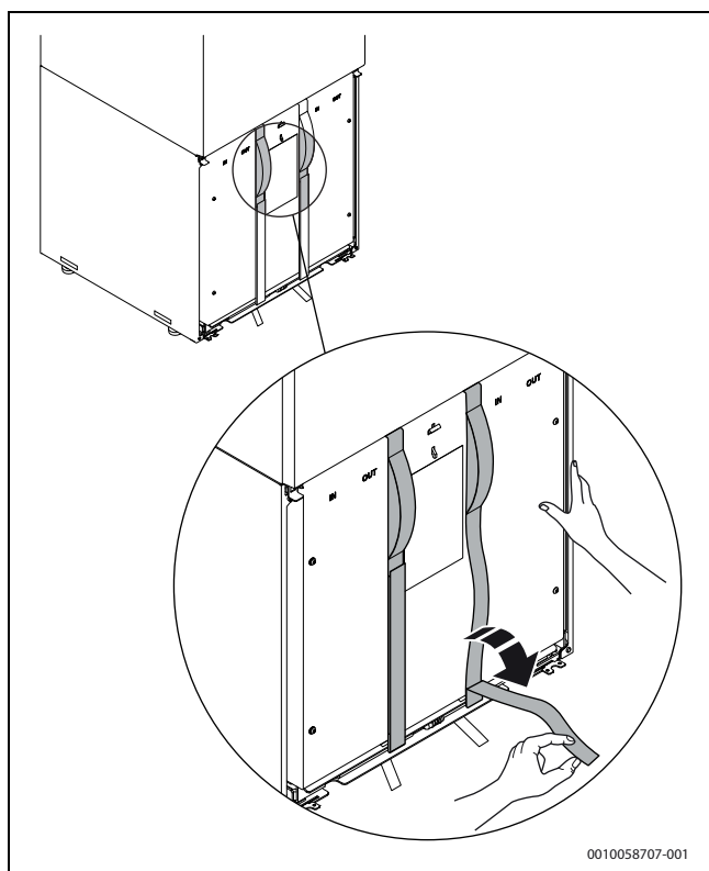
Rys. 17 Poluzować paski
