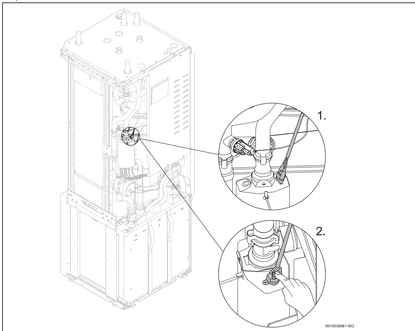
Rys. 68 Zresetować zabezpieczenie przed przegrzaniem
