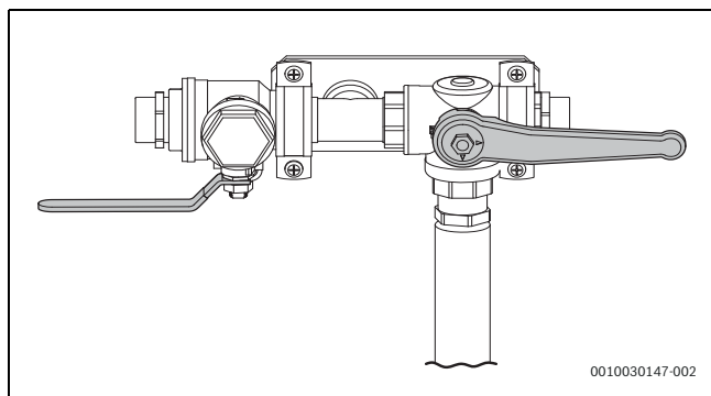
Rys. 53 Stacja napełniająca w pozycji napełniania
