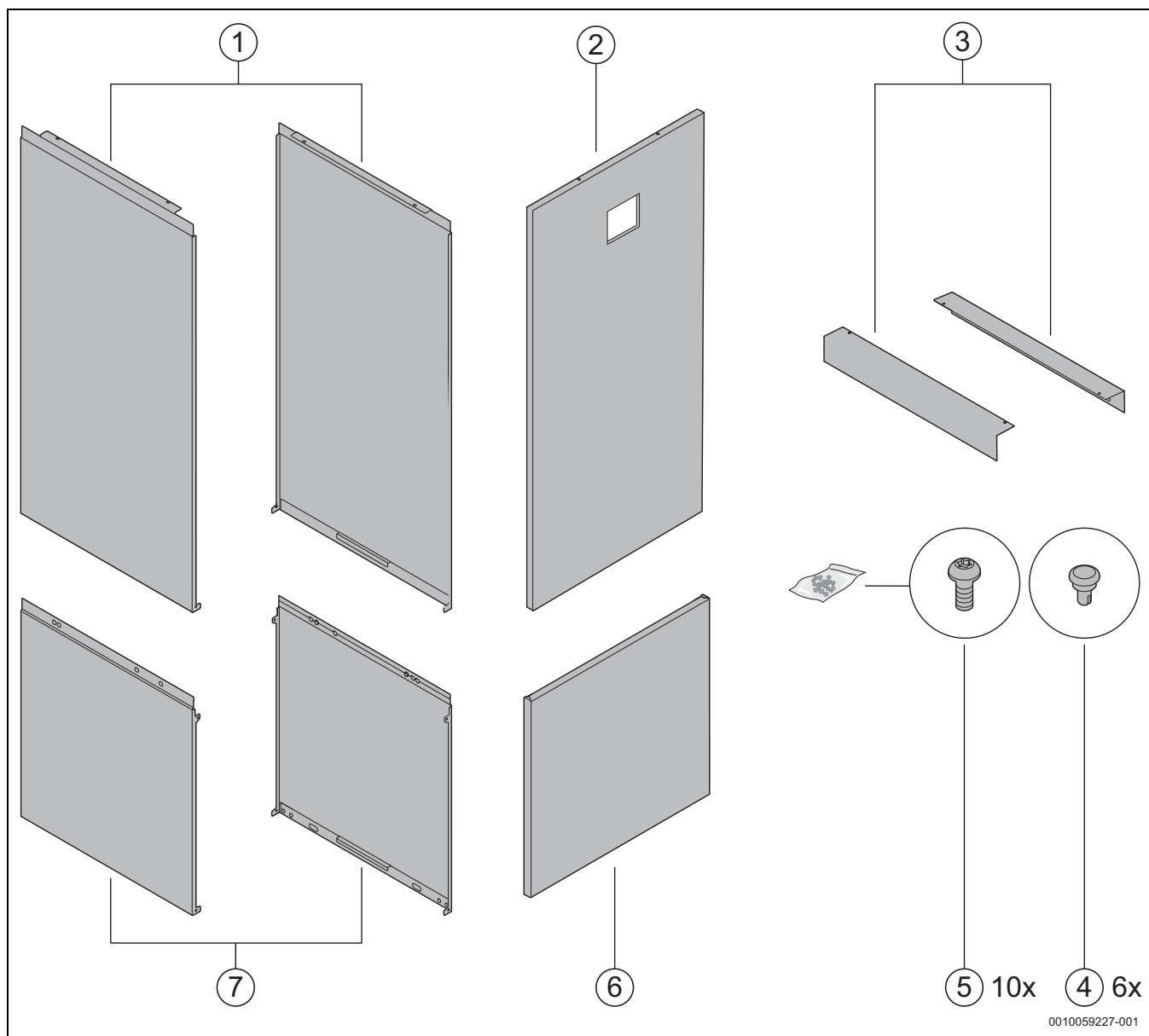
Rys. 6 Montaż zestawu ozdobnego
