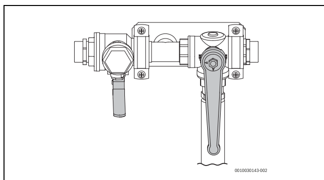
Rys. 52 Stacja napełniająca w pozycji mieszania
