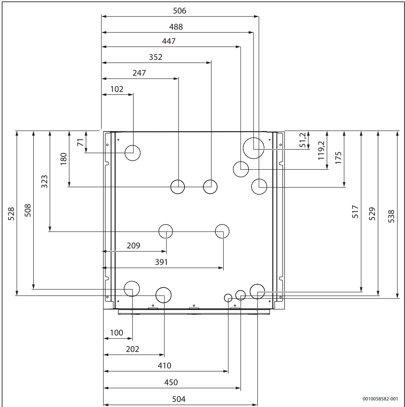
Rys. 3 Wymiary, przyłącza – widok z góry
