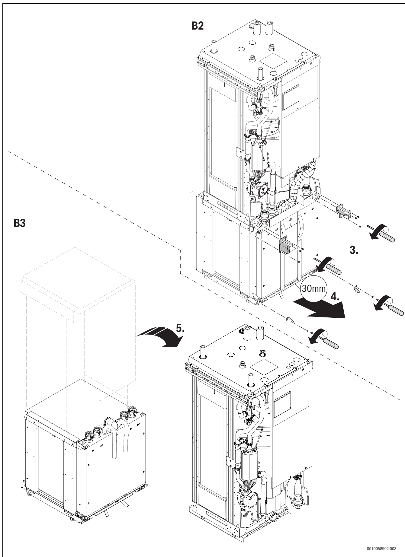
Rys. 13 Podział pompy ciepła
