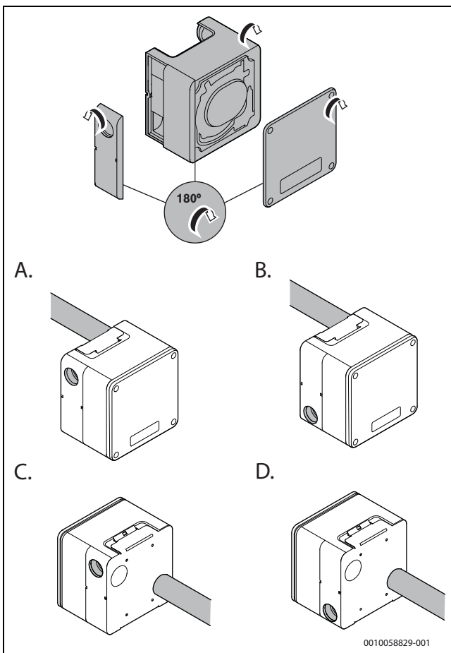
Rys. 32 Sposoby montażu obudowy wentylatora
