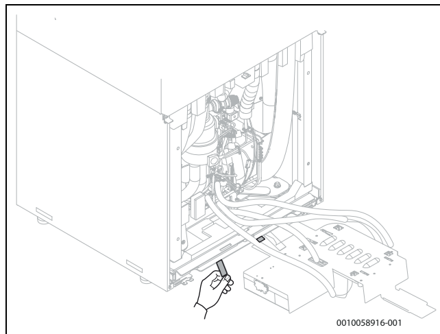
Rys. 22 Zdjąć paski znacznikowe
