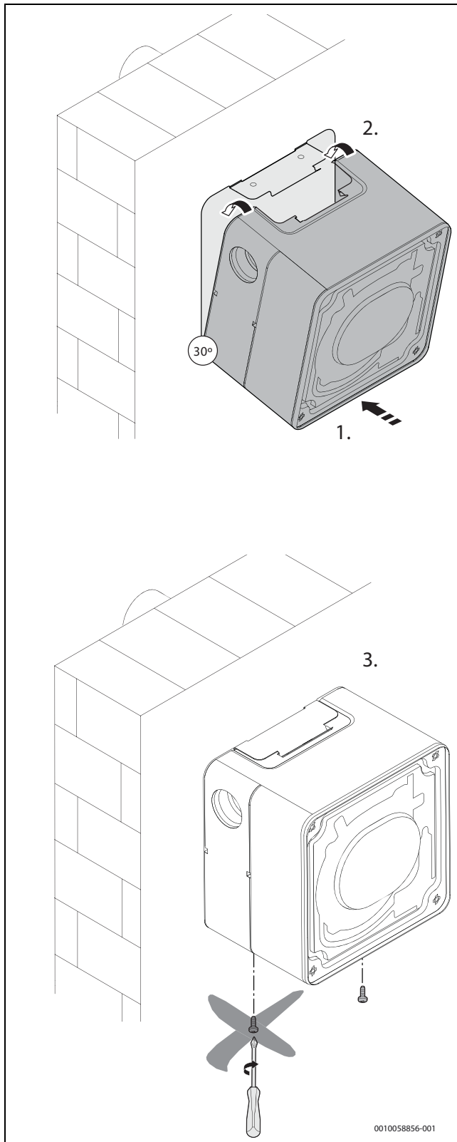
Rys. 38 Zamocować obudowę wentylatora do uchwytu
