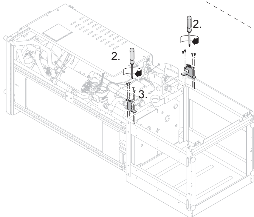
Rys. 15 Podział pompy ciepła
