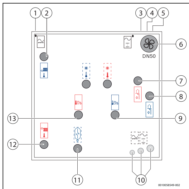
Rys. 5 Przyłącza pompy ciepła, widok z góry
