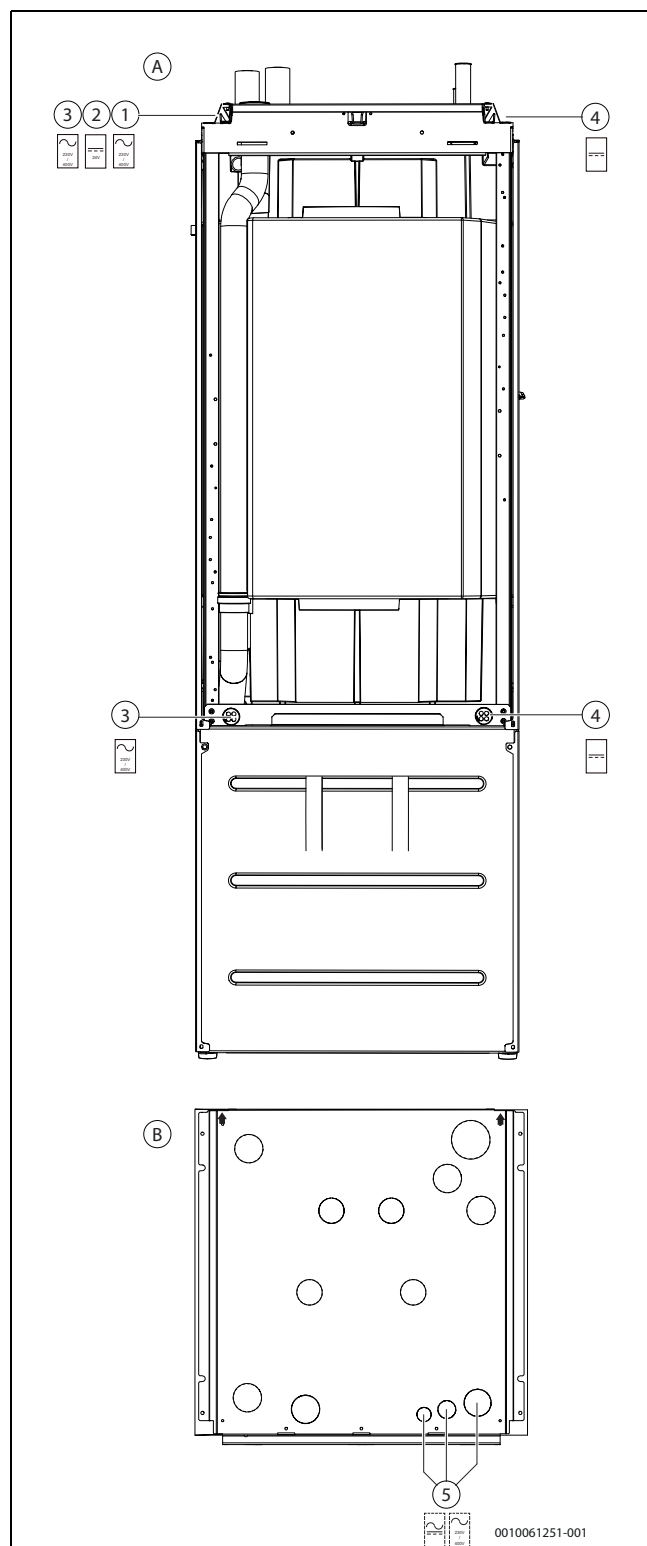
Rys. 58 Przepusty kablowe
