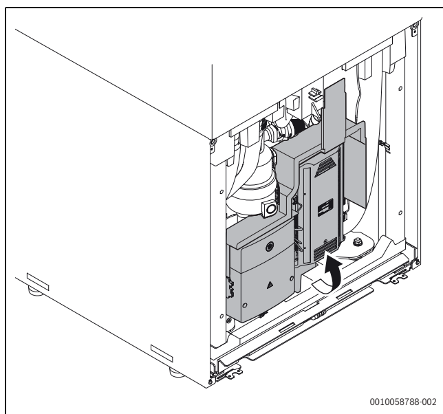
Rys. 25 Zamontować z powrotem panel elektryczny
