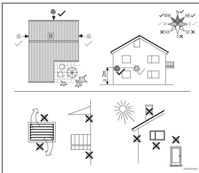
Rys. 63 Położenie czujnika temperatury zewnętrznej
