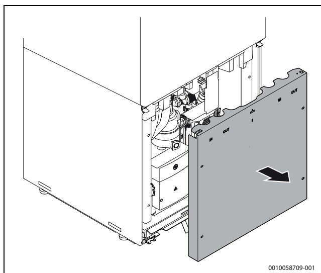
Rys. 19 Zdejmowanie przedniej pokrywy
