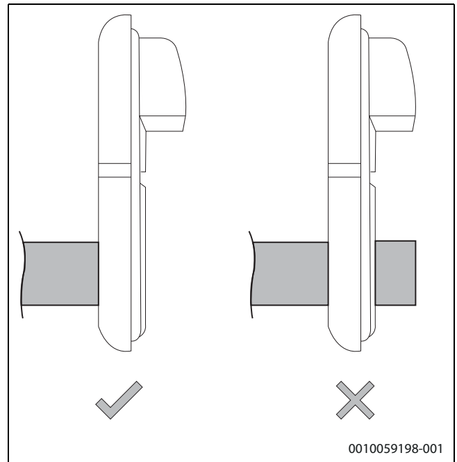
Rys. 40 Nie wsuwać szachtu zbyt głęboko w obudowę wentylatora
