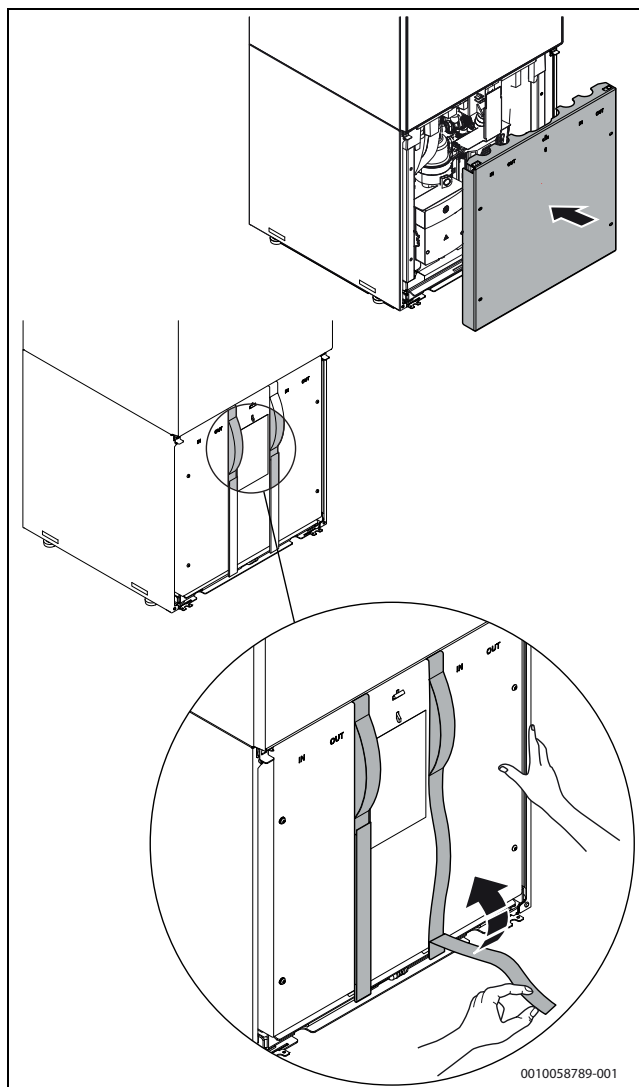
Rys. 26 Zamontować z powrotem pokrywę przednią
