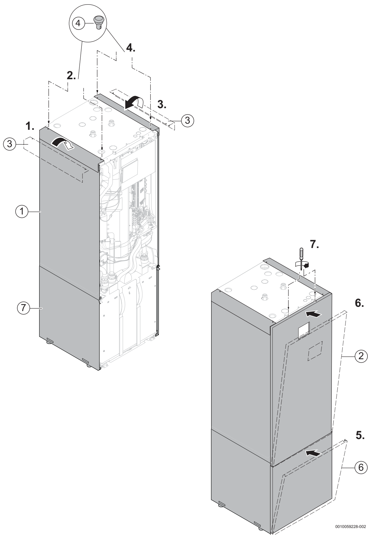
Rys. 8 Montaż zestawu ozdobnego
