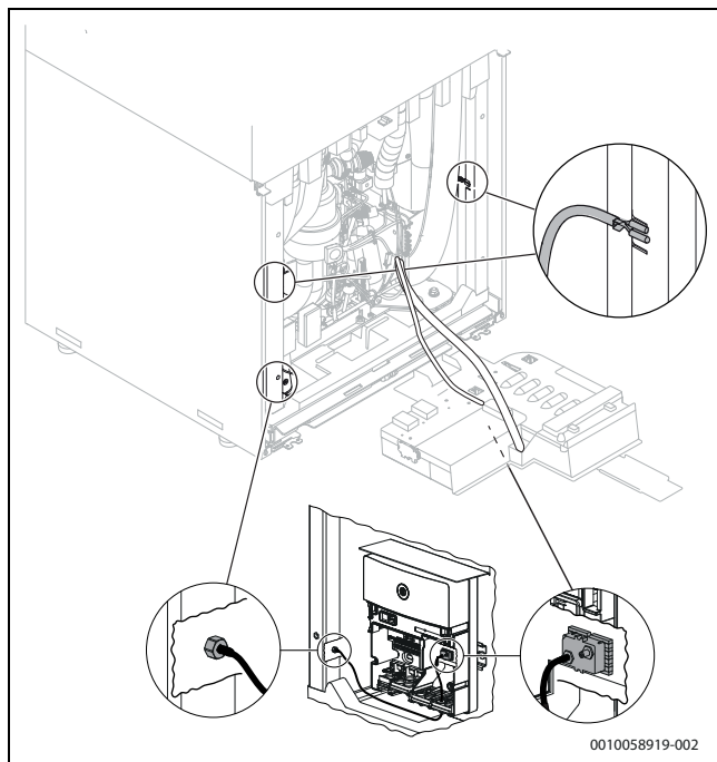
Rys. 24 Sprawdzić węzł i kabel uziemiający
