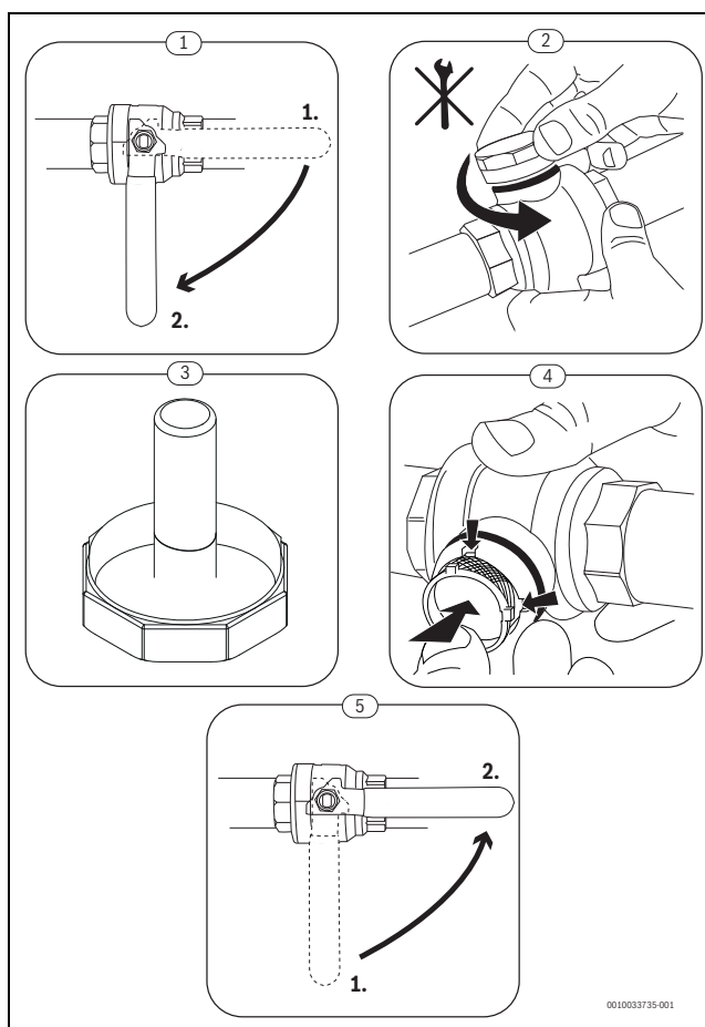
Rys. 67 Czyszczenie filtra cząstek stałych
