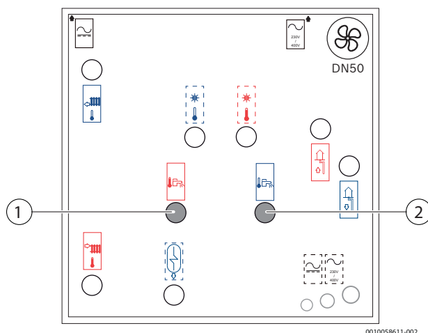
Rys. 48 Przyłącza wody do pompy ciepła
