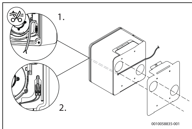
Rys. 42 Jak poprowadzić kable w obudowie wentylatora
