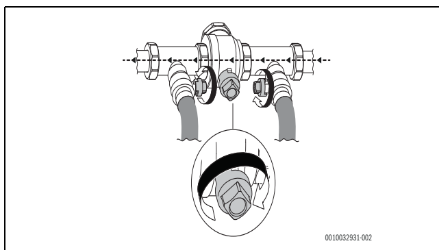
Rys. 55 Urządzenie napełniające w pozycji normalnej
