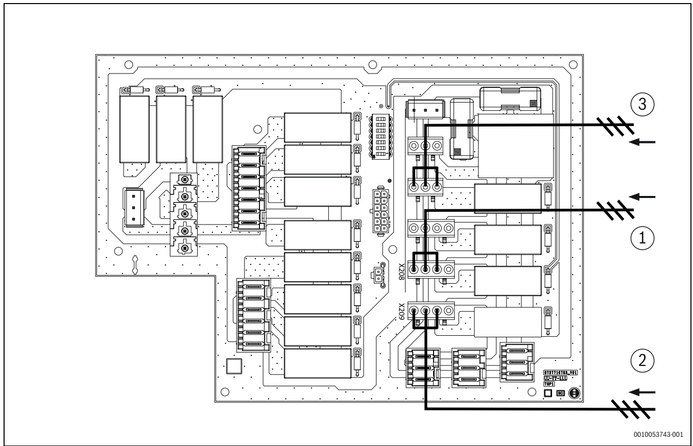
Rys. 60 Podłączenia elektryczne osprzętu dodatkowego
