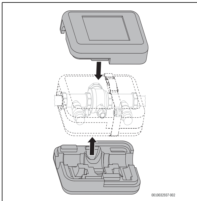
Rys. 56 Izolacja urządzenia napełniającego
