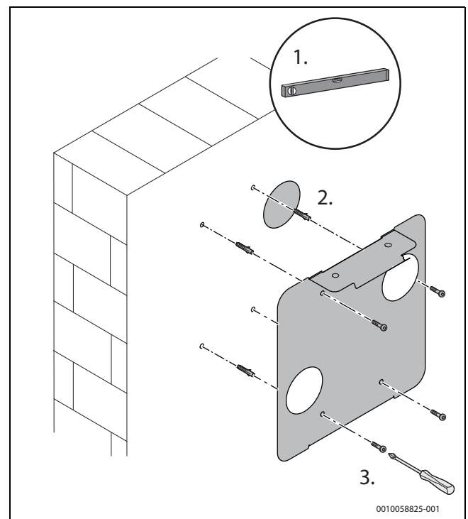
Rys. 34 Zamocować uchwyt
