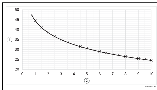
Rys. 29 Poziom ciśnienia akustycznego w trybie ciągłym w przeliczeniu na energię ( L_p(r, Q=4) ) dla wylotu szachtu wentylatora wentylacji awaryjnej umieszczonego na zewnątrz, w funkcji odległości od wylotu szachtu do punktu emisji (miejsca oceny). Całkowity czas oceny wynosi 8 godzin, a wykres przedstawia średni poziom ciśnienia akustycznego w całym okresie oceny
