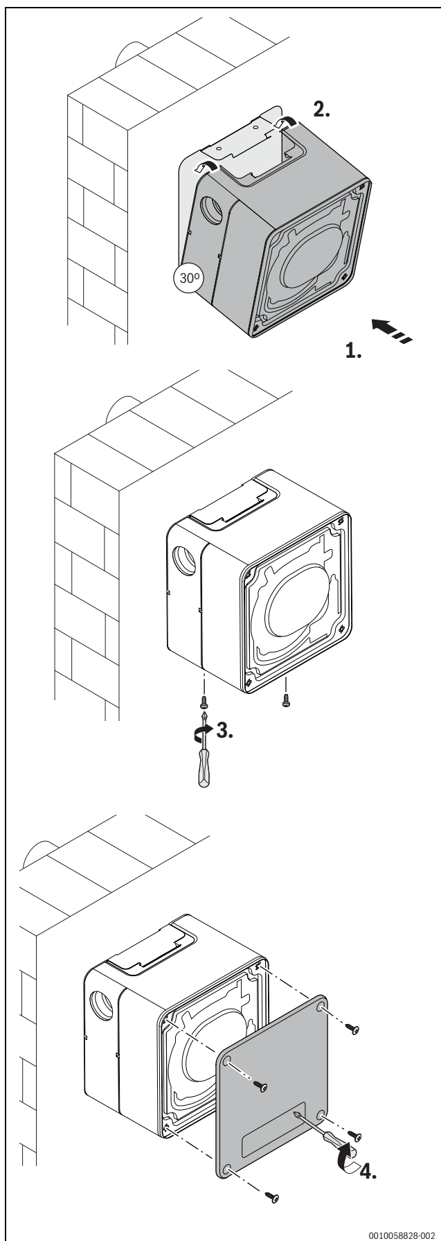
Rys. 43 Jak zamknąć obudowę wentylatora
