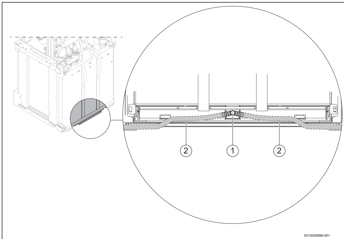
Rys. 45 Podłączyć wąż odpływowy
