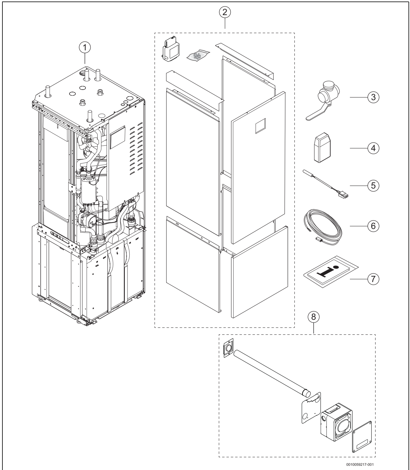
Rys. 1 Zakres dostawy
