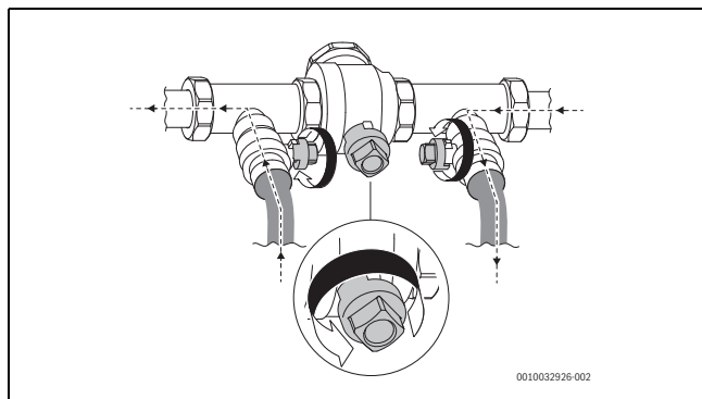
Rys. 51 Urządzenie napełniające w pozycji napełniania
