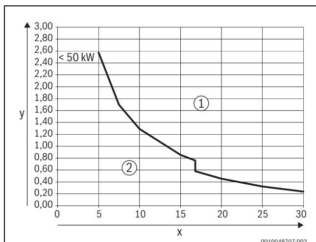
Rys. 9 Urządzenia grzewcze < 50–100 kW
