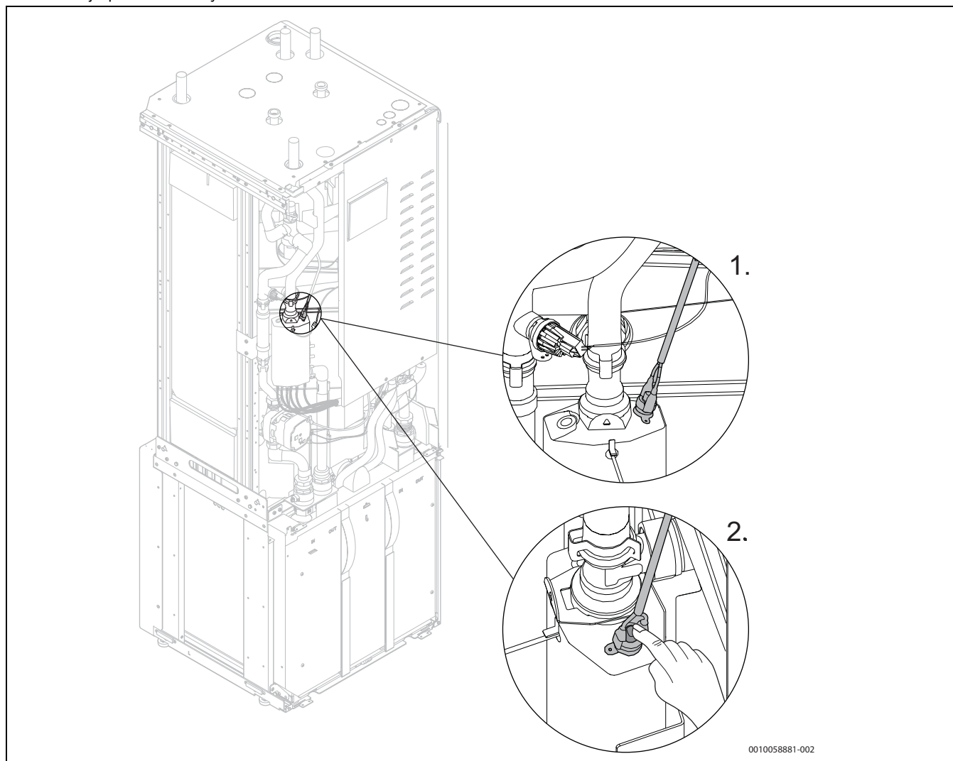
Obr. 69 Reset ochrany proti přehřátí
