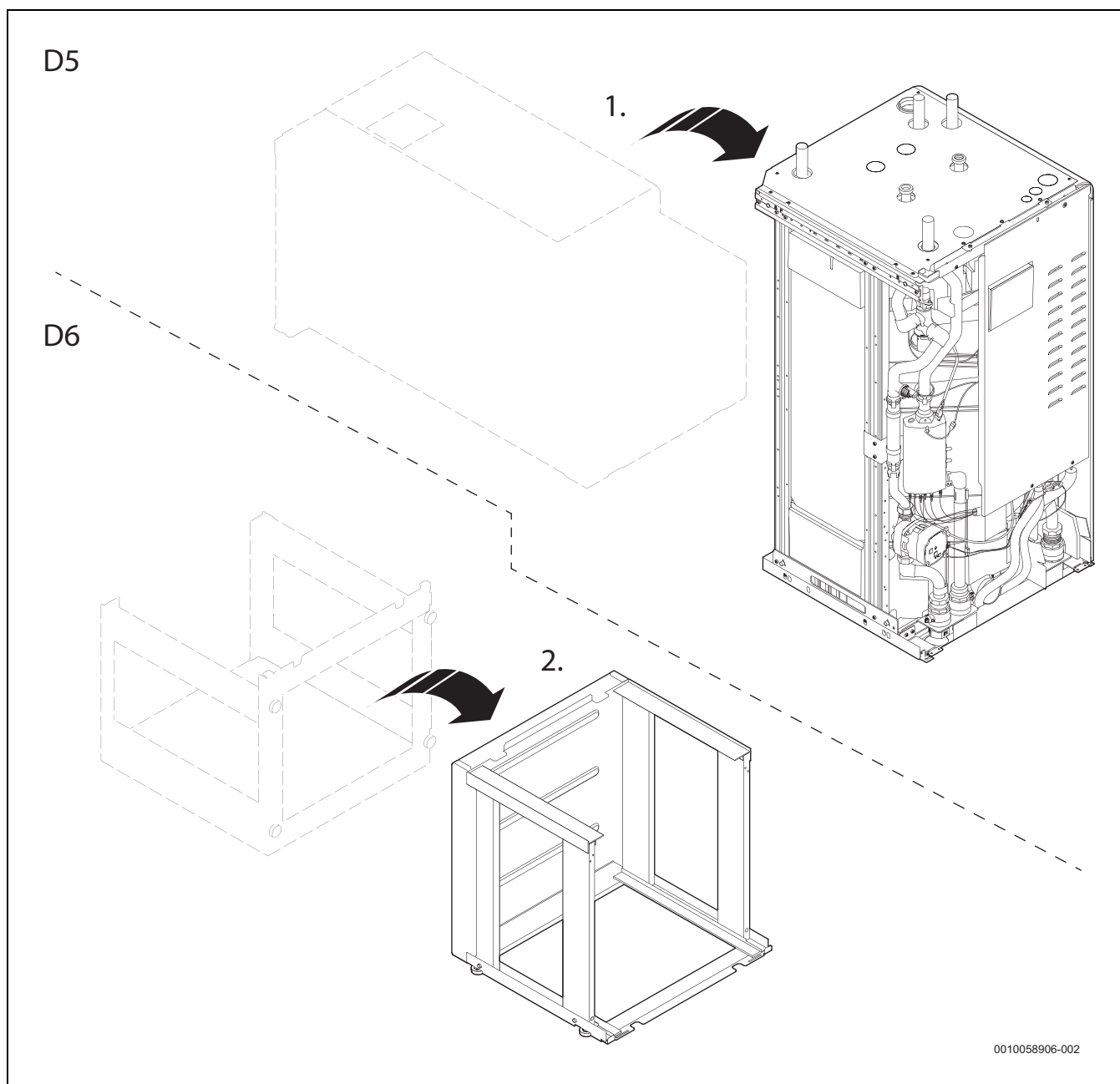
Obr. 16 Rozdělení tepelného čerpadla
