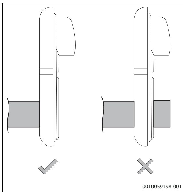
Obr. 40 Kanál nevkládějte příliš hluboko do skříně ventilátoru
