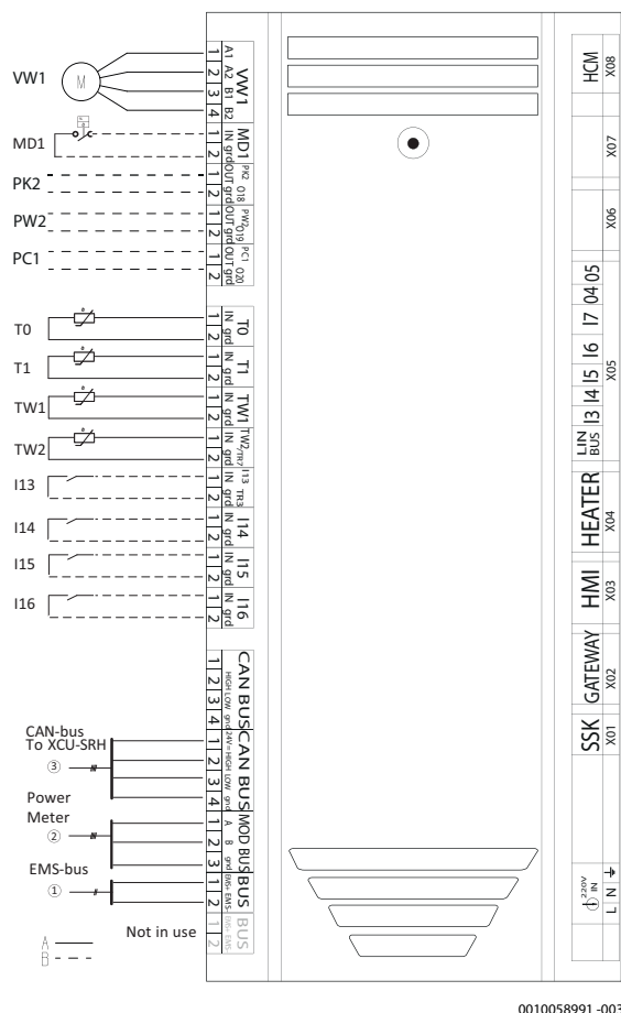
Obr. 62 Přípojky XCU-THH (XCU HY)
