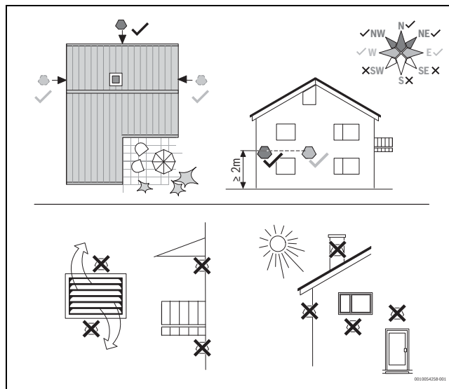
Obr. 64 Poloha čidla venkovní teploty
