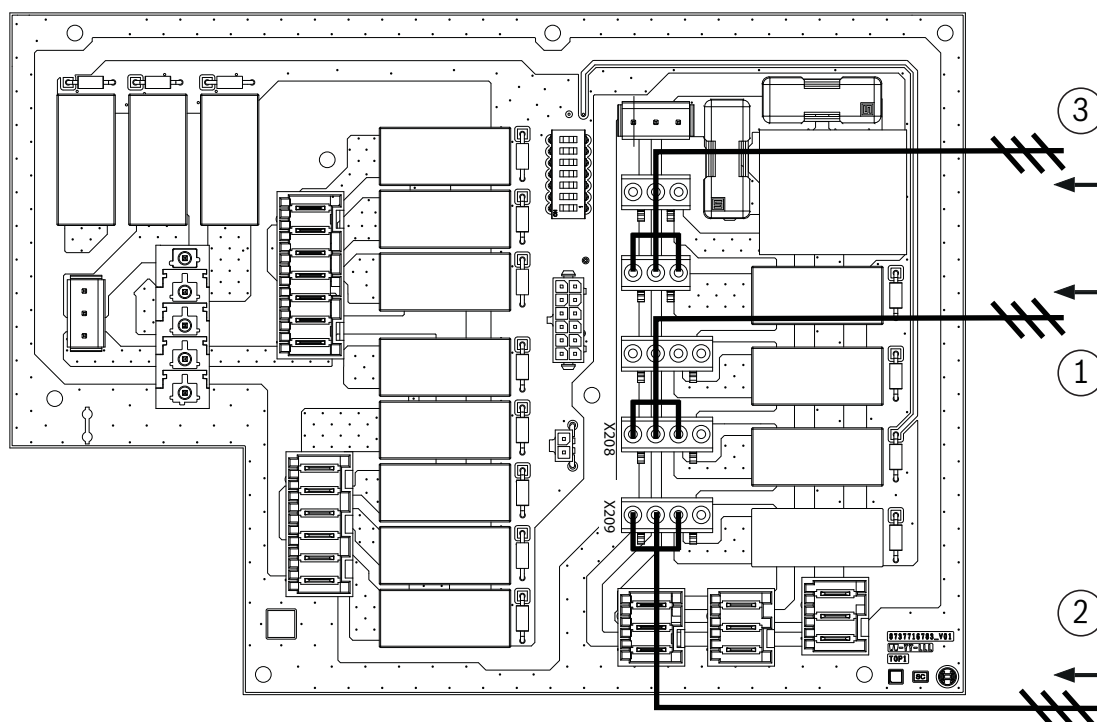
Obr. 61 Elektrické připojení příslušenství
