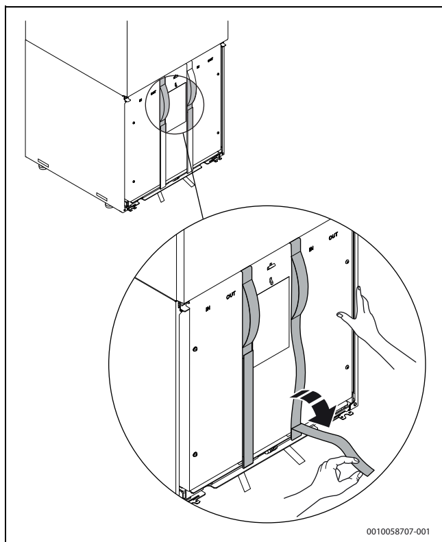
Obr. 17 Uvolněte pásky
