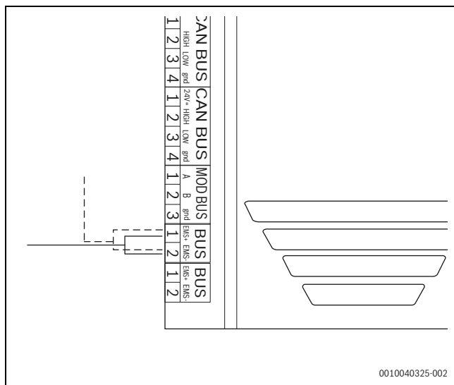
Obr. 65 Připojení EMS
