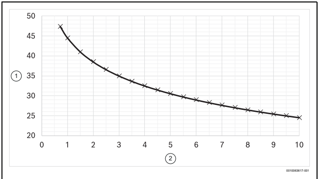
Obr. 29 Úroveň nepřetržitého akustického tlaku vyjádřená jako energetický ekvivalent (Lr(r, Q=4)) pro výstup potrubí evakuačního ventilátoru umístěného venku, v závislosti na vzdálenosti od výstupu potrubí k místu imise (místu posuzování). Celková doba měření činí 8 hodin a graf
