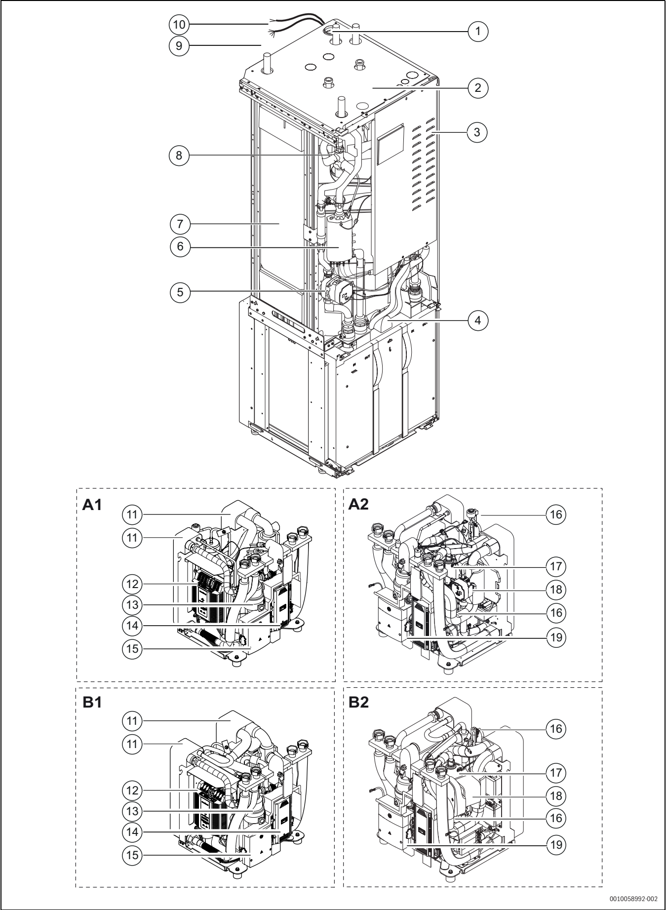
Obr. 4 Přehled výrobku
