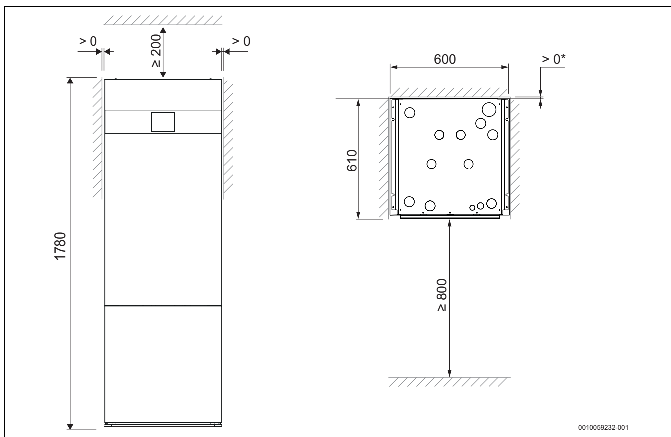
Obr. 2 Rozměry a minimální vzdálenosti
