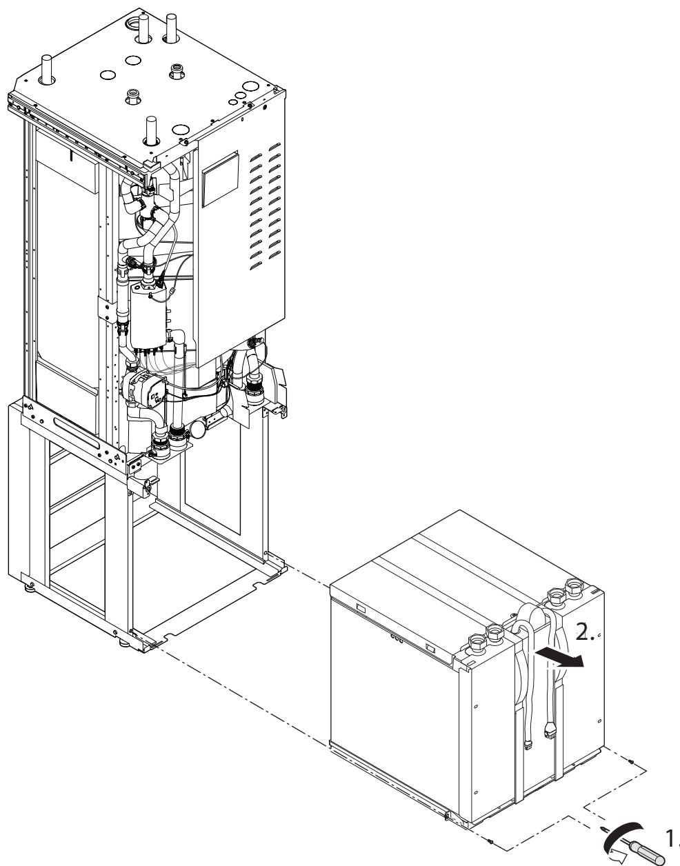
Obr. 14 Rozdělení tepelného čerpadla
